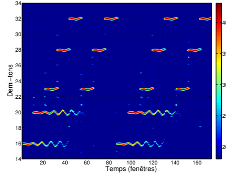
(b) Représentation des activations incluant les fréquences fondamentales (deux premières mesures de l'extrait). L'échelle de couleur est en dB.
