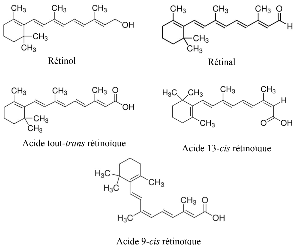
Figure 10 : Formule chimique des rétinoïdes naturelles
