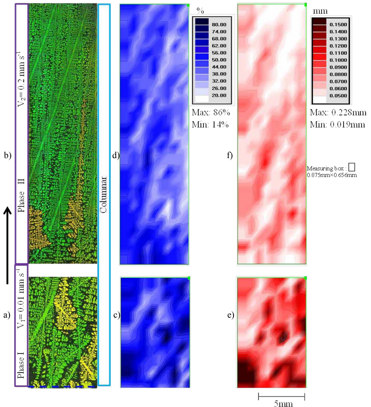
Chapitre 3 Fig. 1: Al-Si 7,0 %pds non affiné solidifié en microgravité, G_{\text{initial}} de 10\text{ K/cm} , V = 10\text{ }\mu\text{m/s} à 200\text{ }\mu\text{m/s} , Phase II : vitesse de refroidissement sur la zone chaude du four: 4\text{ K/min} simultanément à l'application de la vitesse de 200\text{ }\mu\text{m/s} . a) et b) Coupes longitudinales après polissage électrolytique, c) et d) Distribution du pourcentage d'eutectique (maximum 86 % et minimum 14 %), e) et f) Distribution de l'espacement dendritique, DAS (maximum 228\text{ }\mu\text{m} et minimum 19\text{ }\mu\text{m} ). La flèche noire indique le sens de solidification. Taille de la boîte pour la mesure du pourcentage d'eutectique et de l'espacement dendritique: 0.875\text{ mm} \times 0.656\text{ mm} .
