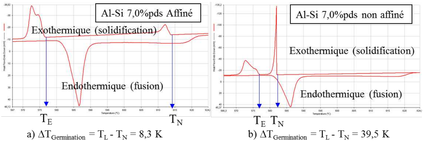
Chapitre 2 Fig. 11: Mesures par DSC pour l'alliage Al-Si 7,0 %pds. Protocole : Chauffé à 10 K/min jusqu'à 700 °C, Maintien à 700 °C pendant 1 h, Refroidissement à 5 K/min. a) Affiné, b) Non affiné. T_L est la température liquidus, T_N est la température de germination de la phase primaire.
