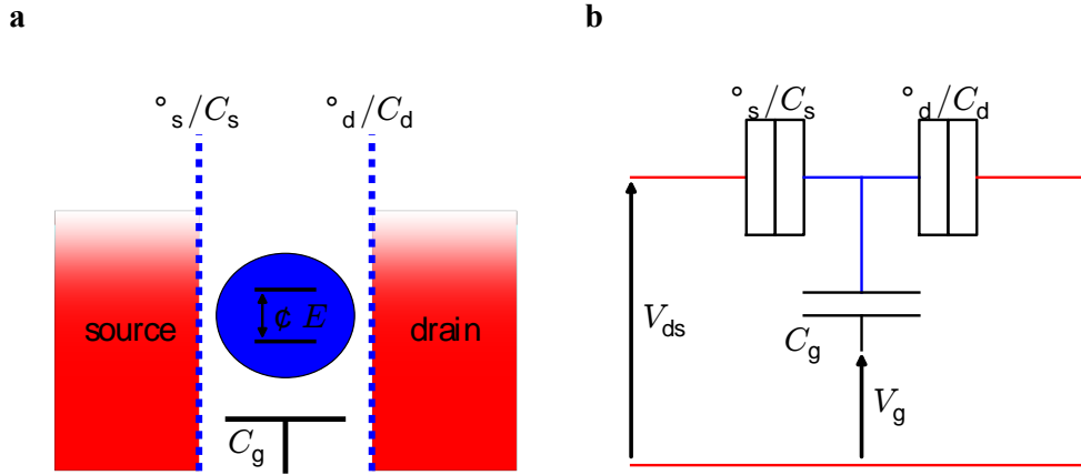
FIGURE A.1 – a : schémas d'un transistor à électron unique. b : schémas électrique équivalent.
