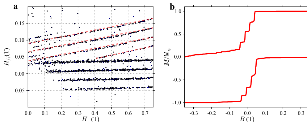
FIGURE Concl.2 – a : étude de la position des transitions induites en fonction du champ transverse et du champ parallèle. Chaque point marque un retournement de l'aimantation. Les transitions surlignées en rose correspondent à des renversements de l'aimantation induits par le couplage de l'aimant moléculaire avec un second système magnétique. b : reconstruction du cycle d'hystérésis obtenu en régime Kondo. Seules les transitions correspondantes au phénomène de QTM sont visible.
