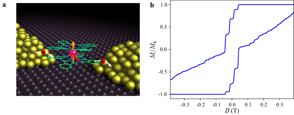
FIGURE Concl.1 – a : vue d’artiste de notre transistor moléculaire. b : reconstitution du cycle d’hystérésis de la molécule TbPc 2 pour un champ transverse de 750\text{ mT} .
