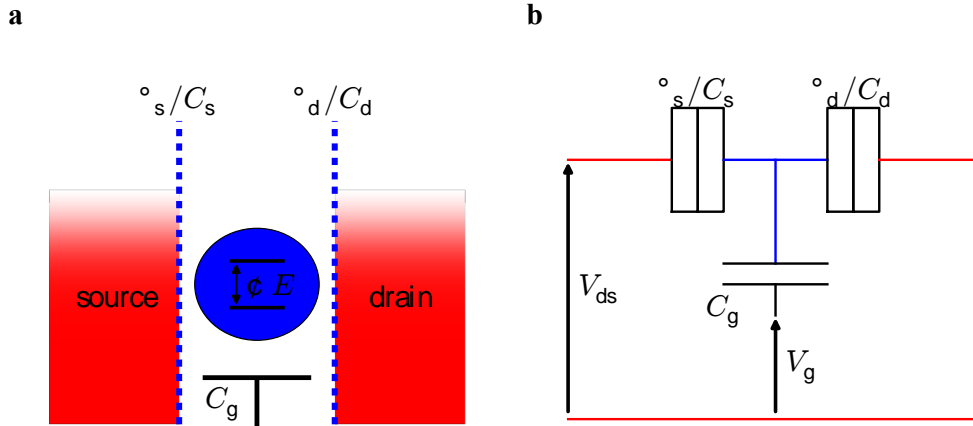
FIGURE A.1 – a : schémas d'un transistor à électron unique. b : schémas électrique équivalent.
