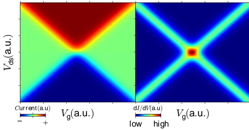
FIGURE B.1 – Courant correspondant à un état de charge (0,1) dans le plan (V_g, V_{ds}) sans champ magnétique
