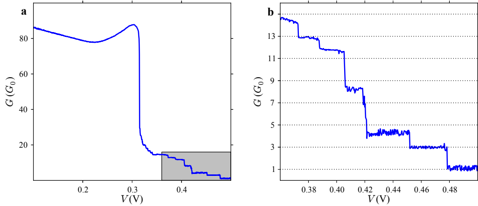
FIGURE 2.10 – a : conductance de la jonction durant l'électromigration. b : grossissement de la partie grisée de a montrant les marches de conductance témoignant du bon déroulement de l'électromigration.
