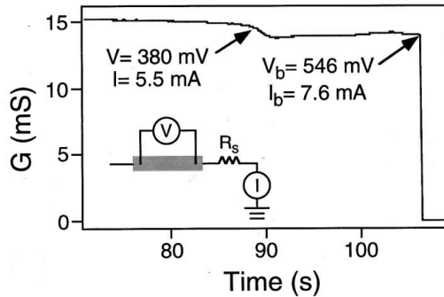
FIGURE 2.7 – Evolution de la conductance d'un nanofil au court du temps lors d'une procédure d'électromigration à rampe unique. Extrait de [51].
