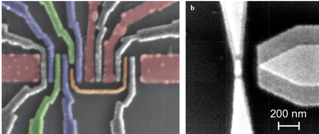
FIGURE 2.2 – Images obtenues par microscopie électronique à balayage. a : nanotube sur lequel on est venu positionner 9 grilles afin de réaliser un double point quantique ainsi qu'un détecteur de charge (extrait de [63]). b : configuration en grille latérale réalisée dans le cadre de jonctions électromigrées (extrait de [62]).
