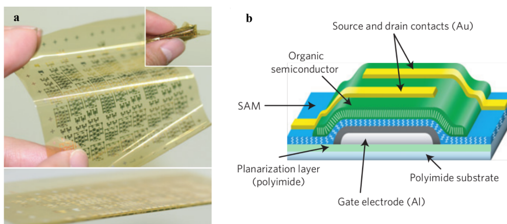
FIGURE 1.2 – a : Photographie d'un substrat de polyimide contenant des transistors organiques. b : Vue en coupe d'un transistor organique (figure extraite de [25]).
