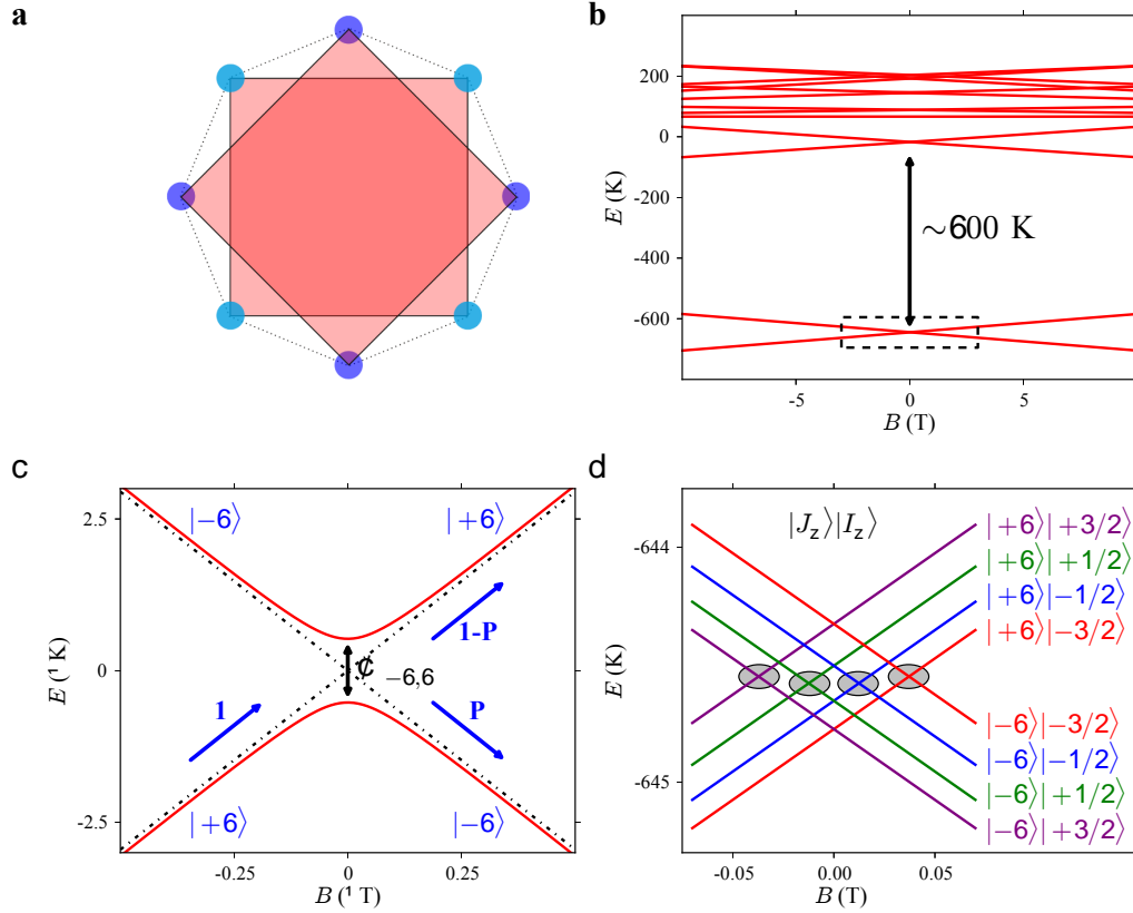
FIGURE 3.2 – a : schémas représentant la coordination anti-prisme. Les atomes d'azote sont représentés en bleu clair et bleu foncé, chaque couleur correspondant à un plan de ligand. b : diagramme Zeeman de la molécule TbPc_2 représentant l'énergie des différents états du système en fonction du champ magnétique. Les états fondamentaux J_z \pm 6 sont séparés des premiers états excités par une énergie de 600 K. c : agrandissement du diagramme Zeeman des deux états fondamentaux à faible champ magnétique. Il met en évidence un anti-croisement de valeur minimale \Delta_{-6,6} de l'ordre du \mu K qui traduit un mélange entre les états |+6\rangle et |-6\rangle . Si l'on balaie le champ magnétique des valeurs négatives vers les valeur positives, il existe une probabilité P de passer de l'état |+6\rangle à l'état |-6\rangle . Cette probabilité est régie par la formule de Landau-Zenner. d : Diagramme Zeeman lorsque l'on tient compte du couplage hyperfin entre le spin I = 3/2 du noyau et le moment magnétique électronique. Les deux doublets sont séparés en deux jeux de quatre sous-états. On ne relève que quatre anti-croisements marqués d'un cercle, où une transition de l'état |+6\rangle à l'état |-6\rangle est possible. (inspiré de [30] et [80]).
