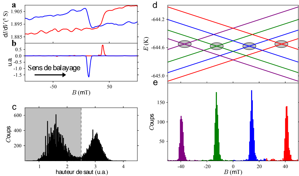
FIGURE 3.10 – a - Mesure de deux sauts de conductance montrant deux variations \Delta g de signes opposés. b - Signal correspondant à la mesure a filtrée : les sauts de conductance sont transformés en pics dont l'orientation (vers le haut ou vers le bas) dépend du signe de \Delta g . c - Statistique de la hauteur des sauts : cette dernière met en évidence deux distributions : celle contenue dans la zone grise correspond à de petites transitions relatives au bruit de mesure ; la seconde distribution correspond au signal induit par le retournement de l'aimantation. d - Diagramme Zeeman de l'état fondamental de la molécule de TbPc 2 à faible champ : les anti-croisements donnant lieu au phénomène de QTM sont repérés par les cercles grisés. e - Statistique portant sur la position en champ des retournements de l'aimantation : quatre résonances sont clairement identifiables et correspondent aux quatre anti-croisements.
