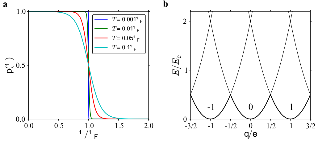
FIGURE A.2 – a : probabilité d’avoir un électron de potentiel chimique \mu sachant que le potentiel chimique du métal est \mu_F , pour différentes températures. b : évolution de l’énergie des états de charges -1 , 0 et 1 en fonction de q = -C_g V_g . Pour des valeurs demi-entières de q/e , deux états de charge se retrouvent dégénérés. On parle de point de dégénérescence (inspiré de [103]).
