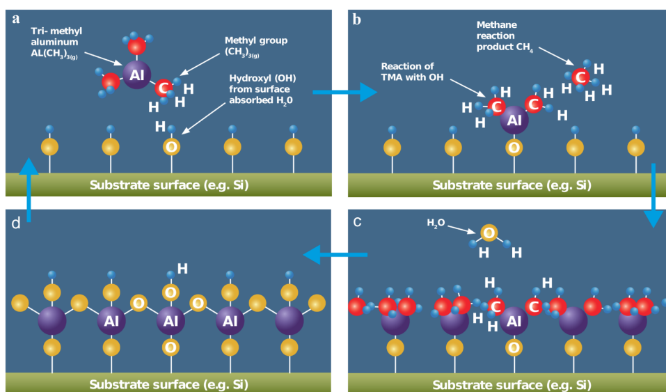
FIGURE 2.4 – Première étape du cycle ALD : le premier précurseur, ici du \text{Al}(\text{CH}_3)_3(g) , se fixe à la surface (a) et les produits issues la réaction de fixation sont évacués par un flux de gaz inerte (b). Dans un deuxième temps, de l'eau est injectée et réagit avec la première couche de précurseur (c) pour former une couche atomique d'oxyde (d). Le cycle se répète ensuite à raison d'une couche atomique par cycle. (extrait du site CambridgeNanoTech)
