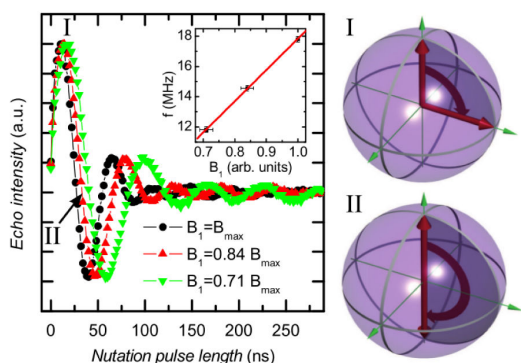
FIGURE Concl.4 – (lignes de couleur) Oscillations de Rabi obtenues en enregistrant l'intensité de l'écho en fonction de la durée de pulsation sur du \text{Fe}_4 à très basse température et pour différents champs magnétiques. Pour deux positions dans le cycle de Rabi, la position correspondante est présentée dans la partie droite (extrait de [14]).
