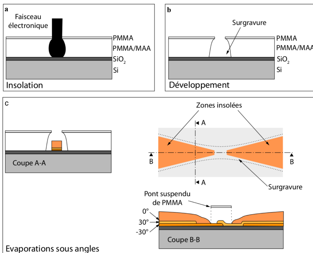
FIGURE 2.6 – a : Insolation par lithographie électronique de la bicouche de résine. La partie la plus proche du substrat (PMMA/MAA) se trouve plus insolée de par une plus grande sensibilité aux électrons et la présence des électrons rétrodiffusés. b : résultats après développement montrant clairement la surgravure générée par la surexposition de la partie basse. c : Evaporation sous angles : différentes couleurs représentent les différents angles d'évaporation ( -30^\circ , 0^\circ et 30^\circ - extrait de [?]).
