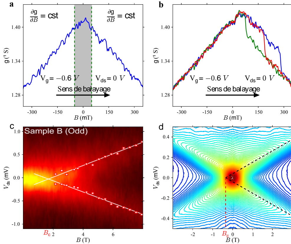
FIGURE 3.9 – a - Mesure de la conductance différentielle en fonction du champ magnétique en l'absence de saut de conductance : les zones non grisées correspondent à des valeurs de champ magnétique où la variation de potentiel chimique \Delta\mu est directement proportionnelle à la variation en conductance \Delta g . b - Mesure de trois sauts de conductance pour différentes valeurs de champ magnétique : celle-ci met en évidence l'indépendance de la variation \Delta g vis-à-vis du champ magnétique appliqué. c(d) : Mesure en conductance différentielle de l'effet Kondo 1/2 en fonction du champ magnétique et de la tension source-drain pour un système sans (soumis à l') interaction d'échange. L'extrapolation des maxima de conductance permet d'extraire la séparation Zeeman ainsi que la valeur du champ critique B_c .
