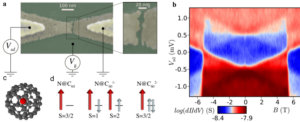
FIGURE 1.8 – a : image obtenue par microscopie électronique à balayage illustrant la géométrie d'un transistor moléculaire obtenu par électromigration. b : spectroscopie en cotunneling obtenue en mesurant la conductance différentielle de l'échantillon en fonction de la tension source-drain V_{ds} et du champ magnétique B pour une tension de grille V_g fixée. c : vue d'artiste de la molécule de N@C_{60} . d : configuration magnétique de cette dernière en fonction de son état de charge (extrait de [49]).
