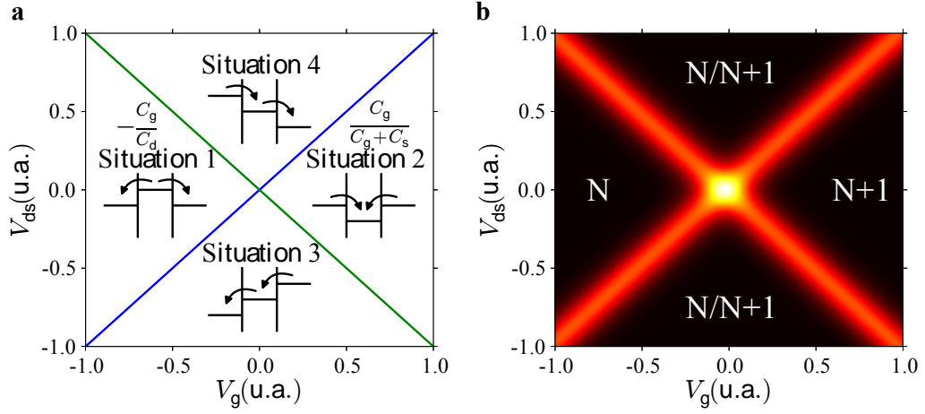
FIGURE A.3 – a : représentation de la charge et de la décharge de l'îlot dans le plan (V_g, V_{ds}) . Le régime de blocage de Coulomb est représenté par les situations 1 et 2. Un courant est mesuré dans les situations 3 et 4. b : même diagramme obtenu en mesurant la conductance différentielle dI/dV en fonction des tensions V_g et V_{ds} . La valeur de la conductance différentielle est basse pour les zones sombres et élevée pour les zones claires.
