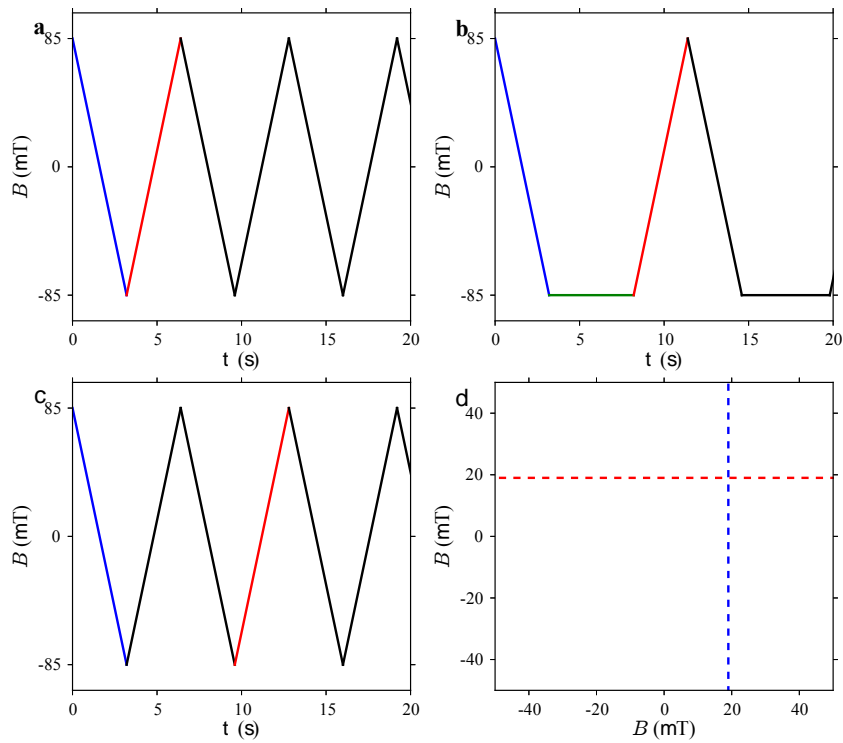
FIGURE 3.16 – a (b) : représentation de la procédure de mesure lorsqu’aucun temps d’attente (un temps d’attente de 5 secondes, représenté en vert) n’est inséré entre la retrace et la trace suivante. c : procédure de mesure correspondant à une corrélation du troisième ordre, deux mesures se situant entre les deux retournement considérés (en bleu et en rouge). d : représentation d’une corrélation dans un diagramme à deux dimensions. La position en champ magnétique du retournement de l’aimantation obtenue durant les deux mesures est repérée sur les axes x , et y par deux lignes dont le croisement va donner un point de corrélation. En répétant cette procédure un grand nombre de fois, un histogramme en deux dimensions de ces corrélations peut être obtenu (cf Fig.3.17).
