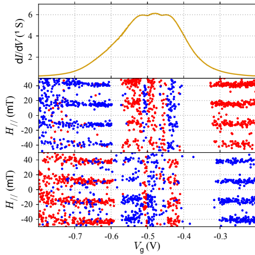
FIGURE 3.12 – Panel haut - Mesure de la conductance différentielle en fonction de la tension de grille V_g à tension source-drain nulle. Panel du milieu (bas) - Mesure du signe de \Delta g en fonction de la tension de grille V_g et du champ transverse H_{//} durant la trace (retrace) : les points rouges correspondent à \Delta g > 0 ; les points bleus à \Delta g < 0 . Les zones blanches dénotent des valeurs de tension de grille pour lesquelles le signal magnétique n'est pas résolu.
