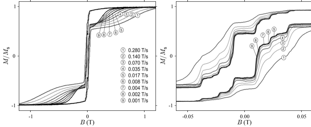
FIGURE 3.3 – a : Mesure de l'aimantation d'un cristal de TbPc_2 dilués à 10 % pour différentes vitesses de balayage. b : grossissement de la partie centrale mettant en évidence l'influence de la vitesse de balayage sur la hauteur des marches associées au retournement par QTM.(extrait de [30]).
