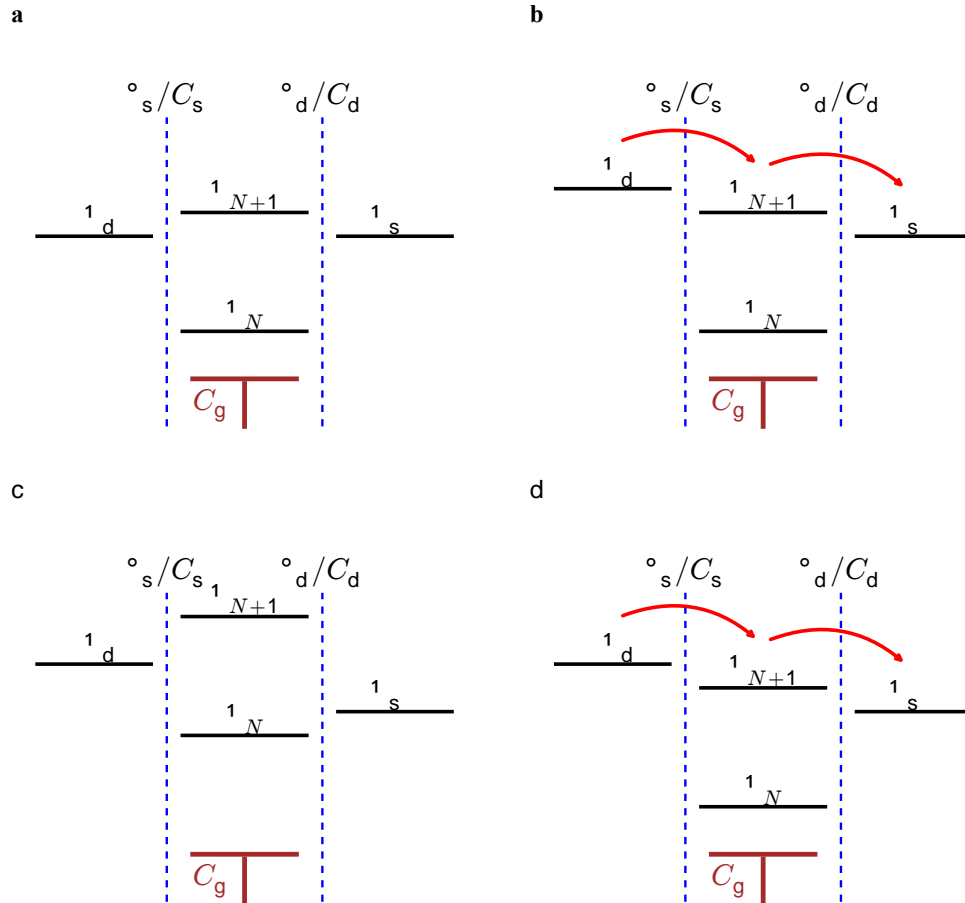
FIGURE 3.5 – Représentation schématique d'un point quantique. a : Lorsque les potentiels chimique de la source et du drain ( \mu_s et \mu_d ) ne sont pas alignés avec ceux du point quantique, aucun courant ne circule, et l'état de charge du point quantique est bien défini (ici N ). b : en appliquant une tension source drain, on ouvre une fenêtre de potentiel chimique. Si le potentiel chimique du point quantique se trouve dans cette fenêtre, un courant peut circuler. De plus, en appliquant une tension sur l'électrode de grille, on peut amener un potentiel chimique du point quantique, initialement en dehors de la fenêtre ( c ), à l'intérieur de celle-ci ( d ), induisant un courant.
