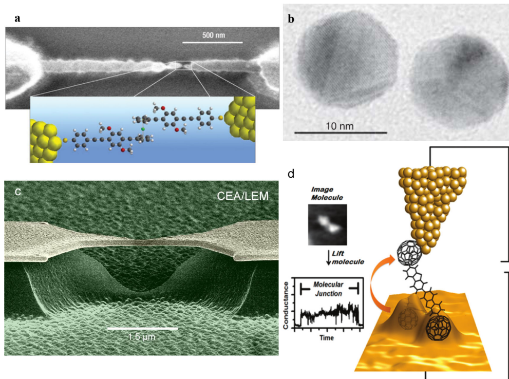
FIGURE 1.5 – a : image obtenue par microscopie électronique à balayage d'une jonction moléculaire obtenue par technique d'électromigration, ainsi que la vue d'artiste correspondante (extrait du site WEB de l'université de Tel Aviv). b : image par microscopie électronique à transmission (TEM) d'un dimer, à base de BDMT (1,4- benzenedimethanethiol), constitué par deux billes d'or de 10\text{ nm} . Le nanomètre qui sépare les deux billes correspond approximativement à la taille de la molécule de BDMT ( 0.9\text{ nm} ). (Figure extraite de [37]). c : image par microscopie électronique à balayage d'une jonction à cassure (image CEA/LEM). d : image d'artiste d'une mesure STM (extrait de [38]).
