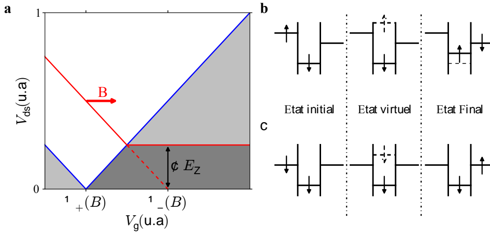
FIGURE A.5 – a : représentation du cotunneling dans le plan (V_g, V_{ds}) . Ce dernier est responsable de la présence de courant dans les zones de blocage. Ce courant peut varier au sein de cette zone comme le montre les deux niveaux de gris. b : représentation des trois temps du cotunneling inélastique. L'état final de l'îlot est de plus haute énergie que l'état initial. c : représentation des trois temps du cotunneling élastique. L'énergie de l'îlot entre l'état initial et l'état final est identique.
