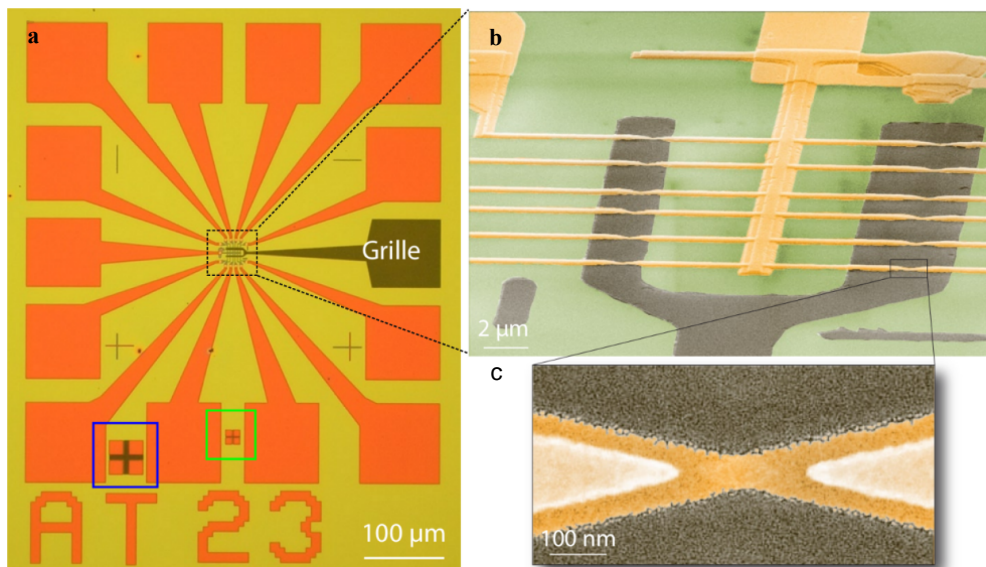
FIGURE 2.5 – a : Échantillon après les deux étapes de lithographie optique. Les lignes d'amené de courant sont visibles en orange et la grille locale en gris. Les deux carrés repèrent les marques d'alignement. b : Image obtenue par microscopie électronique à balayage montrant la structure centrale de nos échantillons. c : grossissement présentant une constriction obtenue à l'aide de l'évaporation sous angle. La grille, colorée en gris, est clairement visible au centre (extrait de [?]).
