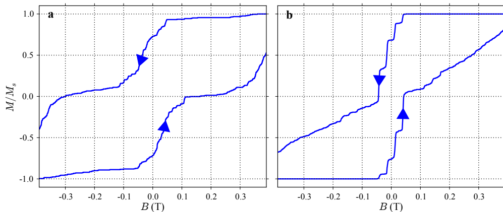
FIGURE 3.14 – Hysteresis de la molécule \text{TbPc}_2 reconstruit à partir des mesures en transports sans champ transverse (a), et avec un champ transverse de 750 \text{ mT} (b).
