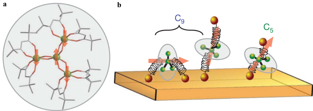
FIGURE 1.3 – a : Structure du cluster de Fe 4 . b : Représentation des différents modes d’ancrage, correspondant à différentes orientations de l’axe facile (extrait de [26]).
