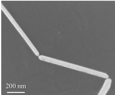
FIGURE Concl.3 – Configuration idéale, bien que très peu reproductible pour l'instant, de bâtonnets d'or joints bout-à-bout par une ou quelques molécules (extrait de [99]).
