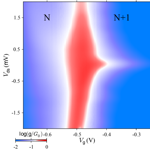
FIGURE 3.8 – Diagramme de Coulomb montrant la mesure en conductance différentielle de notre échantillon, en fonction de la tension de grille V_g et la tension source drain V_{ds} . L'état de charge passe de N à gauche du point de dégénérescence à N+1 à gauche de ce point.
