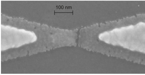
FIGURE 2.11 – Image obtenue par microscopie électronique à balayage d'une jonction électromigrée pour laquelle l'interstice nanométrique est clairement visible.
