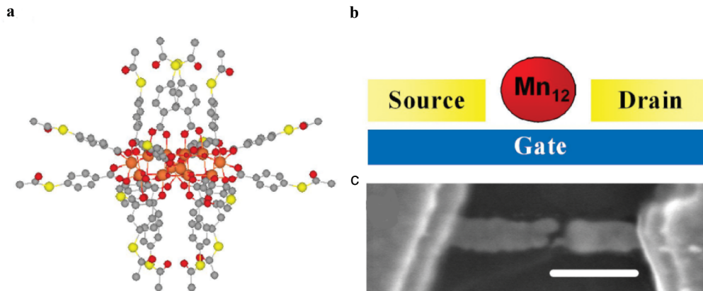
FIGURE 1.6 – a : structure du Mn_{12} entouré de ligands thiols favorisant l’ancrage. b : Représentation schématique de la molécule de Mn_{12} piégée entre les électrodes. c : image de la jonction électromigrée obtenue par microscopie électronique à balayage. Le trait blanc correspond à 200\text{ nm} . (extrait de [43]).
