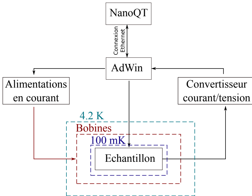
FIGURE C.1 – Diagramme de notre dispositif expérimental. L'automate AdWin est commandé à l'aide du logiciel NanoQt à travers la rédaction de scripts. Cet automate prend en charge les commandes relatives aux bobines, à la polarisation de l'échantillon ainsi qu'à l'acquisition des données qui sont renvoyées vers l'ordinateur pour traitement. Un réfrigérateur à dilution permet de refroidir l'échantillon à une température électronique de 100\text{ mK} . Les bobines, immergées dans l'hélium liquide, sont à une température de 4.2\text{ K} .
