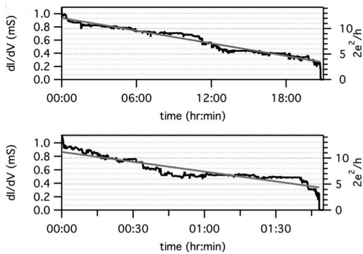
FIGURE 2.9 – Évolution de la conductance de deux nanofils au cours du temps lors d'une procédure d'électromigration à cassure spontanée. Extrait de [77].
