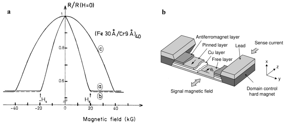
FIGURE 1.1 – a : mesure de la résistance d'une vanne de spin mettant en évidence la magnéto-résistance géante (extrait de [18]). b : Schéma d'une tête de lecture de disque dur, dont le fonctionnement est basé sur le phénomène de magnéto-résistance (extrait de [20]).
