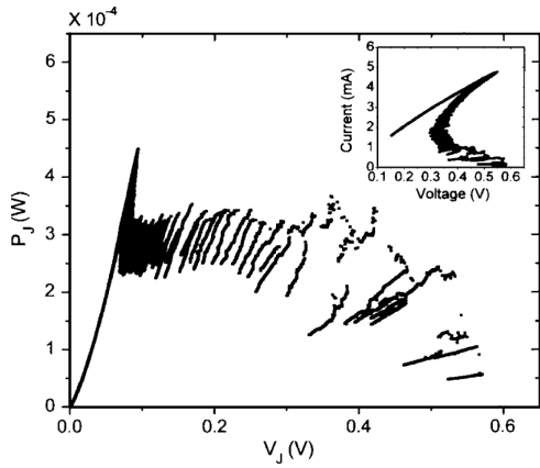
FIGURE 2.8 – Evolution de la puissance dissipée en fonction de la tension appliquée, lors d'une procédure d'électromigration à contre-réaction. En encart, caractéristique courant-tension lors de cette même procédure. Extrait de [76].
