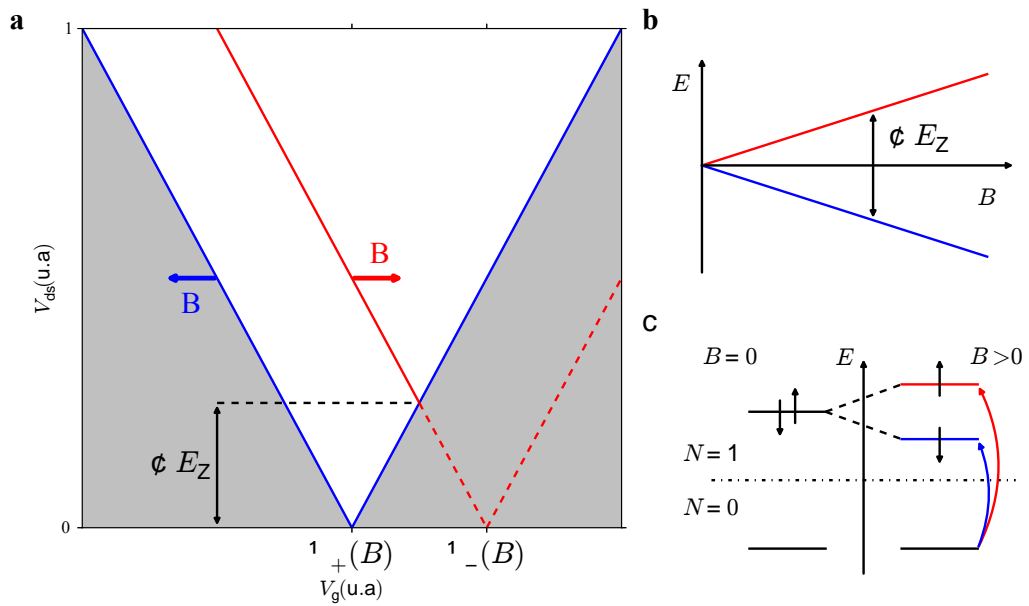
FIGURE A.4 – a : diagramme de stabilité tenant compte des états fondamentaux et excités. L'influence du champ magnétique est directement mesurable au niveau des croisements des bords de diamant qui nous donnent une lecture directe de l'énergie de Zeeman \Delta E_z . b : diagramme Zeeman de l'état de charge N=1 . L'application d'un champ magnétique lève la dégénérescence entre les deux spins de l'énergie Zeeman \Delta E_z . c : potentiel chimique correspondant à la transition 0/1. L'influence du champ magnétique vient lever la dégénérescence des deux états de spin et donc des deux potentiels chimiques correspondants.
