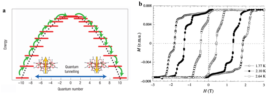
FIGURE 1.4 – a : échelle des énergies des différents états de spin pour un spin S = 10 . Le renversement peut s’effectuer par effet tunnel (QTM - Quantum Tunneling of the Magnetization) lorsqu’un des niveaux dans le premier puits est en résonance avec un niveau dans le second (flèche bleue). L’aimantation peut également “monter” l’échelle des énergies par l’absorption de phonons, pour ensuite redescendre dans le second puits en émettant des phonons (flèche verte) (extrait de [10]). b : Première mesure du phénomène de QTM sur un cristal moléculaire de Mn_{12}Ac , mettant en évidence la structure en marche associée au retournement par effet tunnel (extrait de [28]).
