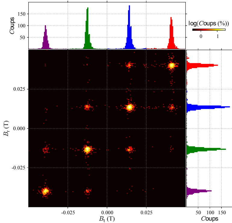
FIGURE 3.17 – La cartographie couleur en deux dimensions représente l’histogramme de corrélation des champs de retournement ayant lieu durant la trace et la retrace. Celui-ci a été obtenu à partir de 22000 traces et retraces mesurées consécutivement, et sans temps d’attente. Les histogrammes à une dimension disposés le long des axes x et y représentent respectivement la statistique des positions en champ magnétique des retournements durant la trace et la retrace. La prépondérance des éléments diagonaux atteste de la préservation de l’état de spin entre deux mesures.
