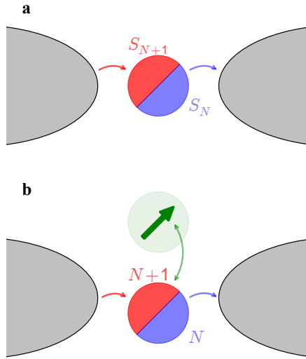
FIGURE 3.6 – a : configuration directe. Le centre magnétique est directement impliqué dans le transport électronique. Il oscille entre les états de charges N et N + 1 . Cette oscillation entraîne une alternance entre les états magnétiques S_N et S_{N+1} . b : configuration indirecte. Le centre magnétique n'est pas directement couplé au transport électronique mais par l'intermédiaire d'un point quantique. Cette dernière oscille entre deux états de charge N et N + 1 , ces derniers étant influencé par l'état magnétique du centre magnétique, du fait d'une interaction (échange, dipolaire etc.).
