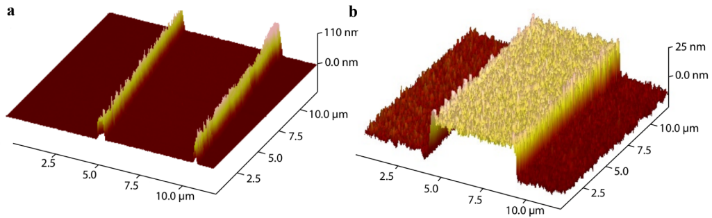
FIGURE 2.3 – a : image AFM d'une électrode de grille présentant des bords trop relevés dû fait d'un problème de lift-off, obtenue par une technique monocouche. b : image AFM montrant une électrode de grille après lift-off ne présentant pas d'anomalie après lift-off obtenue par la la technique bicouche (extrait de [54]).
