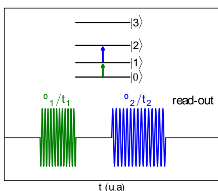
FIGURE Concl.5 – Schéma de la technique de pompe-sonde. Une première fréquence \nu_1 initialise l'état de |0\rangle à l'état |1\rangle . Puis un second pulse fait passer le système de l'état |1\rangle à l'état |2\rangle . On effectue ensuite la lecture de l'état par la méthode présentée au Chap.3.
