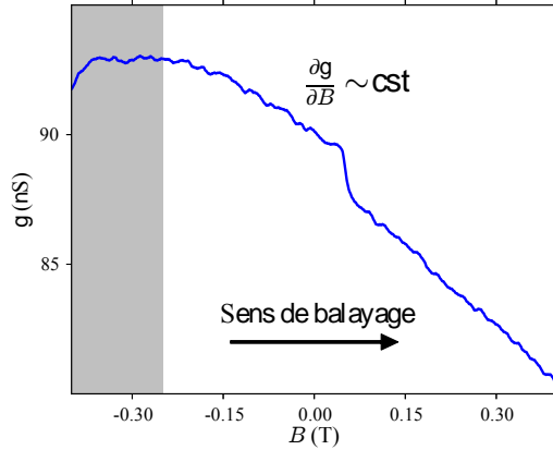
FIGURE 3.15 – Mesure de la conductance différentielle g pour un champ transverse 750 \text{ mT} . La zone correspondant à \frac{\partial g}{\partial B} \sim \text{cst} s'étend sur toute la zone de mesure.
