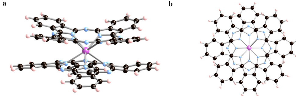
FIGURE 3.1 – Vue d’artiste de la molécule de terbium double-decker de côté (a) et de dessus (b). L’atome de terbium, ici en violet, est pris en sandwich entre deux phthalocyanines, ces derniers étant orientés à 45^\circ environ, l’un par rapport à l’autre. Les atomes d’azote et de carbone sont représentés respectivement en bleu et noir.
