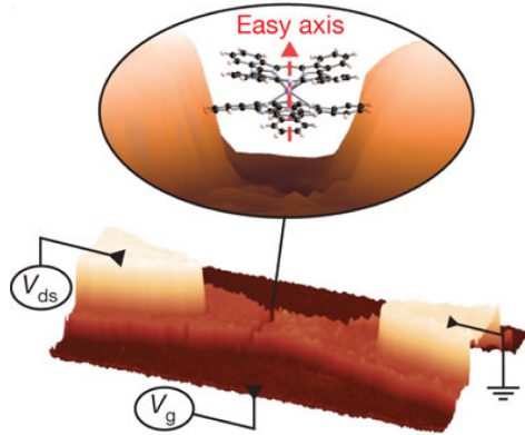
FIGURE 2.1 – Extrapolation 3D d’une image obtenue par microscopie électronique à balayage. Elle correspond à la structure finale que l’on souhaite obtenir : les électrodes de source et de drain, l’électrode de grille, ainsi qu’un interstice nanométrique dans lequel une molécule est piégée (extrait de [55]).
