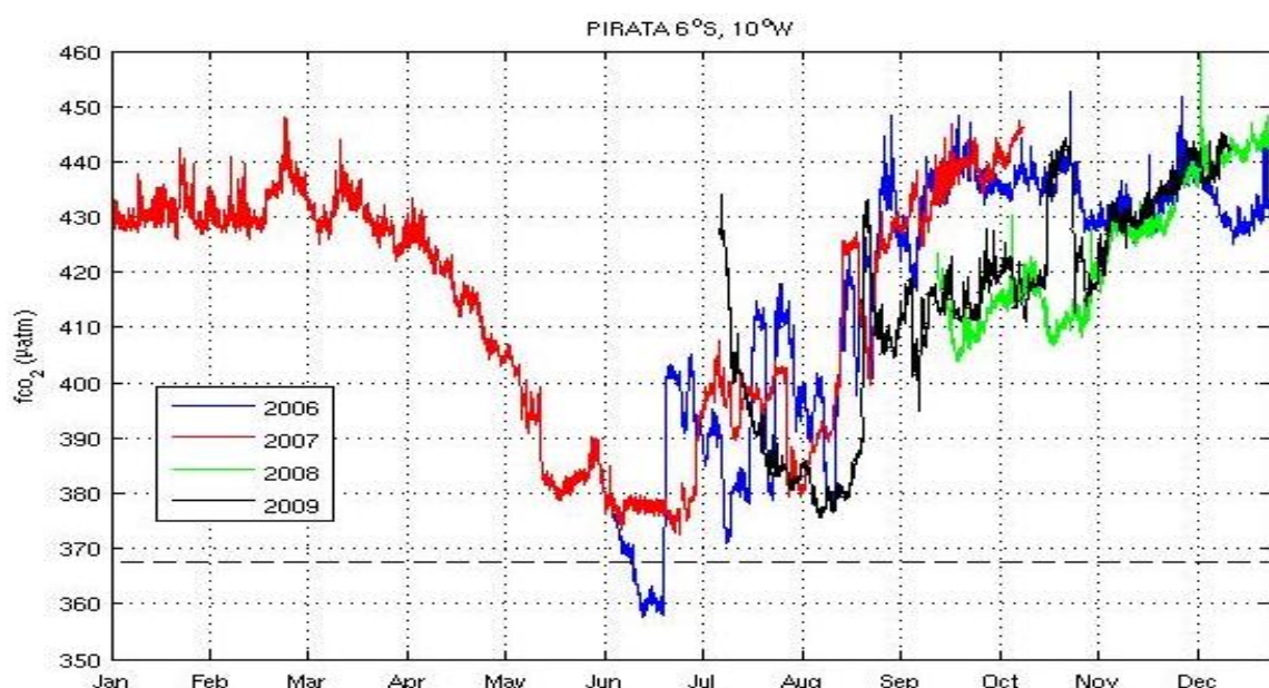
Figure 47 : Mesures en continu de la f\text{CO}_2 sur la bouée PIRATA (6°S, 10°W) en 2006, 2007, 2008 et 2009 (Parard et al, 2010).
