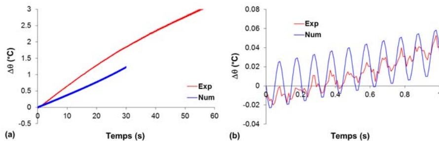
Figure 9.36. Evolution de la température simulée au cours de 300 cycles à droite en bas (a) au cours de 300 cycles, (b) 10 premiers cycles de l'essai de cisaillement à F_{\max} = 250\text{N} , f = 10\text{Hz} et R = -1 .
