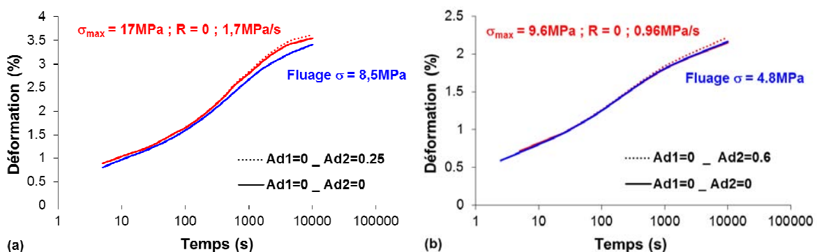
Figure 5.18. Rôle de la contrainte moyenne en distinguant l'état stabilisé en charge et en décharge : (a) en traction et (b) en cisaillement.
