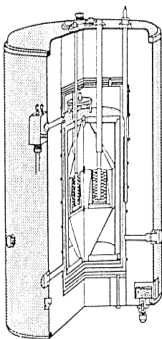
Fig. 3.1 Calvet microcalorimeter.
