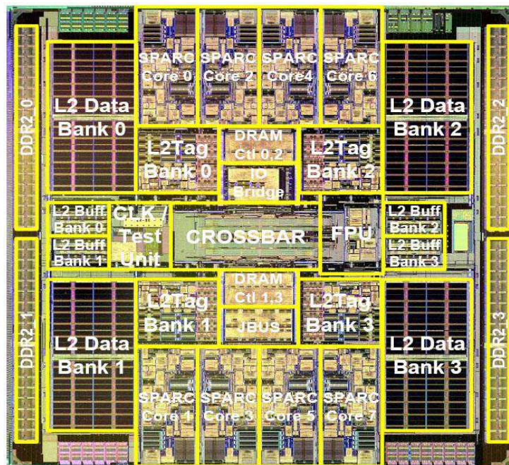
Figure 5.23 : Le floorplan de l'UltraSparc considéré
