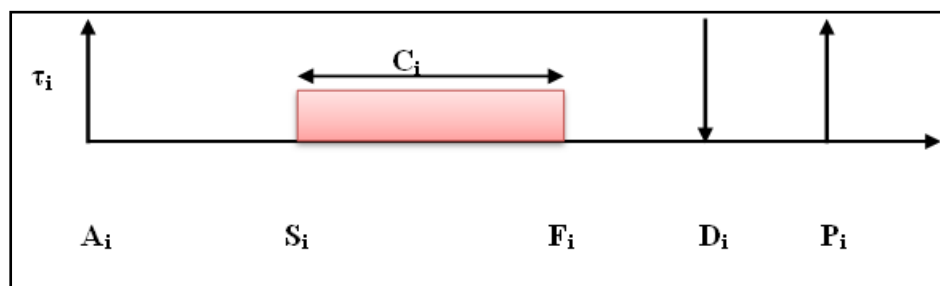
Figure 2.1 : Notations et caractéristiques de base d'une tâche
