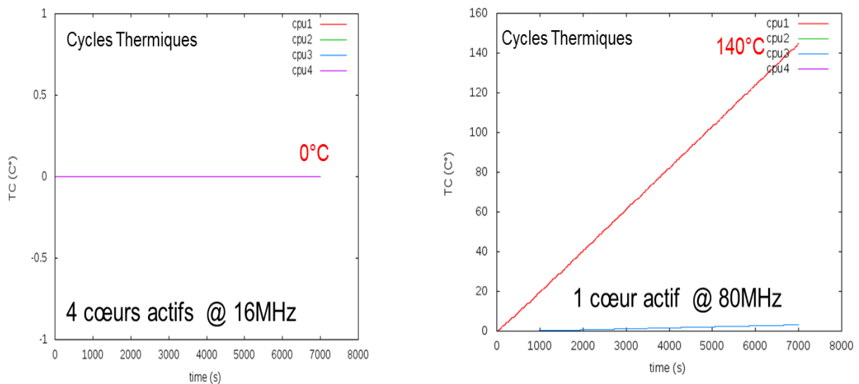
Figure 5.10 : Cycles thermiques cumulés par processeur
