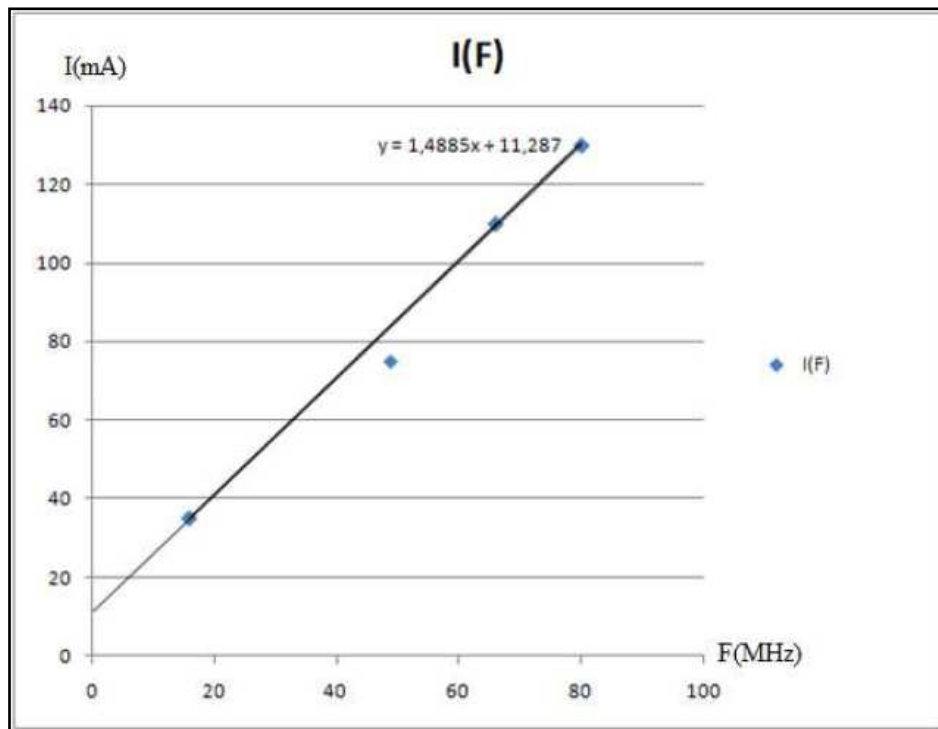
Figure 3.9 : Courbe de courant en fonction des fréquences à température ambiante 70°
