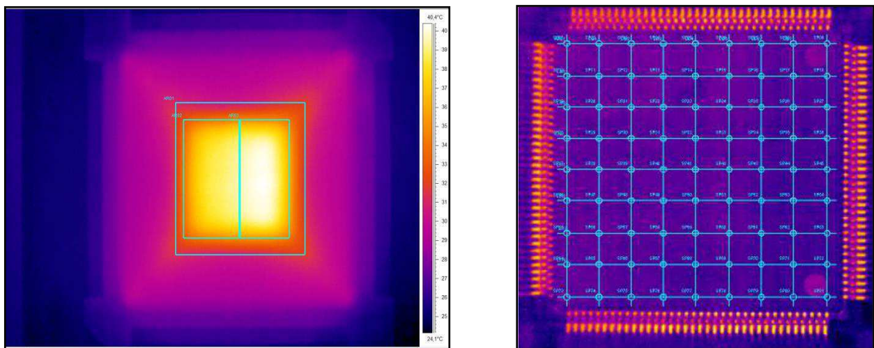
Figure 3.3 : Circuit encapsulé vu par la caméra thermique
