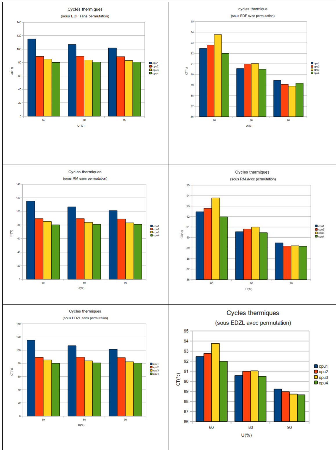
Figure 5.22 : Cycles thermiques subi par les différents cœurs et les 3 algorithmes globaux considérés, ainsi sous les différentes charges de processeurs.
