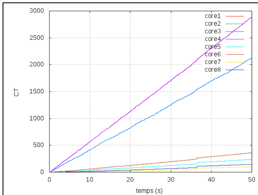
Figure 5.29 : Cycles thermiques correspondent à l'évolution en température de la Figure 5.26
