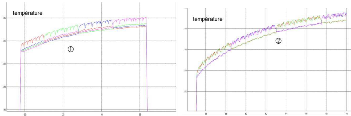
Figure 5.20 : Détail des variations en température des intervalles ① et ② de la
