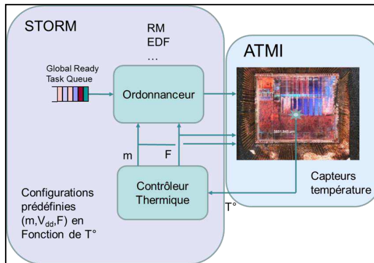
Figure 4.4 : Contrôleur thermique
