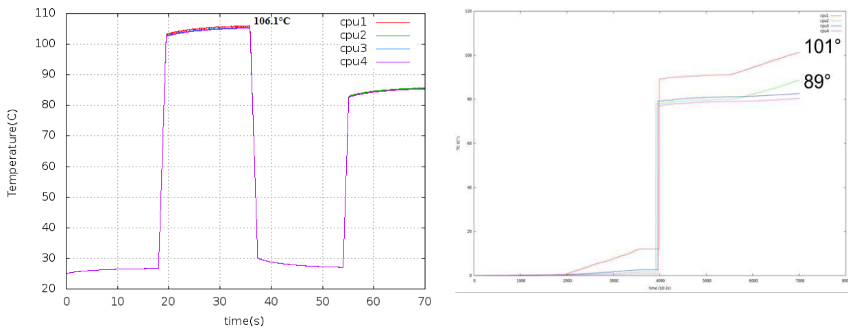
Figure 5.17 : Résultats avec EDZL et U=90%
