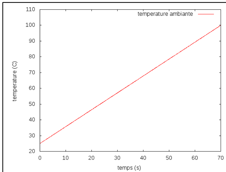
Figure 5.1 : Variation linéaire de la température ambiante en simulation
