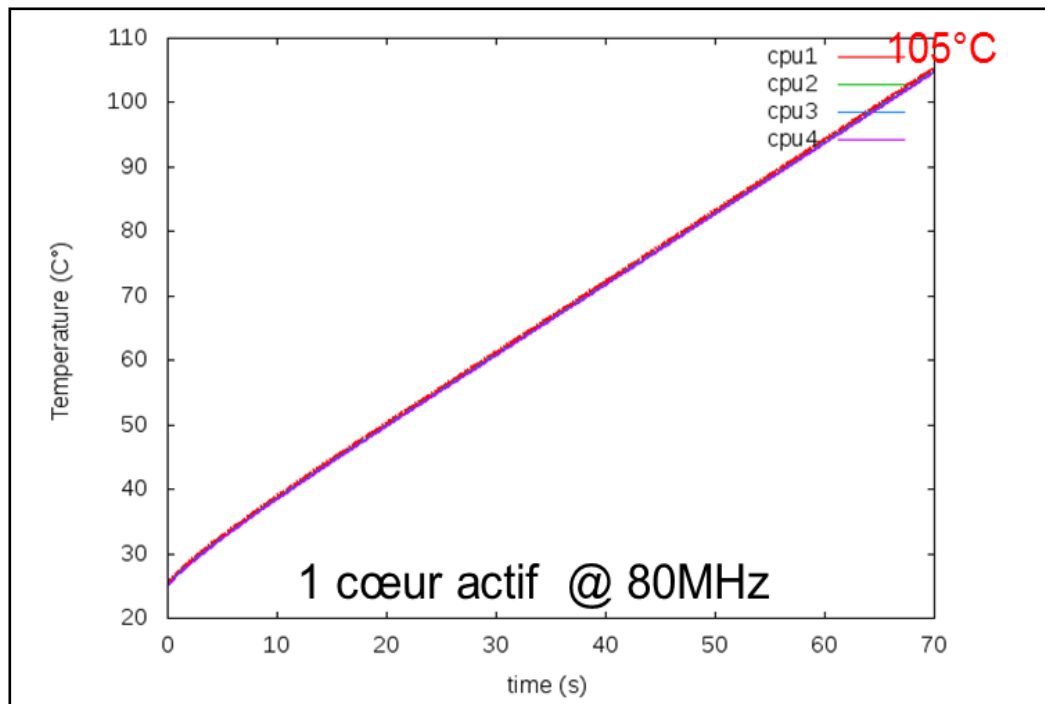
Figure 5.4 : Variation en température de l'architecture à 4 cœurs à 80 MHz (EDF) dont un seul est actif.
