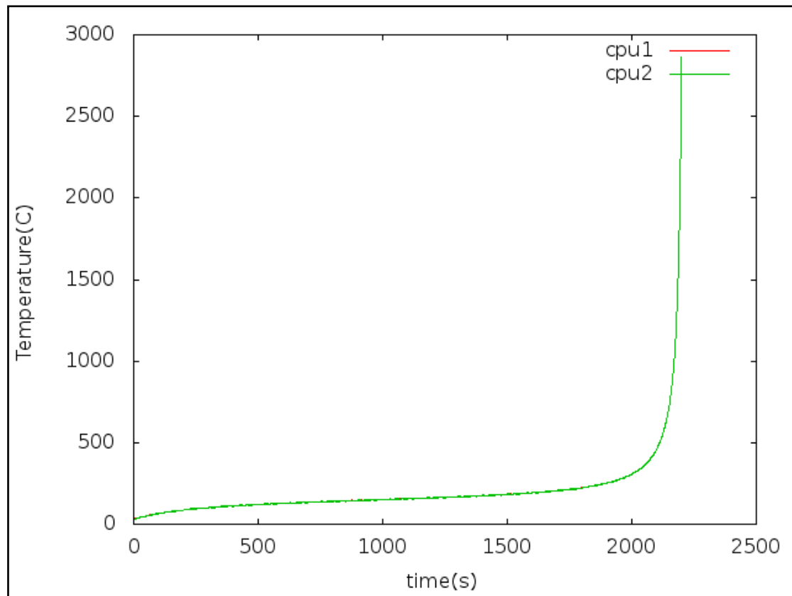
Figure 3.15 : Simulation par ATMI de l’emballage thermique observé sur un MPC5517E
