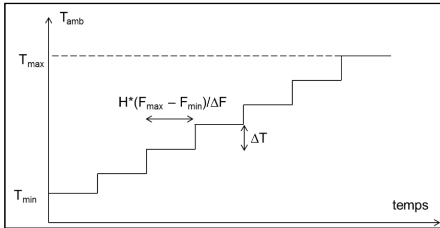
Figure 4.3 : Variation de la température ambiante dans ATMI
