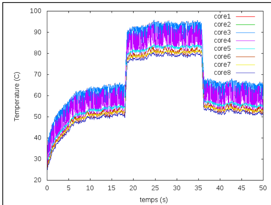
Figure 5.26 : Variation en température de l'architecture à 2 cœurs à 1200 MHz (avec RM).
