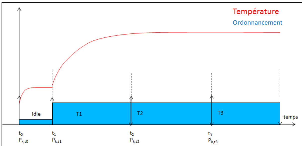
Figure 4.2 : Ordonnancement de 3 tâches sur un seul cœur à fréquence minimal
