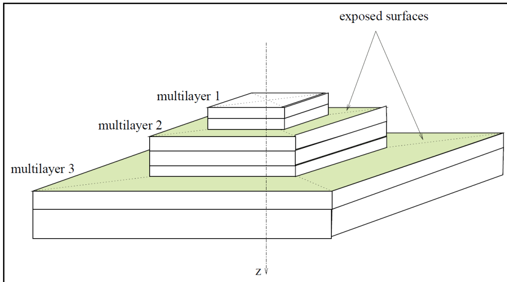
Figure 3.12 : Principe de modélisation d'un circuit avec STiMuL.
