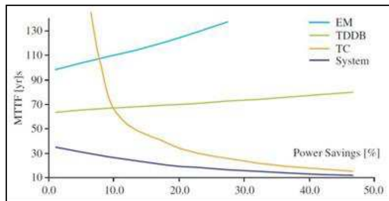
Figure 1.2 : Impact sur le MTTF des techniques classiques de réduction d'énergie/puissance
