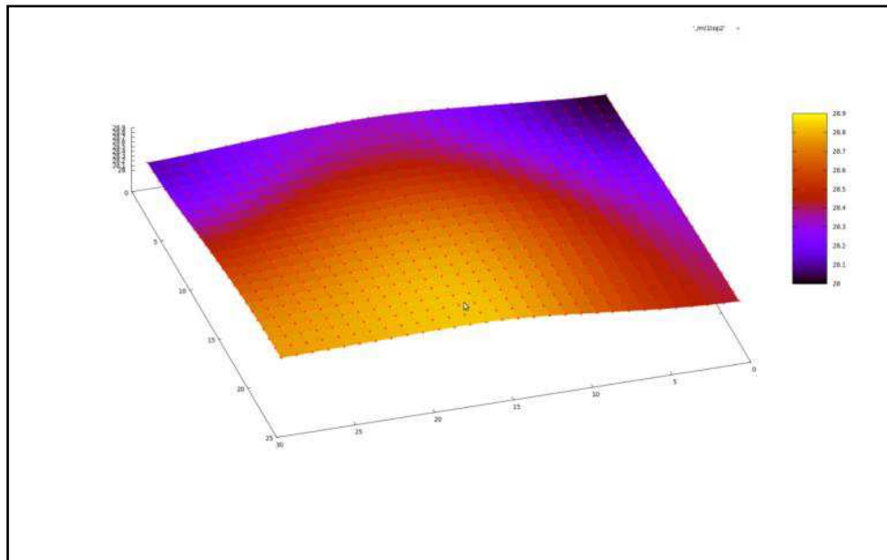
Figure 3.14 : Résultat de STiMul sur le modèle du MPC5517E décapsulé.
