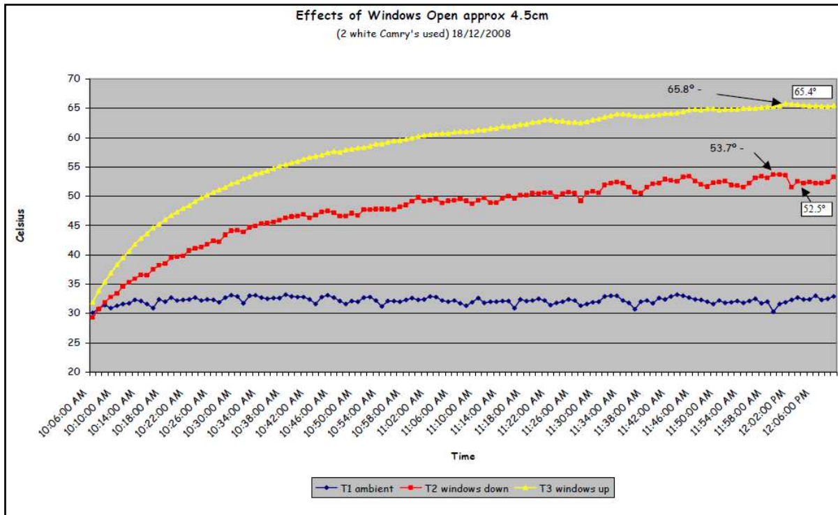
Figure 2.4 : Différences de température intérieure avec fenêtres fermées (courbe jaune) et fenêtres ouvertes (courbe rouge)
