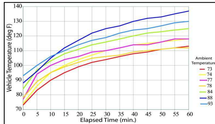
Figure 2.3 : Variation de la température intérieure de l'automobile pour différentes températures extérieures.
