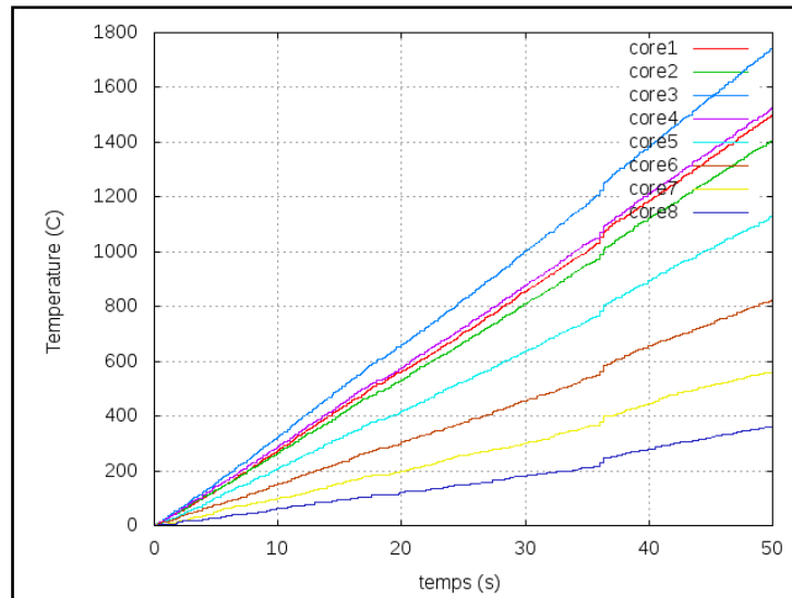
Figure 5.28 : Cycles thermiques correspondent à l'évolution en température de la Figure 5.25
