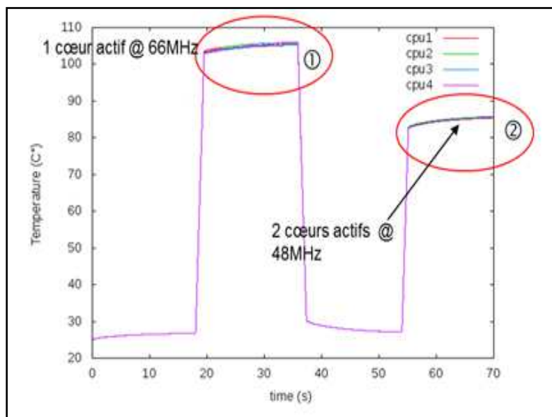
Figure 5.19 : Changement périodique de configuration
