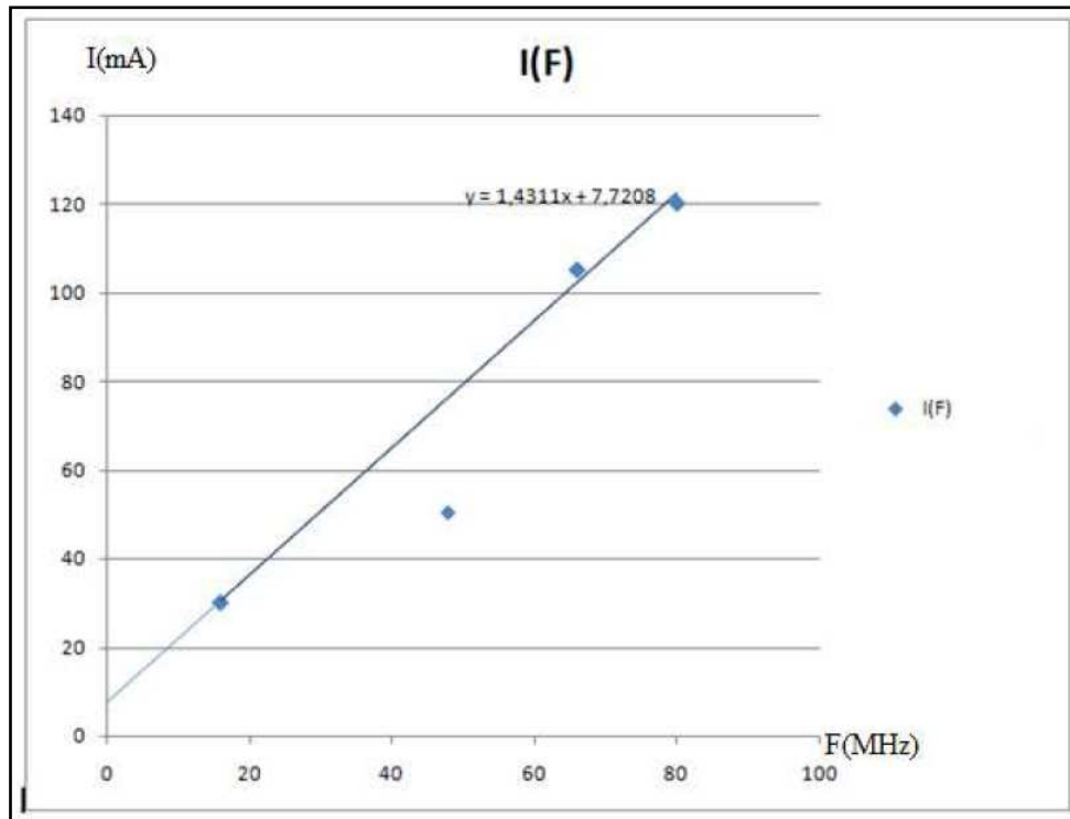
Figure 3.8 : Courbe de courant en fonction des fréquences à température ambiante 25°C
