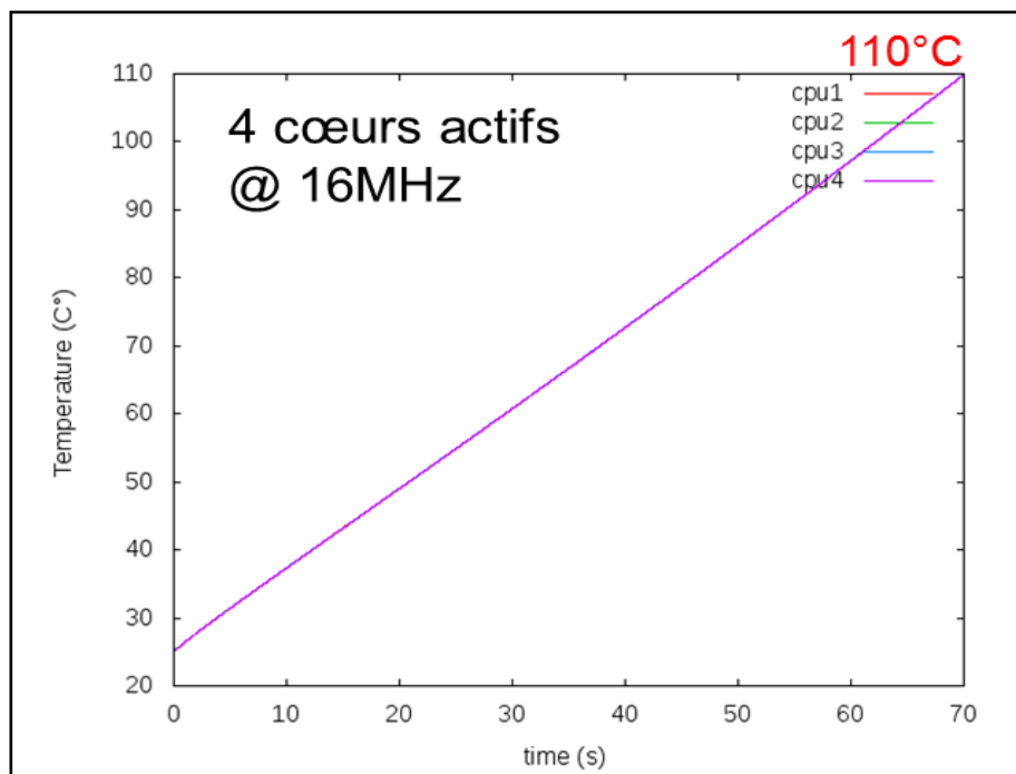
Figure 5.3 : Variation en température de l'architecture à 4 cœurs actifs à 16MHz (EDF)
