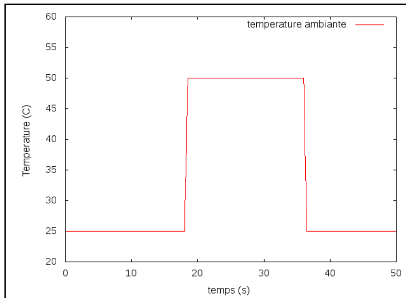
Figure 5.24 : Exemple considéré de variation de la température ambiante pour le Ultra Sparc T1
