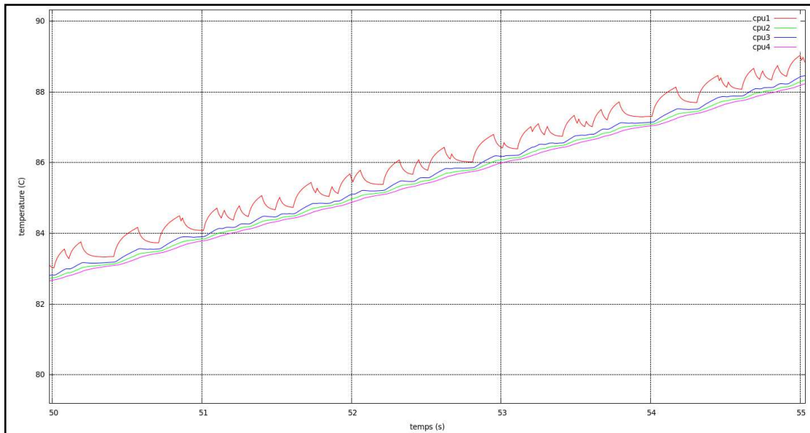
Figure 5.5 : Cycles thermiques d'un cœur fonctionnant à 80MHz (EDF)
