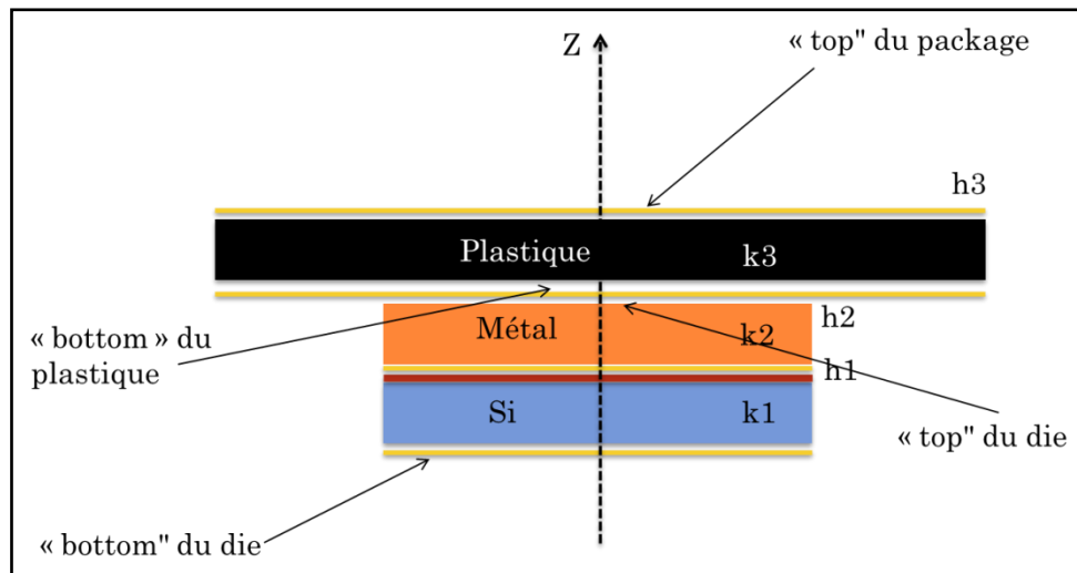
Figure 3.16 : Modèle en trois couches du circuit sous STiMuL.
