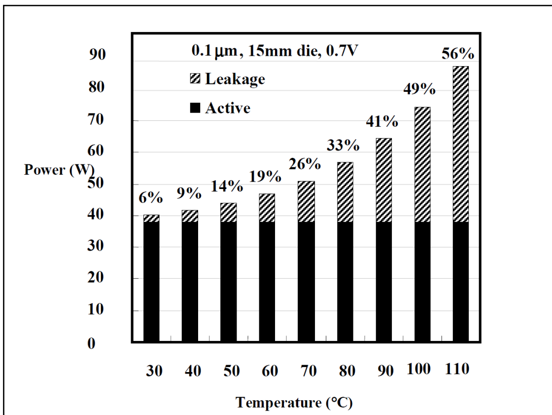
Figure 2.5 : Puissance consommée au niveau du die en fonction de la température.
