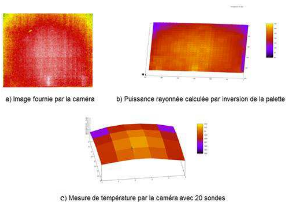
Figure 3.11 : Calcul de la puissance rayonnée à partir de l'image fournie par la caméra thermique
