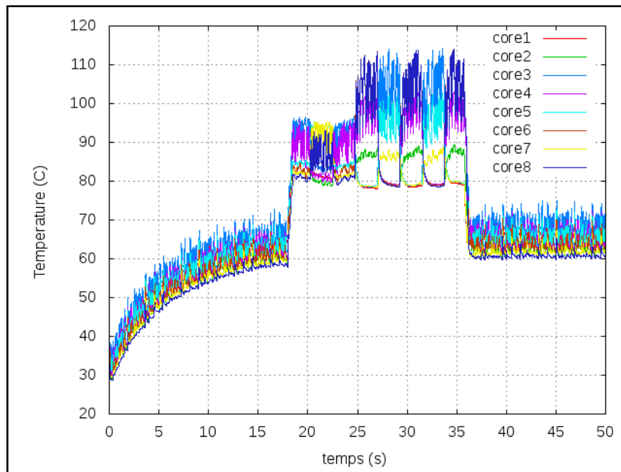
Figure 5.27 : Variation en température de l'architecture en appliquons notre approche.
