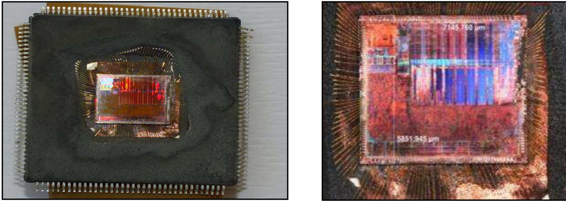
Figure 3.4 : Circuit MPC5517 décapsulé
