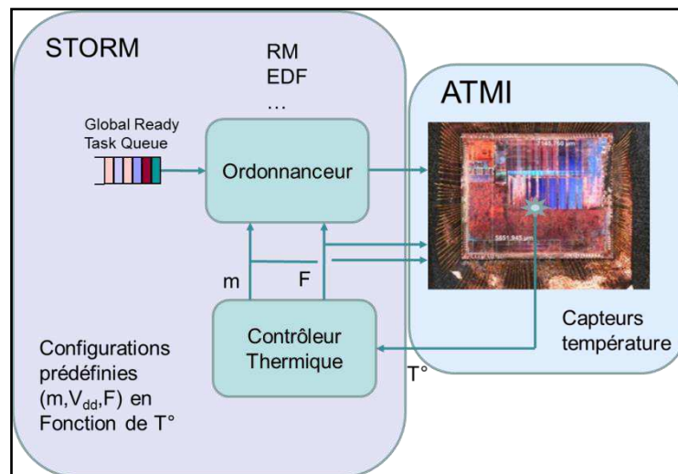
Figure 3.18 : Contrôleur thermique construit par couplage de STORM et ATMI.
