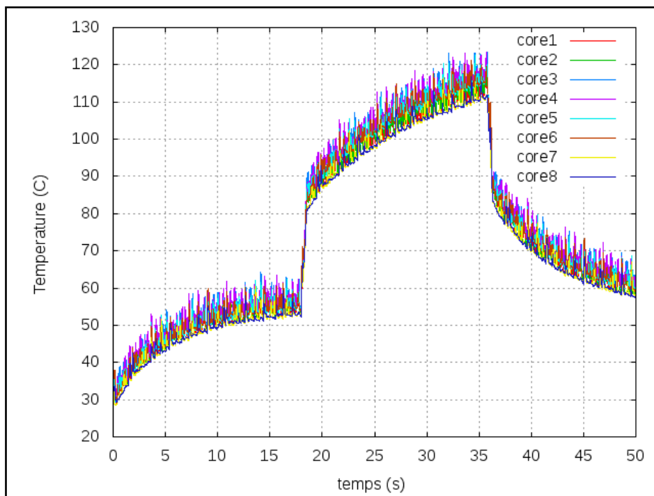
Figure 5.25 : Variation en température de l'architecture à 8 cœurs à 720 MHz (avec RM).
