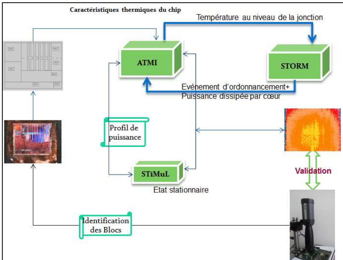
Figure 3.1 : Flot de modélisation retenu
