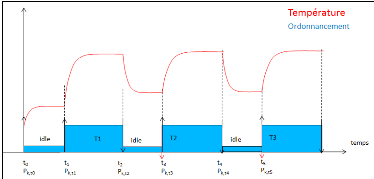
Figure 4.1 : Ordonnancement de 3 tâches sur un seul cœur à fréquence élevée
