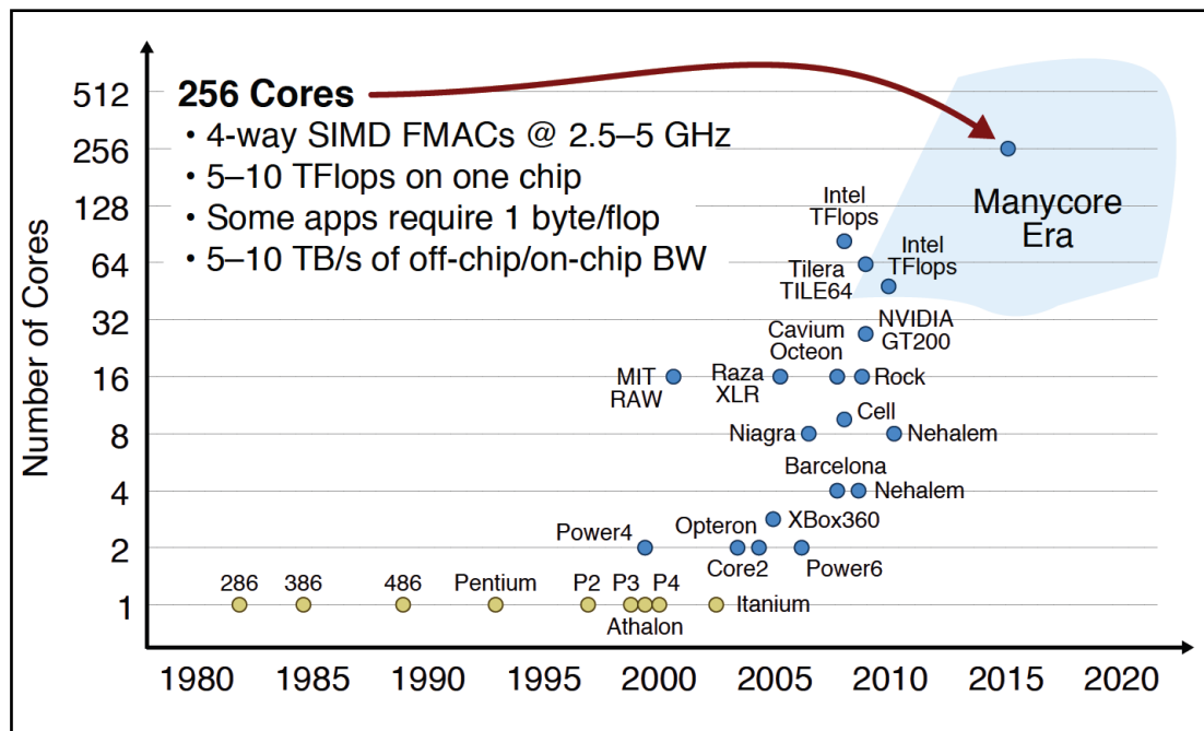
Figure 1.1: Evolution du nombre de cœurs intégrés dans les architectures [3]
