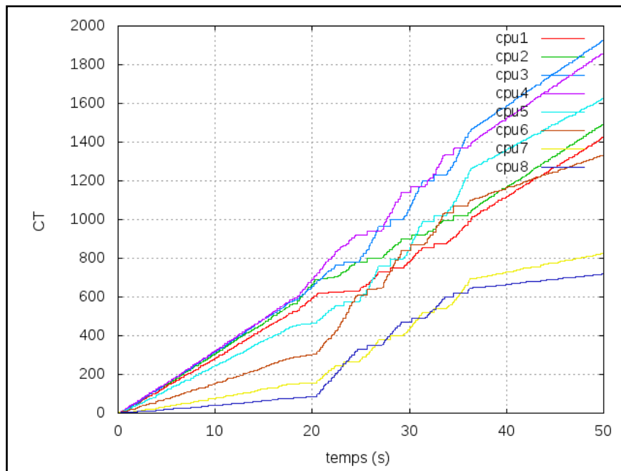
Figure 5.30 : Cycles thermiques correspond à l'évolution en température de la Figure 5.27
