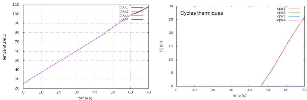
Figure 5.14 : Action du contrôleur thermique sur la température des cœurs, U= 60%, RM
