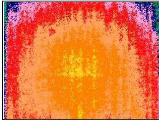
Figure 3.5 : Image thermique du MPC5517 avec le cœur z1 actif (suite d'additions entre registres) et le cœur z0 sous tension.
