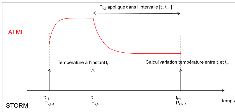
Figure 3.19 : Principe du calcul de la température par ATMI à partir des informations fournies par STORM
