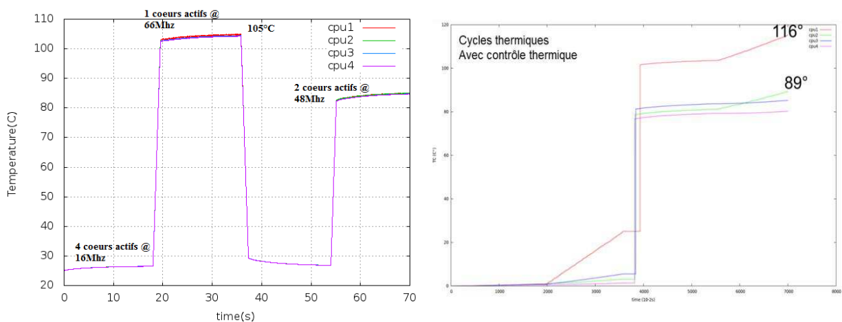
Figure 5.15 : Résultats obtenus avec gestion des cycles thermiques, U=60%, RM
