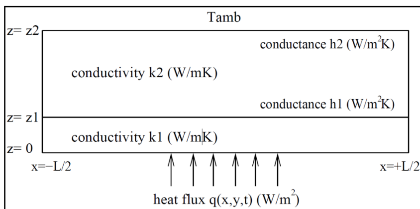
Figure 3.10 : Principe de la modélisation d'un circuit par ATMI
