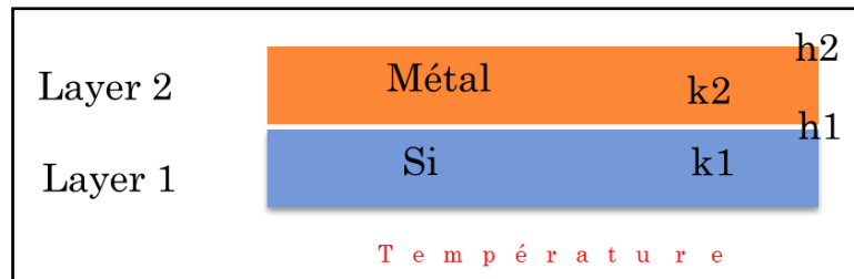
Figure 3.13 : Premier modèle en deux couches sous STiMuL correspondant au chip décapsulé.
