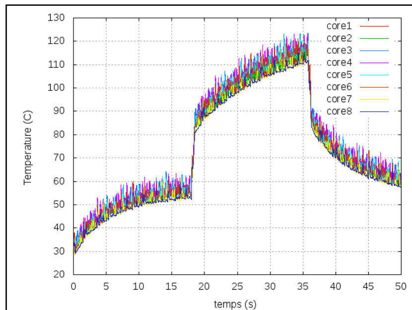
Figure 5.25 : Variation en température à 8 cœurs à 720 MHz (avec RM).
