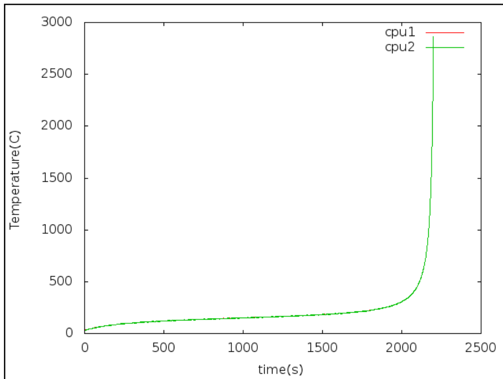
Figure 3.15 : Simulation par ATMI de l'emballement thermique observé sur un MPC5517E
