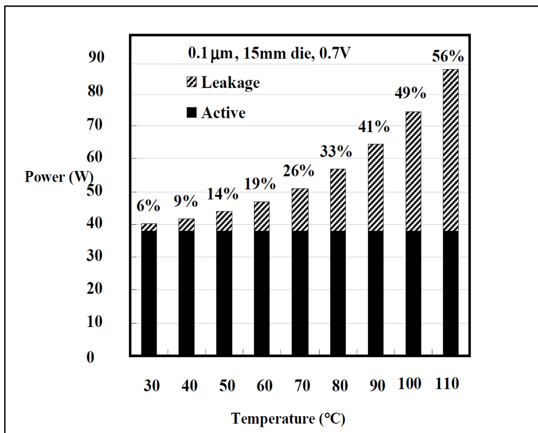
Figure 2.5 : Puissance consommée au niveau du die en fonction de la température.
