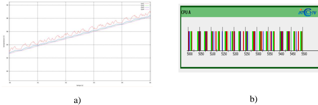
Figure 5.7 : Cycles thermiques (a) et Ordonnancement (b) pour un cœur fonctionnant à 80MHz (EDZL)
