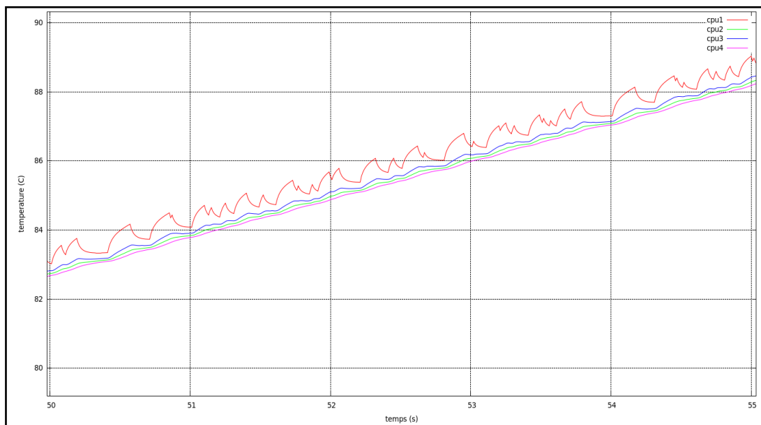
Figure 5.5 : Cycles thermiques d'un cœur fonctionnant à 80MHz (EDF)
