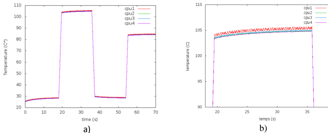
Figure 5.9 : Température des cœurs : 1 cœur actif à 80MHz suivant RM
