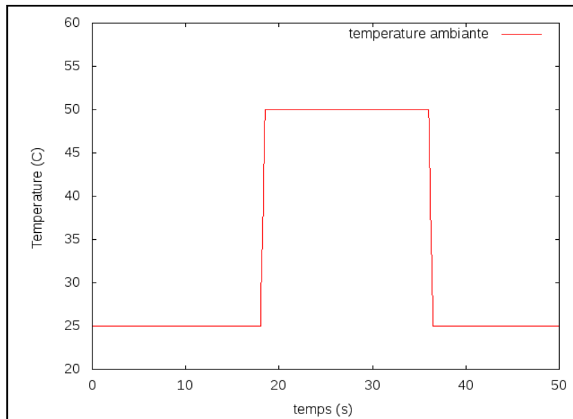
Figure 5.24 : Exemple considéré de variation de la température ambiante pour l'Ultra Sparc T1
