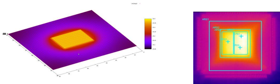
Figure 3.17 : Simulation sous STiMuL (à gauche) et image issue de la caméra thermique (à droite) du MPC5517
