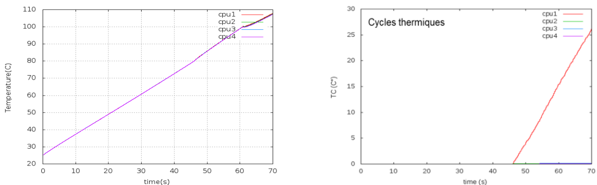
Figure 5.14 : Action du contrôleur thermique sur la température des cœurs, U= 60%, RM
