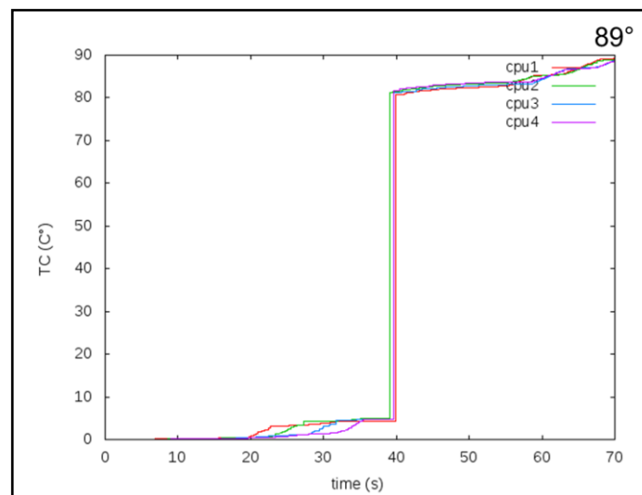
Figure 5.21 : Effet des changements périodiques d'états actifs/inactif sur les cycles thermiques
