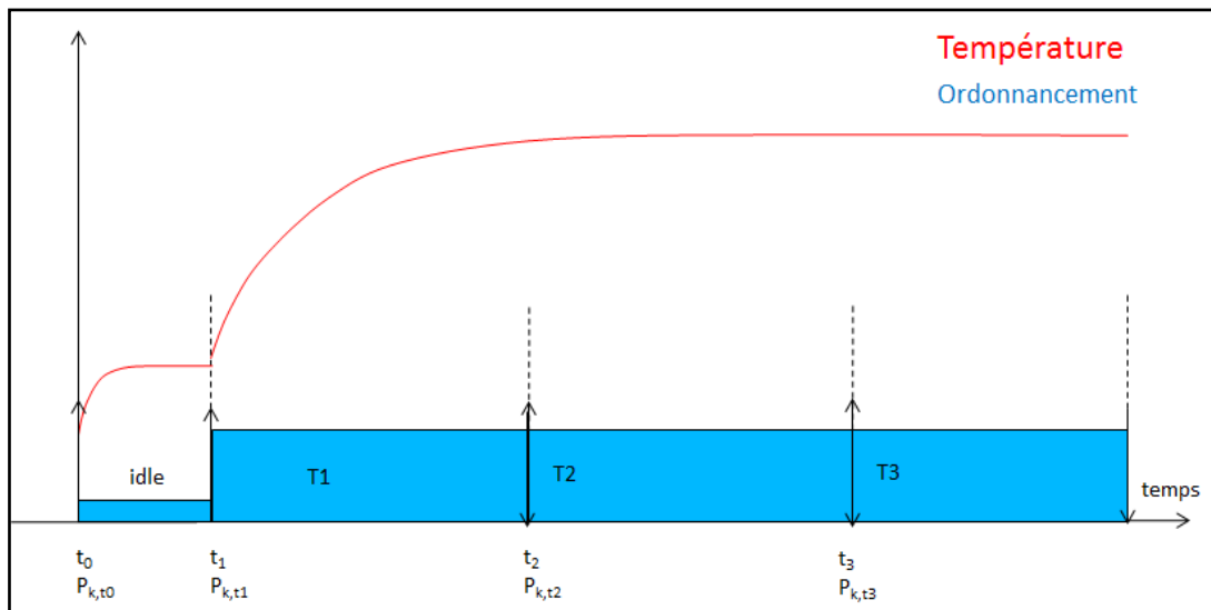
Figure 4.2 : Ordonnement de 3 tâches sur un seul cœur à fréquence minimal
