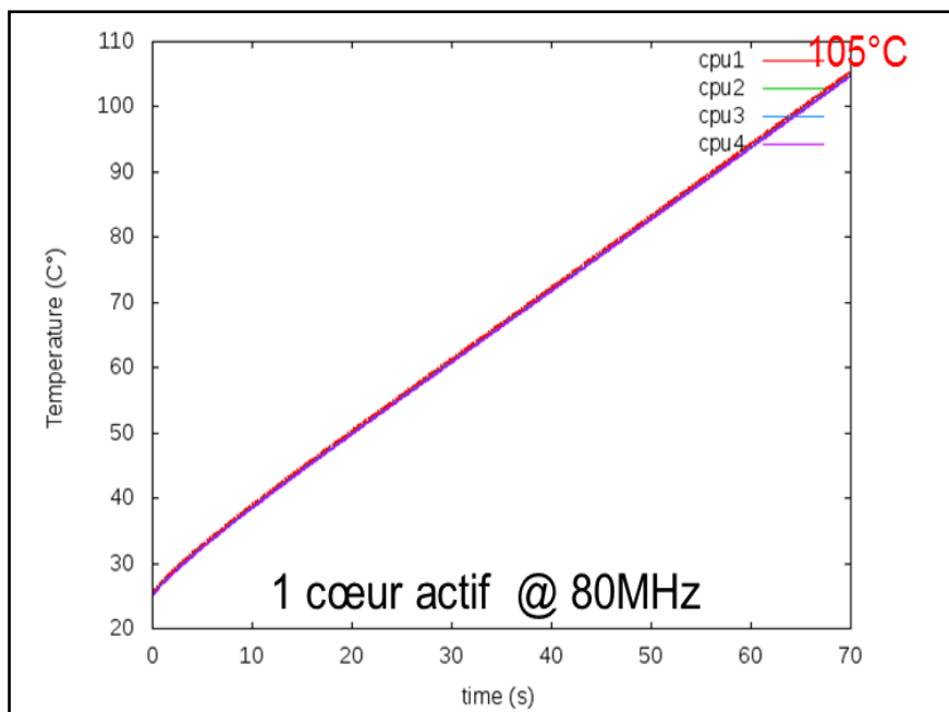
Figure 5.4 : Variation en température de l'architecture à 4 cœurs à 80 MHz (EDF) dont un seul est actif.
