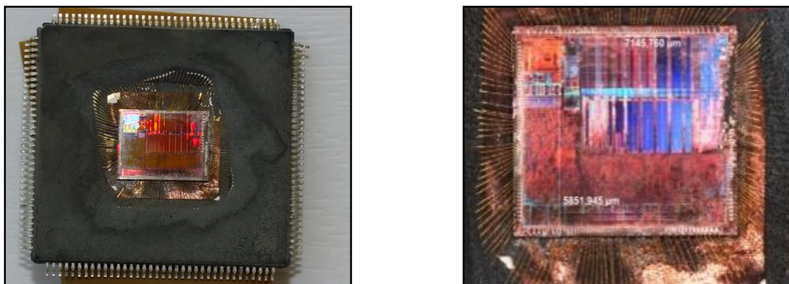
Figure 3.4 : Circuit MPC5517 décapsulé
