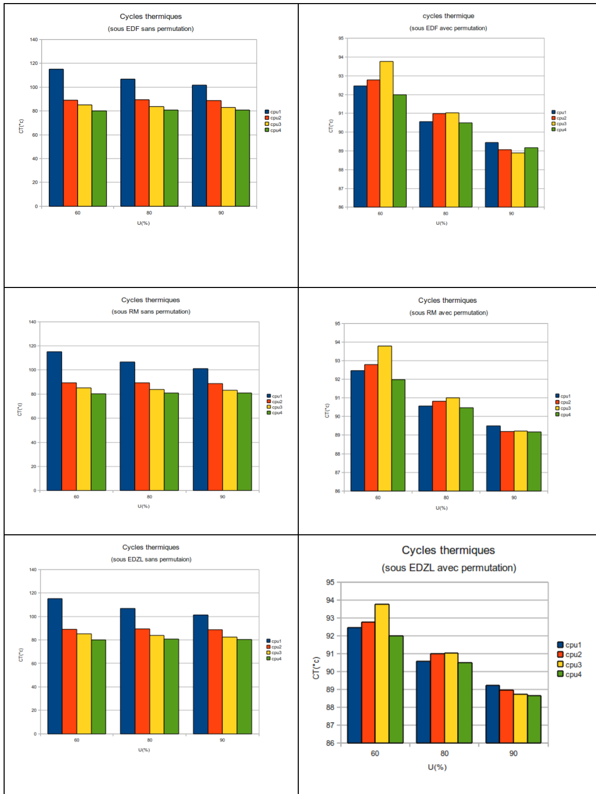
Figure 5.22 : Cycles thermiques subi par les différents cœurs suivant les 3 algorithmes globaux considérés, et sous les différentes charges processeurs.
