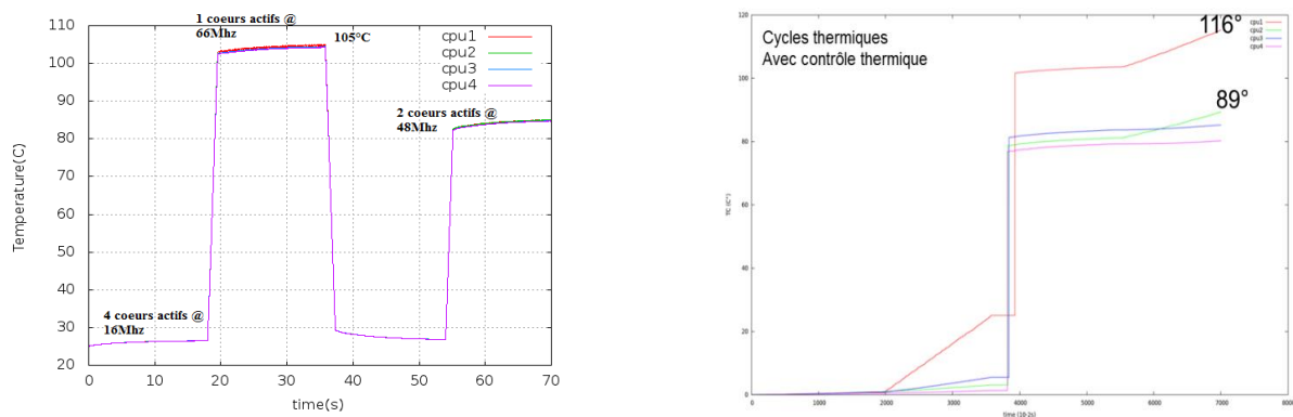
Figure 5.15 : Résultats obtenus avec gestion des cycles thermiques, U=60%, RM
