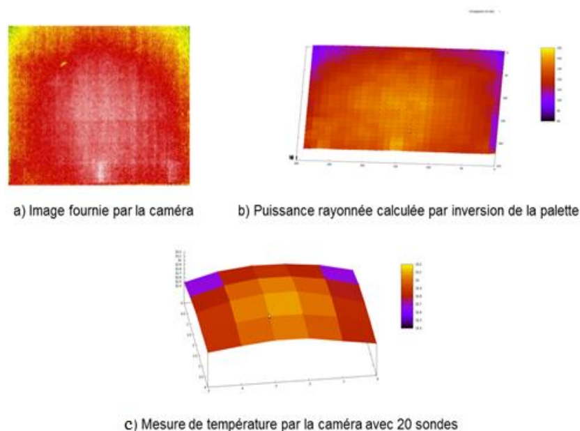
Figure 3.11 : Calcul de la puissance rayonnée à partir de l'image fournie par la caméra thermique
