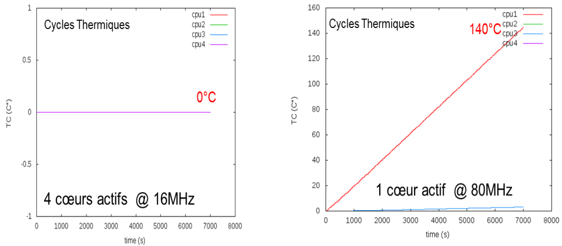
Figure 5.10 : Cycles thermiques cumulés par processeur
