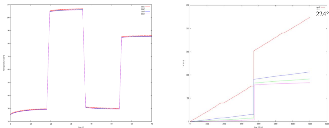
Figure 5.12. Résultats pour EDZL, 1 processeur à 80MHz, taux d'utilisation de 90% : variation de température (figure de gauche) et cycles thermiques subis (figure de droite).
