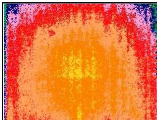
Figure 3.5 : Image thermique du MPC5517 avec le cœur z1 actif (suite d'additions entre registres) et le cœur z0 sous tension.
