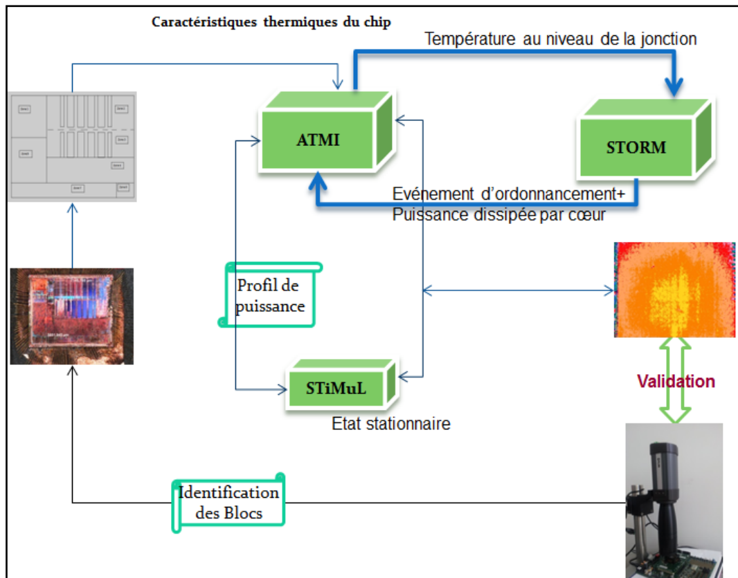
Figure 3.1 : Flot de modélisation retenu
