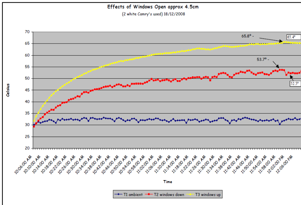
Figure 2.4 : Différences de température intérieure avec fenêtres fermées (courbe jaune) et fenêtres ouvertes (courbe rouge)
