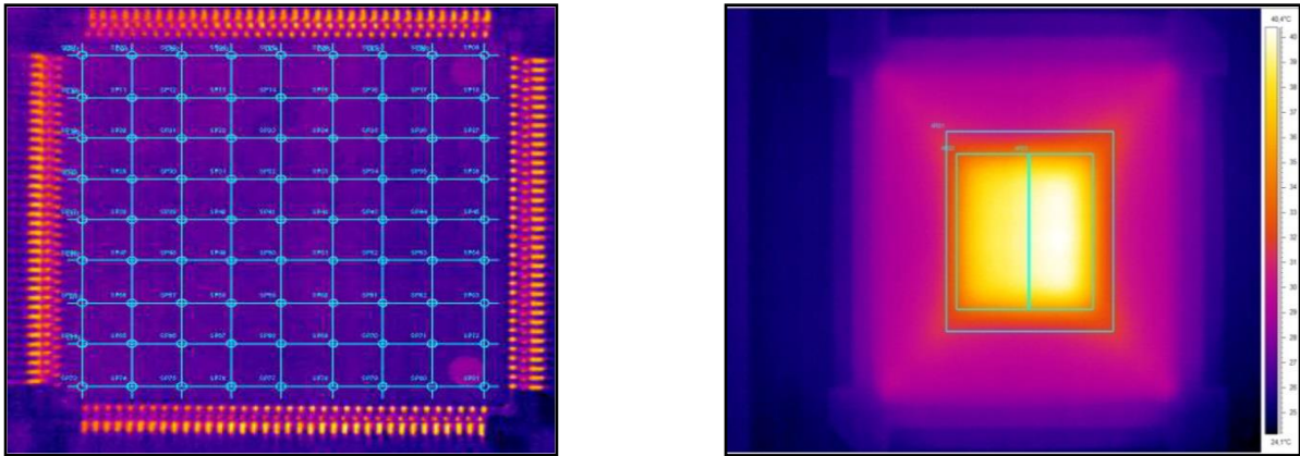
Figure 3.3 : Circuit encapsulé vu par la caméra thermique
