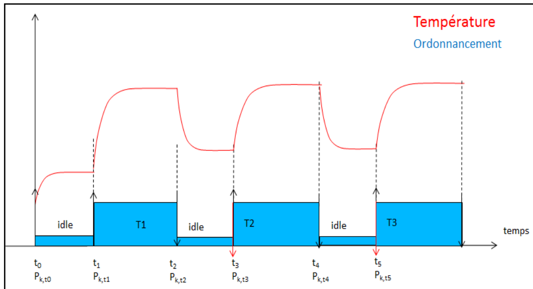
Figure 4.1 : Ordonnancement de 3 tâches sur un seul cœur à fréquence élevée
