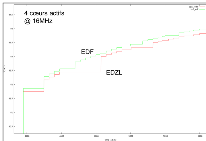
Figure 5.18 : Cycles thermiques pour EDF et EDZL pour U=90\% entre les instants 44s et 54s.
