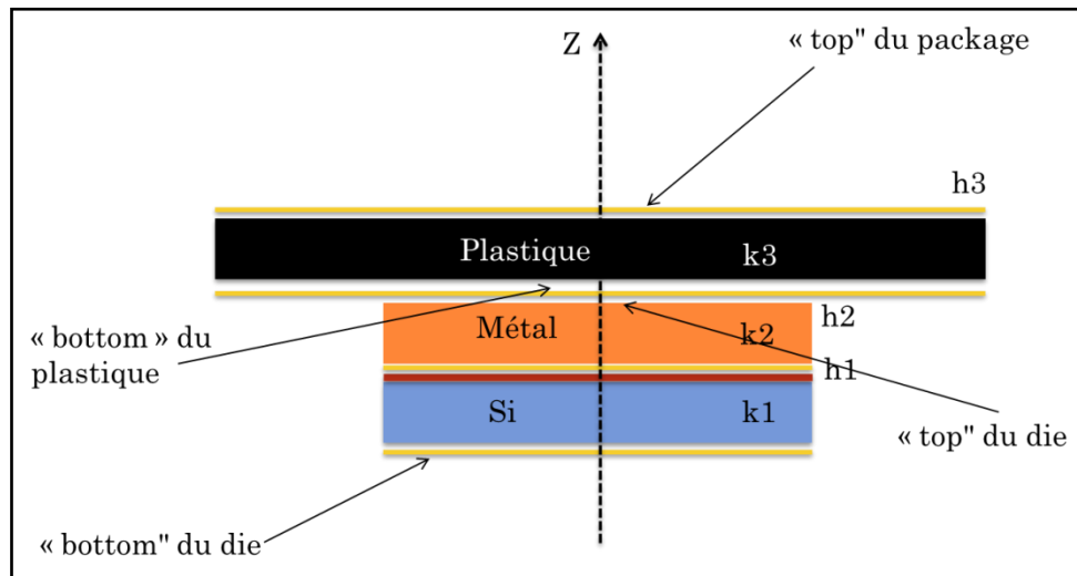
Figure 3.16 : Modèle en trois couches du circuit sous STiMuL.
