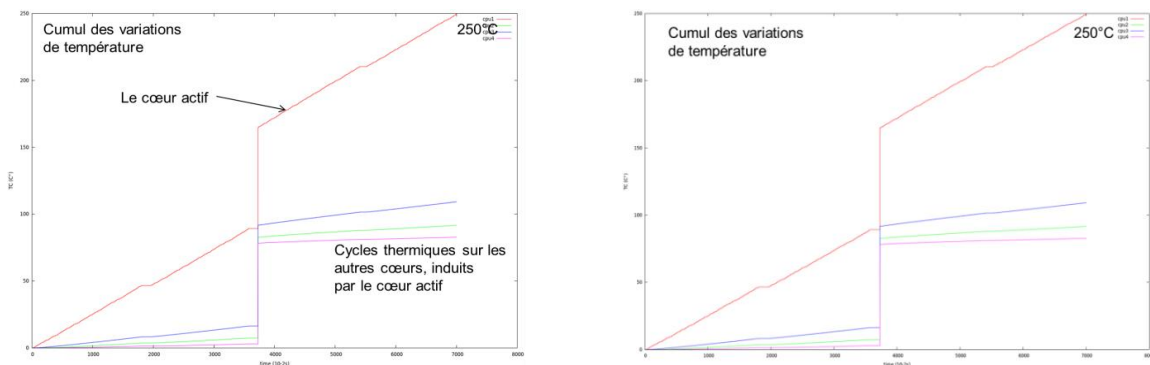
Figure 5.11 : Cycles thermiques avec 1 cœur actif à 80MHz ordonnancé suivant RM (figure de gauche) et EDF (figure de droite)
