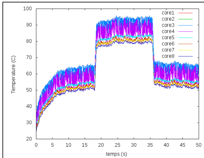
Figure 5.26 : Variation en température de l'architecture à 2 cœurs à 1200 MHz (avec RM).
