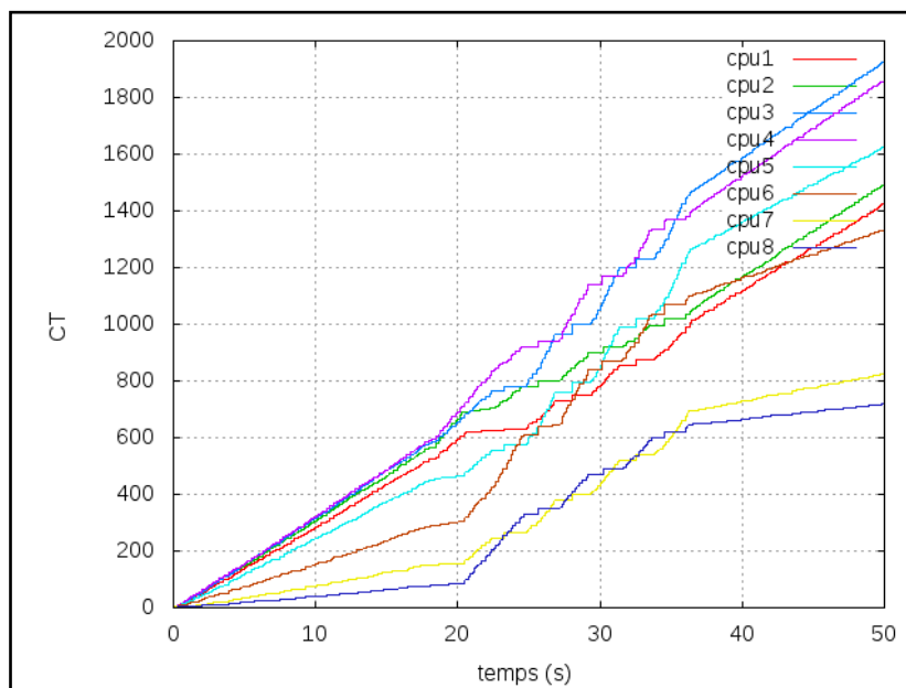
Figure 5.30 : Cycles thermiques correspondent à l'évolution en température de la Figure 5.27
