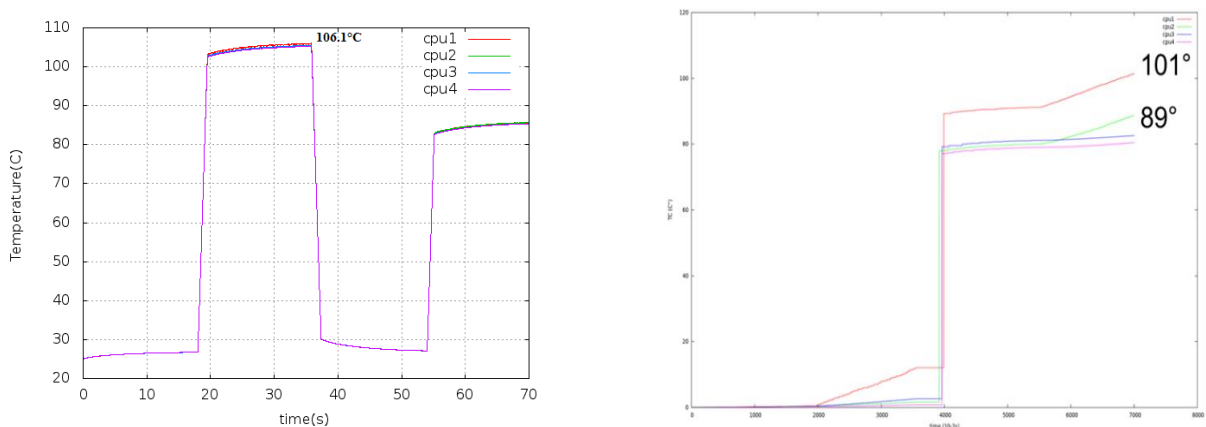
Figure 5.17 : Résultats avec EDZL et U=90%
