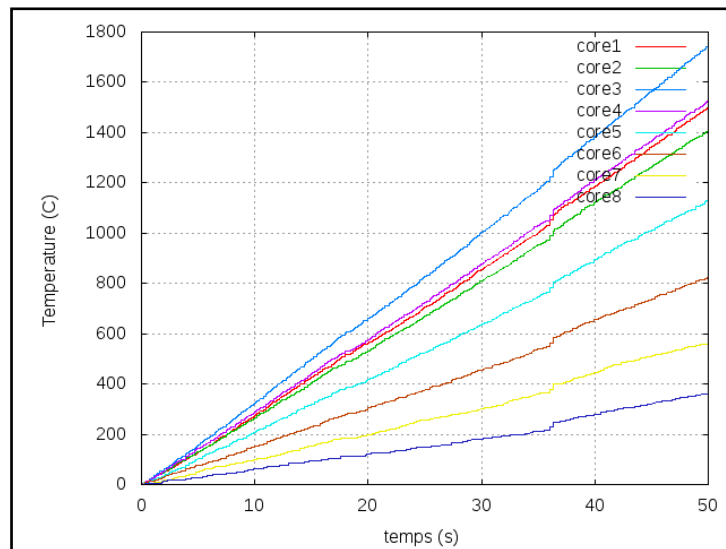
Figure 5.28 : Cycles thermiques correspondant à l'évolution en température de la Figure 5.25
