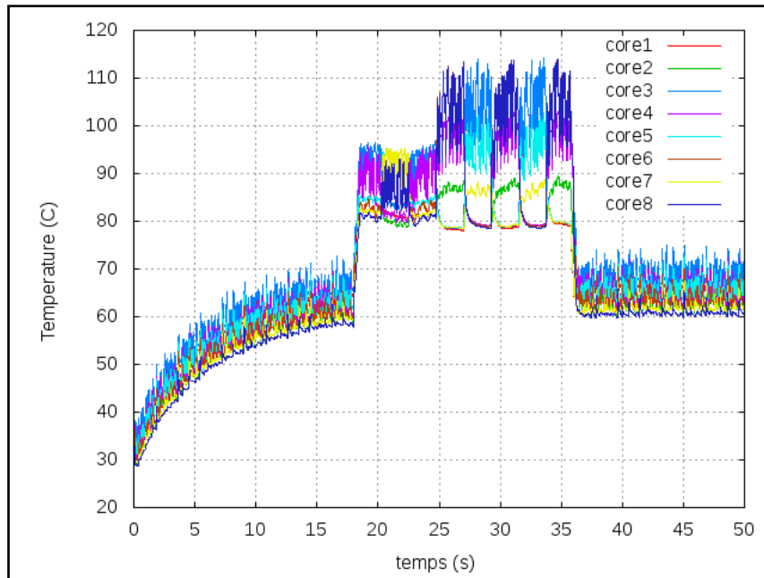
Figure 5.27 : Variation en température de l'architecture en appliquons notre approche.
