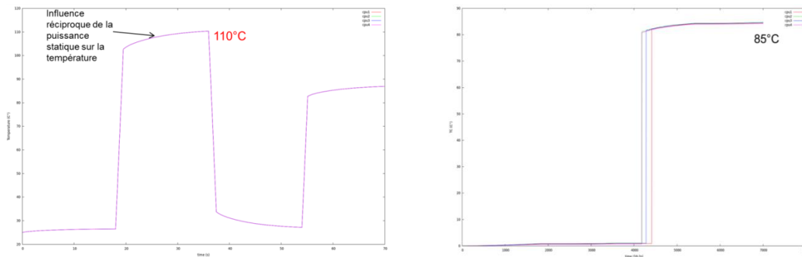
Figure 5.13 : Variation en température (figure de gauche) et cycles thermiques (figure de droite) avec 4 cœurs actifs à 16MHz et le jeu de tâches ayant un taux d'utilisation de 60%
