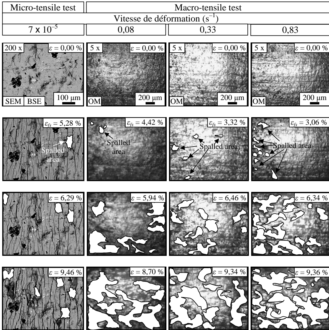
Figure 5: évolution de l'écailage en fonction de la déformation pour l'acier recyclé ( \varepsilon = déformation).
