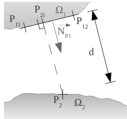
Figure I.35 : Schématisation de l'appariement type nœud-segment .
