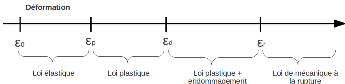
Figure I.30 : Schéma récapitulatif des lois de comportement, avec \epsilon_0 = 0 , \epsilon_p = Déformation élastique limite, \epsilon_d = \frac{1}{2} \epsilon_r ou \frac{3}{4} \epsilon_r , \epsilon_r = déformation à la rupture.
