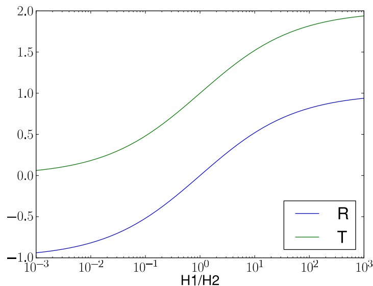
Figure 2.24 ► Valeur des coefficients de réflexion et transmission pour différentes valeurs du gradient de topographie.
