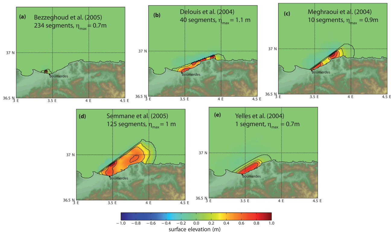
Figure 4.1 ► Les différentes surfaces de déformation en mer générées par les sources utilisées. Les calculs de la déformation de surface ont été faits par les formules d'Okada (1985)
