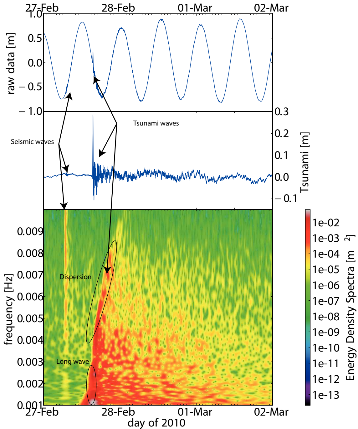
Figure 1.2 ► Enregistrement du tsunami de Maule 2010 par le DART 51406 (proche de Hawaii) en (a) l'enregistrement brut, en (b) l'enregistrement filtré afin de ressortir le signal du tsunami, et en (c) l'analyse temps fréquence du signal obtenu. Plusieurs arrivées peuvent être observées : l'arrivée des ondes sismiques, des ondes tsunamis en deux phases, les ondes dites longues et les ondes dispersives.
