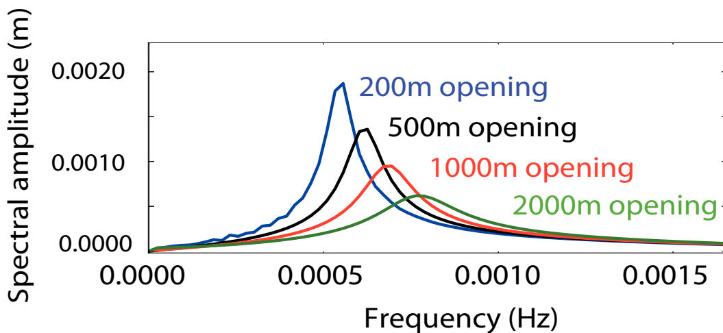
Figure 2.23 ► Détail sur le mode de Helmholtz (mode le plus grave) dans les quatre ouvertures de bassin. La taille de l'ouverture a un effet sur l'amplitude et la largeur de ce mode de résonance.
