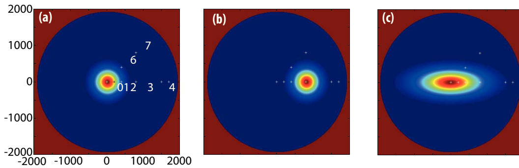
Figure 2.17 ► Représentation du bassin de calcul de mode de résonance (bassin circulaire de 1900 m de rayon et 100 m de profondeur) la position des différents capteurs est représentée par des "+". Trois simulations ont été effectuées avec trois configurations de surface initiales de déformation : (a) source symétrique centrée, (b) source symétrique décentrée, (c) source non symétrique centrée.
