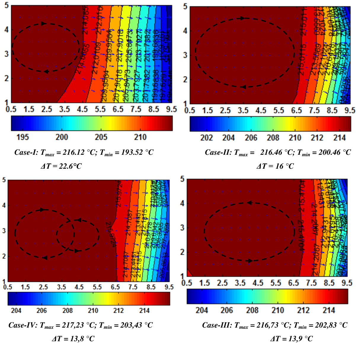
Figure V.17. Cartes de température couplées aux vecteurs des gradients thermiques locaux pour les quatre expériences de solidification (LH19, LH22, LH25 et LH29), à l'instant t_i = 15\text{mn} . Les conditions expérimentales sont: Sn-10wt.%Pb, \Delta T = 40\text{K} , CR = 0,03\text{K/s} , courant appliqué I = 8,2\text{A} .
