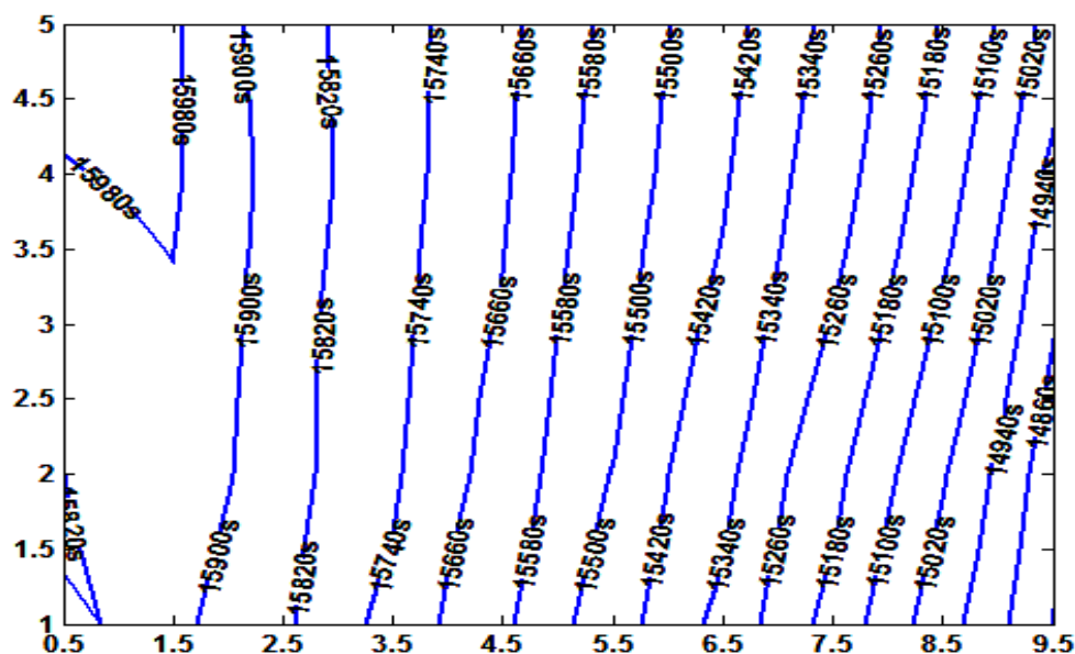
Figure IV.18. Positions du front de solidification avec les temps correspondants, prises pour l'isotherme 224,7^{\circ}\text{C} supposé comme la ligne des pointes de dendrites (surfusion de 3.44^{\circ}\text{C} ). Sn-3wt.%Pb, \Delta T = 40\text{K} , CR = 0,03\text{K/s} .
