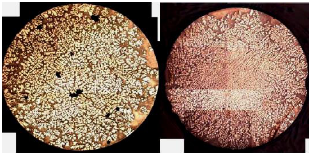
Figure II.13. Coupe radiale après 2 cm de solidification dans le cas d'une force de brassage ascendante ( F^+ ). A gauche : B = 10\text{ mT} et G_l = 28\text{ K.cm}^{-1} . A droite B = 30\text{ mT} et G_l = 24\text{ K.cm}^{-1} . Dans les deux cas, l'extérieur du lingot est constitué d'une couche eutectique K. Zaidat et al [51].
