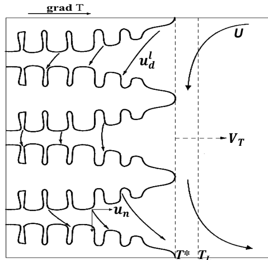
Figure. V.22. Représentation schématisée des vitesses de convection dans le liquide, U , et dans les régions interdendritiques, u_d^l , et sa projection sur le gradient de température, parallèle à la direction d'avancement des isothermes, u_n . La vitesse d'avancement des isothermes est notée V_T .
