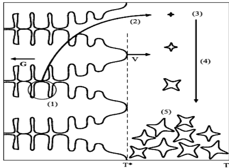
Figure. I.23. Représentation schématisée de la transition colonnaire-équiaxe. Dans ce cas, la surfusion colonnaire est supérieure à la surfusion de germination, la germination en avant du front peut avoir lieu et conduire à une structure équiaxe [54].
