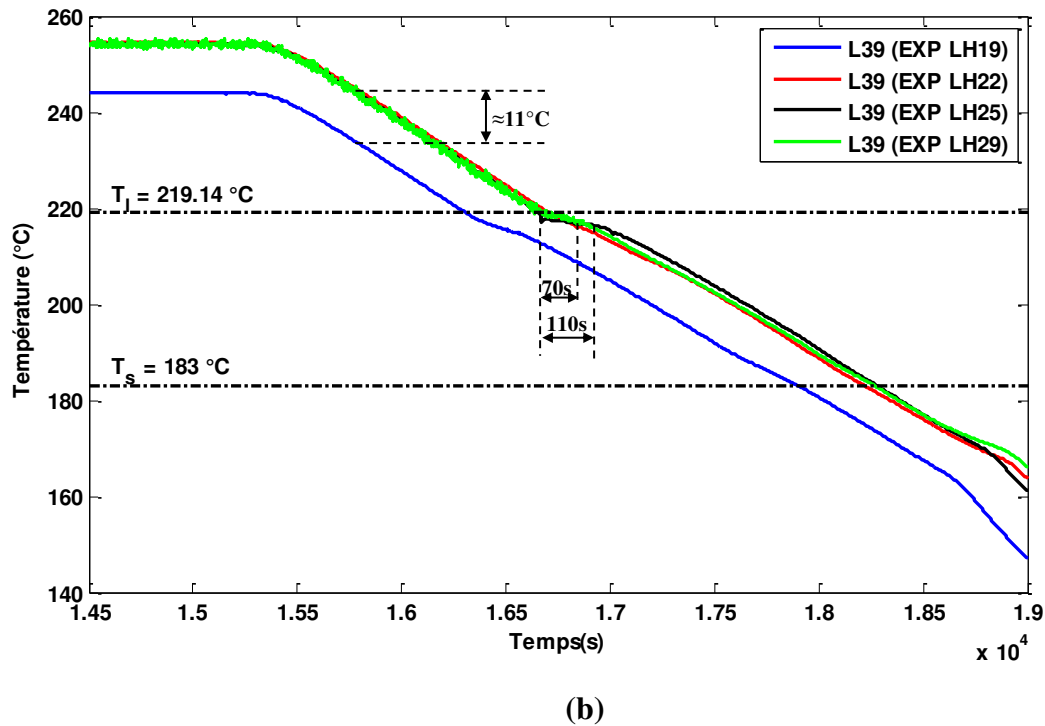
Figure V.14. Les courbes de refroidissement obtenues à partir des données expérimentales. (a) thermocouple L23 et (b) thermocouple L39, pour les trois cas de brassage décrits précédemment comparés au cas de solidification sous la convection naturelle (thermosolutale). Les conditions expérimentales: Sn-10wt.%Pb, \Delta T = 40K , CR = 0,03K/s , courant appliqué I = 9,5A , fréquence f = 50Hz , conductivité électrique de l'alliage \sigma = 1.86 \times 10^6 \Omega^{-1}.m^{-1} , champ magnétique B_0 = 45mT .
