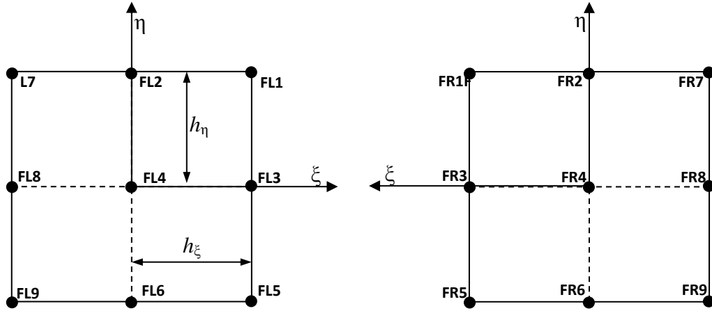
Figure A.II.1. Schéma illustratif de la répartition des thermocouples de chaque échangeur sur un élément quadratique complet.
