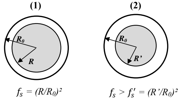
Figure.V.20. Illustration schématique de la refusion d'un bras de dendrite de section circulaire
