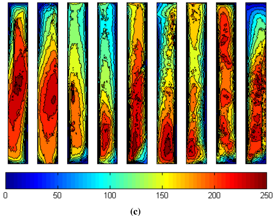
Figures IV.34. Position des coupes transversales (a) ; Radiographie X des coupes transversales (b) ; Carte des contours des iso-concentrations (c) ; Expérience. Sn-3wt.%Pb (Réf LH5), \Delta T = 40K , CR = 0,03K/s . les neuf tranches sont numérotées de droite à gauche.
