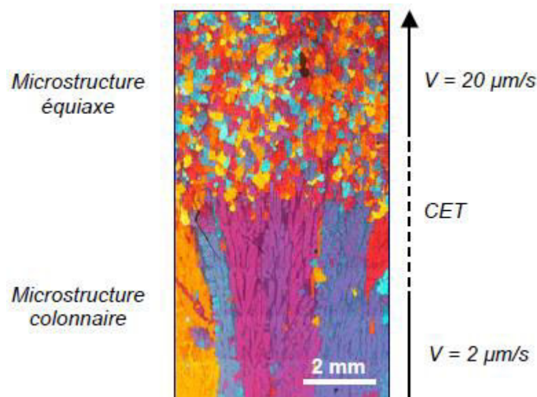
Figure I.22 : Coupe longitudinale d'un barreau cylindrique d'alliage Al-3,5% pds Ni affiné pour lequel la transition d'une microstructure colonnaire à une microstructure équiaxe a été obtenue en appliquant une augmentation de la vitesse de solidification (H. Jung, L2MP).
