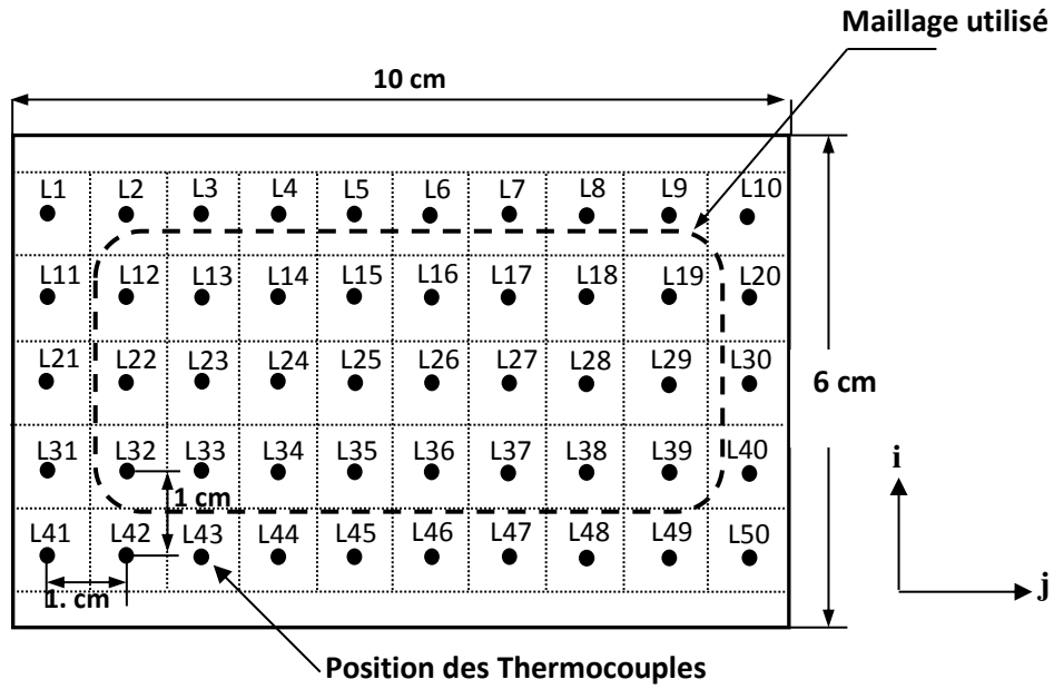
Figure A.II.2. Sous-domaine contenant les points choisis pour le calcul du champ de vitesse représenté par la zone délimitée par la ligne discontinue.
