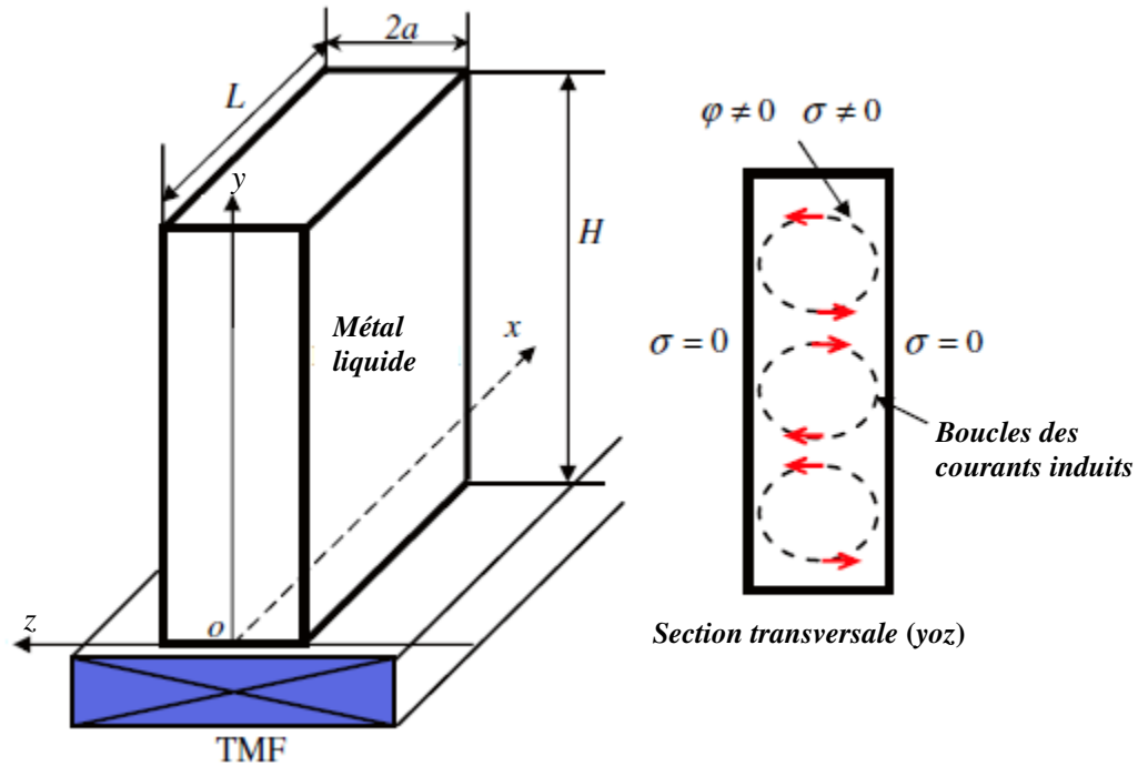
Figure V.2. Géométrie, notations, et schéma illustratif des courants éclectiques induits dans un domaine confiné de métal liquide.
