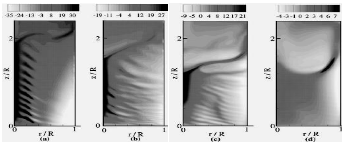
Figure. II.14. Simulation numérique de la solidification de l'alliage Al-7wt.%Si, sous l'influence de RMF pour B_0=4\text{mT} et différents f_p . Tracés de contour de la concentration relative \frac{c_{\text{Si}}-c_0}{c_0} \cdot 100 dans l'échantillon solidifié: (a) RMF continu, (b) f_p = 0,17\text{Hz} , (c) f_p = 0,33\text{Hz} et (d) f_p = 0,75\text{Hz} , B. Willers et al [57].
