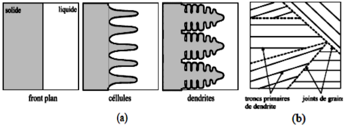
Figure. I.13. Représentation schématisée des différentes morphologies d'interfaces et des microstructures résultantes (a). Représentation schématisée d'une structure macroscopique du grain lors de croissance dendritique (b) [54].
