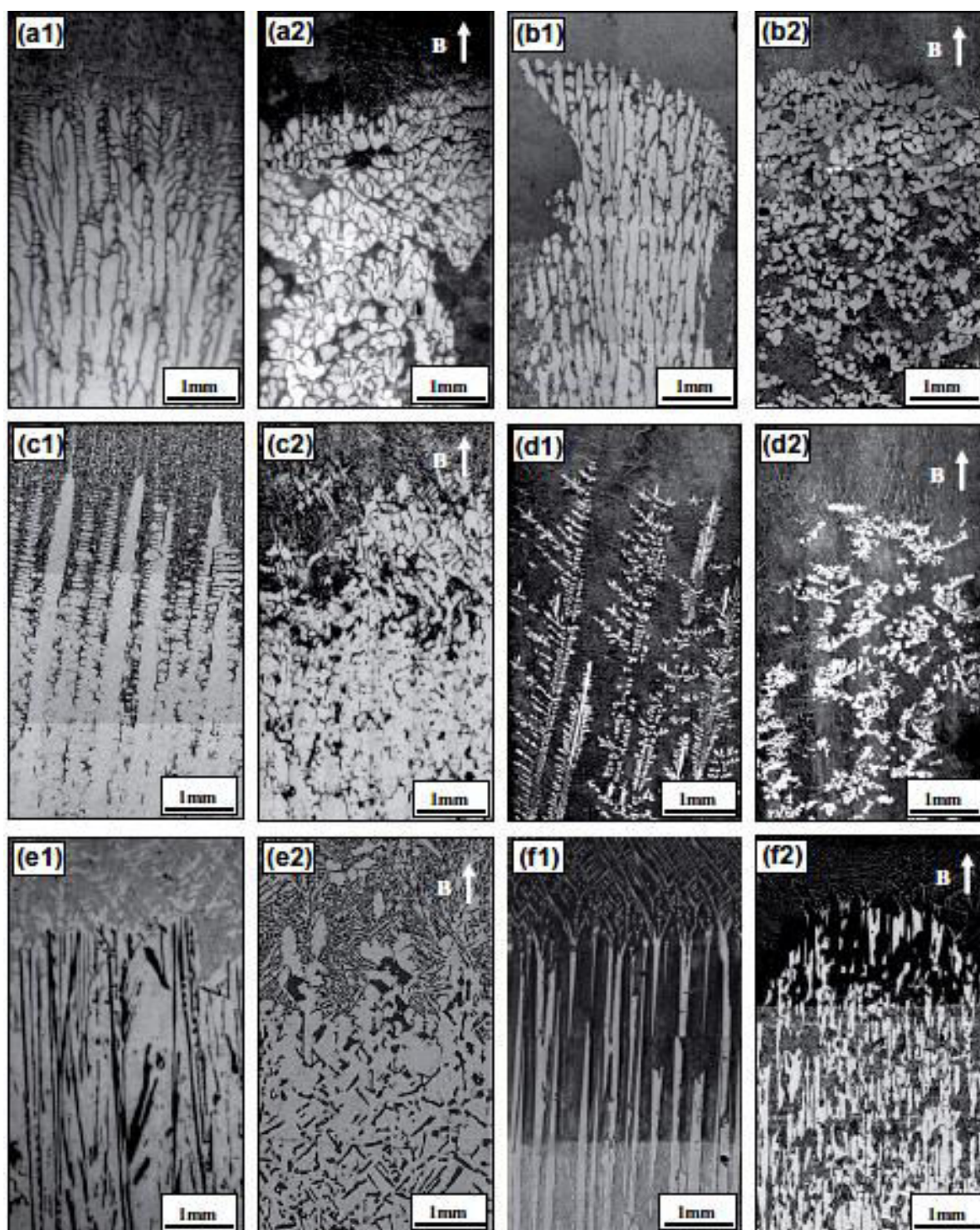
Figure.II.11. Microstructure à l'interface liquide-solide pour une solidification dirigée de six alliages sans et avec un fort champ magnétique: (a) Al dendrites dans l'Alliage Al-4.5wt.%Cu, 10T, 10\mu\text{m.s}^{-1} , (B) Sn dendrites dans l'alliage Pb-80wt.%Sn, 10T, 1\mu\text{m.s}^{-1} (C) \gamma dendrites dans DZ417G superalliage, 6T, 5\mu\text{m.s}^{-1} [58] (d) \gamma dendrites dans l'alliage Zn-5wt.%Cu, 10T, 10\mu\text{m.s}^{-1} (E) Si dendrites dans l'alliage Al-15wt.%Si, 10T, 1\mu\text{m.s}^{-1} (f) \text{Al}_2\text{Cu} dendrites dans l'alliage Al-40wt.%Cu, 10T, 3\mu\text{m.s}^{-1} , X. Li et al [56].
