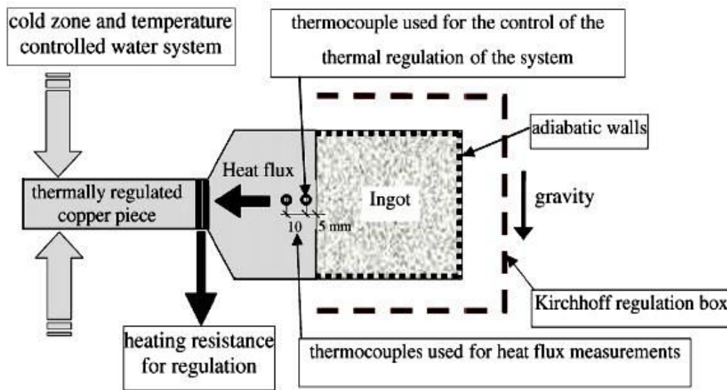
Figure III.4. Schéma illustratif de l'installation expérimentale AFRODITE-I, G. Quillet et al [5].
