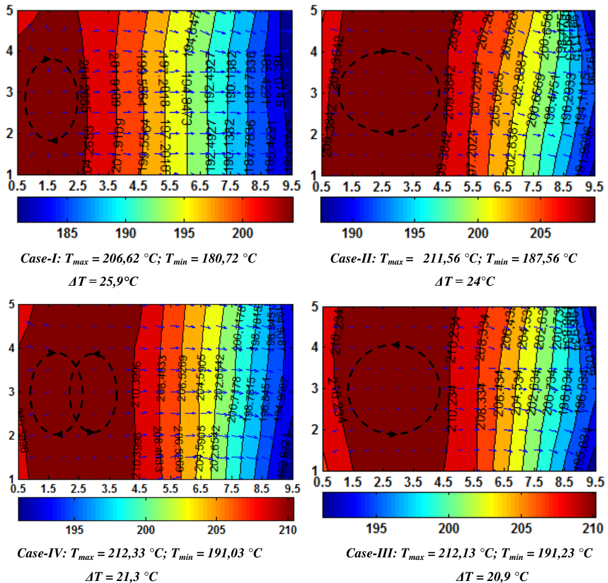
Figure V.18. Cartes de température couplées aux vecteurs des gradients thermiques locaux pour les quatre expériences de solidification (LH19, LH22, LH25 et LH29), à l'instant t_i = 24\text{mn} . Les conditions expérimentales sont: Sn-10wt.%Pb, \Delta T = 40\text{K} , CR = 0,03\text{K/s} , courant appliqué I = 8,2\text{A} .
