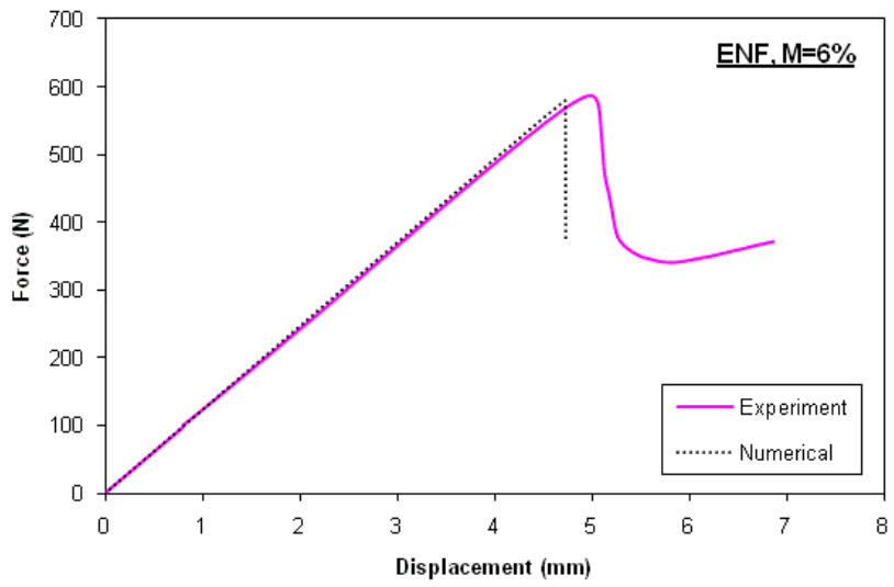
(b) ENF
