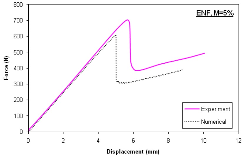
(b) ENF
