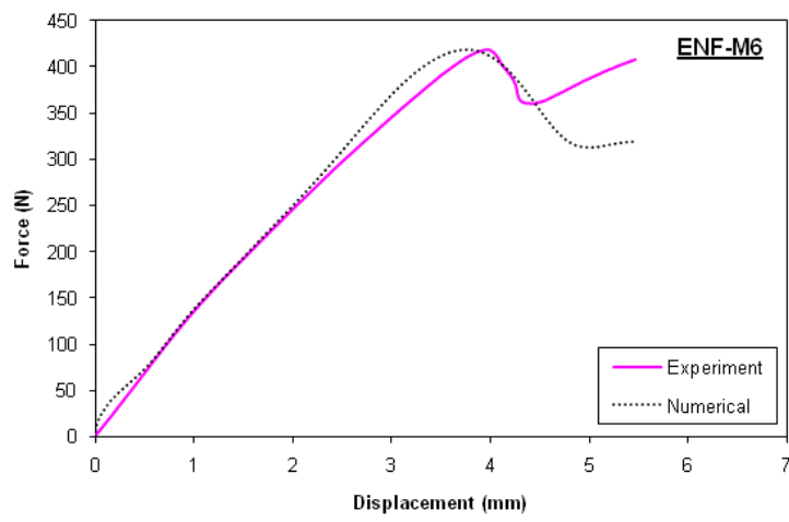
(b) ENF
