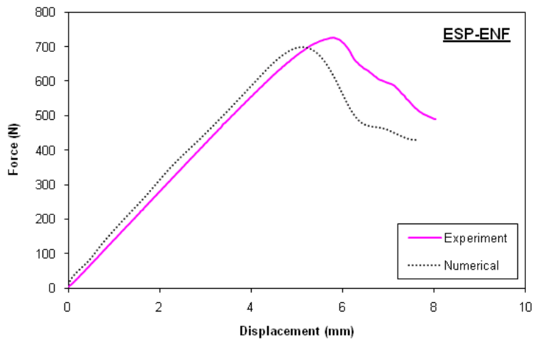
(b) ENF
