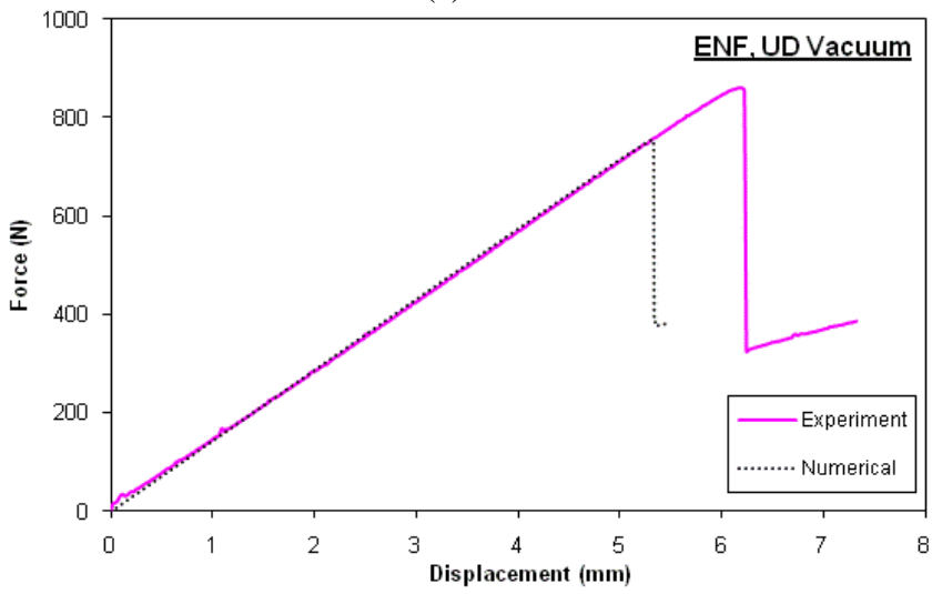
(b) ENF
