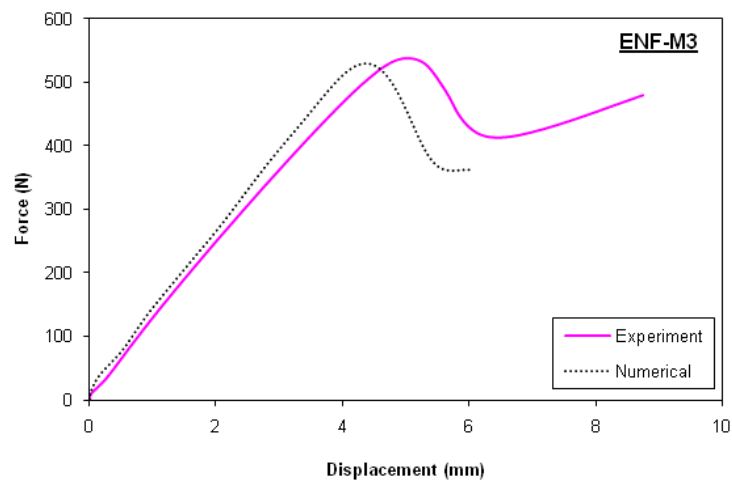
(b) ENF
