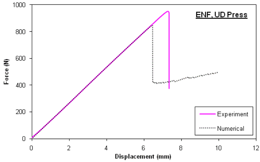
(b) ENF
