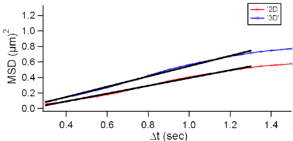
Figure 30: Comparaison du déplacement quadratique moyen (MSD) pour une bille fluorescente de 1\mu\text{m} en 2D (rouge) et en 3D (bleu). Les coefficients de diffusion sont de 0,46\mu\text{m}^2/\text{s} et 0,68\mu\text{m}^2/\text{s} respectivement.
