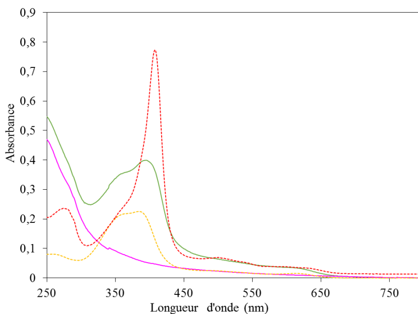
Figure 127. Spectres UV-visible de l'holo-myoglobine (rouge), de l'hème libre en solution (jaune), de l'hybride Mb-[Co(dm \text{gH} ) _2 (H _2 O) _2 ] (rose) et de l'hybride Mb-[Co(dm \text{gH} ) _2 (H _2 O) _2 ] en présence d'hème (vert) (à 10 \mu\text{M} dans du tampon Tris/HCl 50 mM pH 7.5 – spectres stables pendant au moins 4 h).
