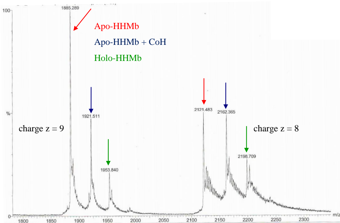
Figure 138. Spectre de masse ESI-TOF d'un échantillon de myoglobine de cheval incubé avec le complexe \text{Co}(\text{dmG})_2(\text{H}_2\text{O})_2 puis passé sur colonne d'exclusion stérique (24 \mu\text{M} dans l'acétate d'ammonium 50 mM pH 7). m/z=1885,289 , m=16961,58\text{Da} z=9 ; m/z=1921,511 m=17284,65\text{Da} z=9 ; m/z=1953,840 m=17578,74\text{Da} z=9 ; m/z=2121,483 m=16961,58\text{Da} z=8 ; m/z=2162,365 m=17284,65\text{Da} z=8 ; m/z=2198,709 m=17578,74\text{Da} z=8 .
