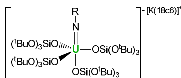
[K18c6][U(NR)(OSi(O t Bu) 3 ) 2 ]
