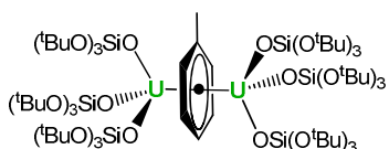
[U(OSi(O t Bu) 3 ) 2 ] 2 (μ-η 6 :η 6 -C 7 H 8 )
