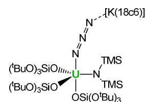
[K18c6][U(N 3 ){N(SiMe 3 ) 2 }(OSi(O t Bu) 3 ) 2 ]
