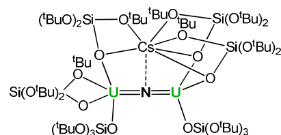
[Cs(μ-N){U(OSi(O t Bu) 3 ) 2 }] 2
