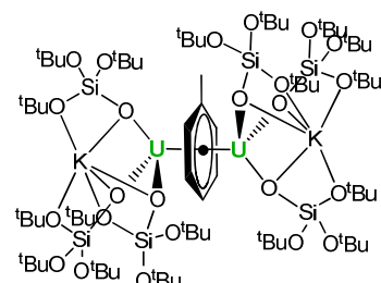
[K 2 {U(OSi(O t Bu) 3 ) 2 }] 2 (μ-η 6 :η 6 -C 7 H 8 )
