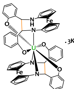
K_3[U(bis-salfen)(bis-Hsalfen)] 13-H
