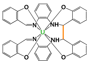
[U(bis-H_2salophen)] 9
