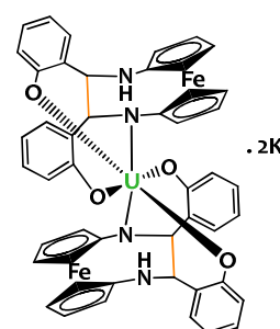
K_2[U(bis-Hsalfen)_2] 13-H 2
