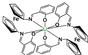
[U(salfen)_2] 12
