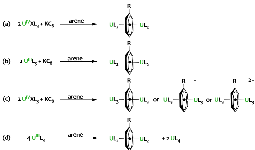
Scheme 1.35. Reported syntheses of uranium arene inverted sandwiches. (a) 74, 256 ; (b) 252 ; (c) 118, 253-255, 259 ; (d) 257 .
