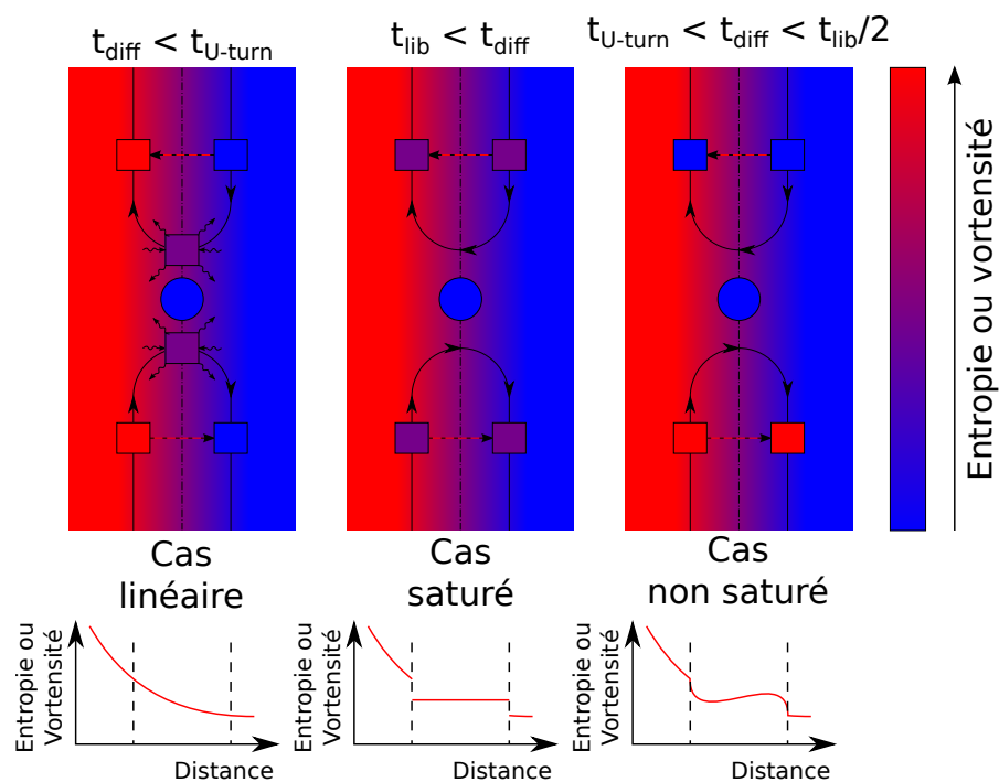
FIGURE 1.13 – Dans le référentiel tournant avec la planète, représentation du mécanisme général à l’origine du couple de corotation. Lorsque les temps de diffusion t_{diff} sont plus grands que le temps de libration t_{lib} , le couple de corotation sature car le gradient de vortensité/entropie au travers de la région fer-à-cheval tend à s’aplatir. Ce dernier est restauré quand les temps de diffusion t_{diff} sont plus courts que le temps de libration t_{lib} . Dans ce cas, la valeur optimale du couple de corotation est obtenue lorsque les temps de diffusion t_{diff} sont de l’ordre de la moitié du temps de libration t_{lib}/2 . Dans la limite où les temps de diffusion t_{diff} sont plus courts que le temps de demi-tour t_{U-turn} , l’amplitude du couple de corotation décroît pour atteindre la valeur prédite par une analyse linéaire.
