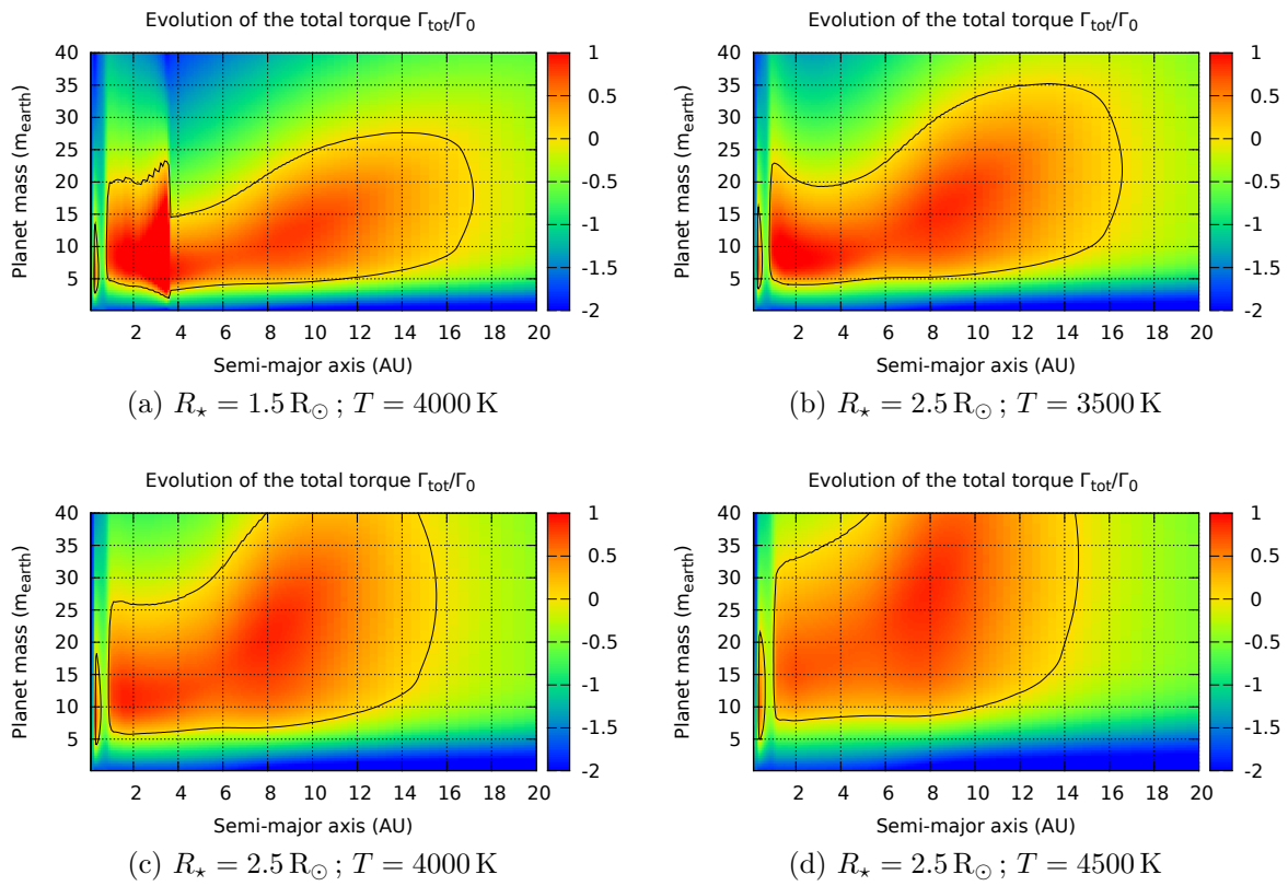
FIGURE 3.13 – Influence du rayon R_{\star} et de la température T_{\star} de l'étoile centrale sur la carte de migration au travers de l'irradiation. Les luminosités correspondantes pour les cartes (a), (b), (c) et (d) sont respectivement 0.5 L_{\odot} , 0.84 L_{\odot} , 1.43 L_{\odot} et 2.30 L_{\odot} . Tous les autres paramètres sont identiques au disque de référence [§ 3.1 page 78].
