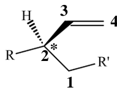
Figure I-18 : Atome de carbone asymétrique (numéro 2) dans une unité butadiène insérée en 1,2. R et R' sont des chaînes macromoléculaires.
