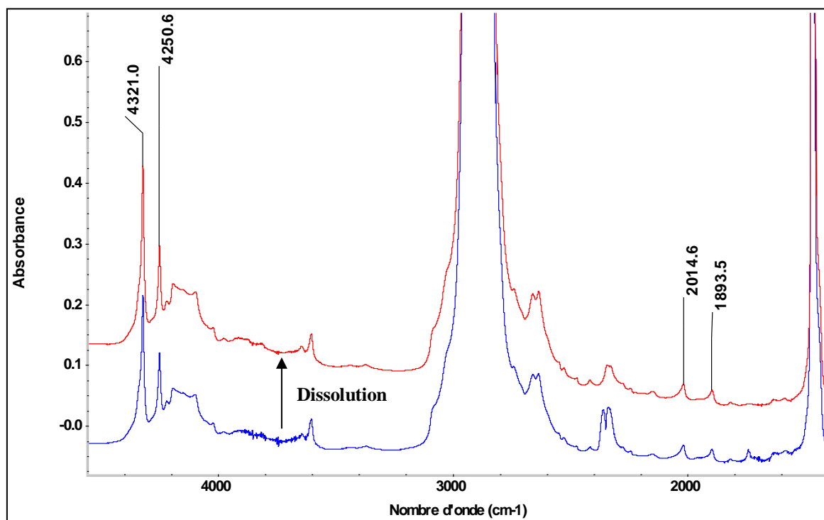
Figure III-20 : Spectres IRTF du PE ATO ® , région 1 500 – 4 500 \text{cm}^{-1} . En bas, spectre d'un échantillon mis en presse ; en haut, spectre d'un échantillon dissout, précipité, puis mis en presse.
