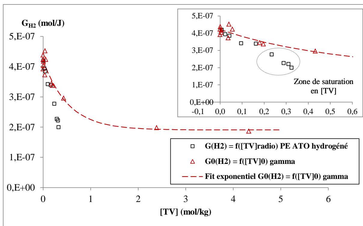
Figure IV-11 : En noir : évolution de G_{H_2} avec [TV]_{radio} pour le PE ATO hydrogéné. [TV]_{radio} calculée avec l'ajustement [TV](D) = [TV]_{sat} - ([TV]_{sat} - [TV]_0) * e^{-b*D} (IV-2). Conditions d'irradiation : électrons 1 MeV, atmosphère inerte He, température ambiante. En rouge : évolution de G_{H_2}(0) avec [TV]_0 (moyenne 75 kGy et 130 kGy). Conditions d'irradiation : photons gamma, atmosphère inerte He, température ambiante. Ajustement exponentiel d'après l'équation (IV-3) avec G_{H_2,D \rightarrow 0,Min} = 1,90 \cdot 10^{-7} mol/J , G_{H_2,D \rightarrow 0,Max} = 4,21 \cdot 10^{-7} mol/J , \beta = 1,9021 kg/mol .
