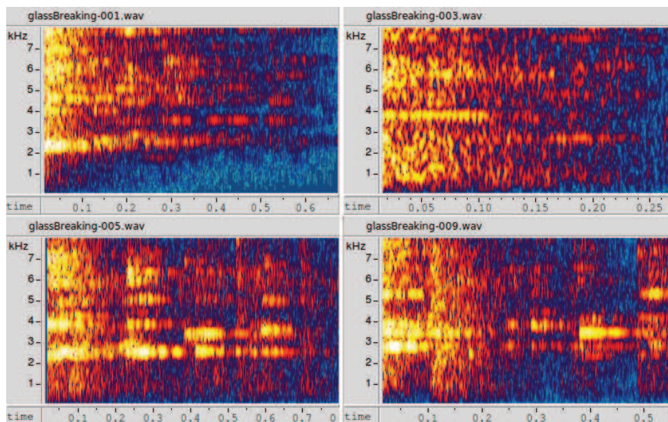
Figure 5.5: Spectrogrammes de bris de glace
