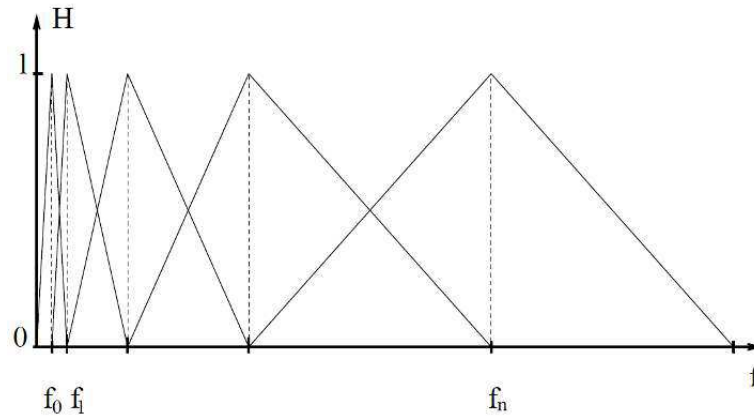
Figure 2.5: Filtres en fréquences de Mel
