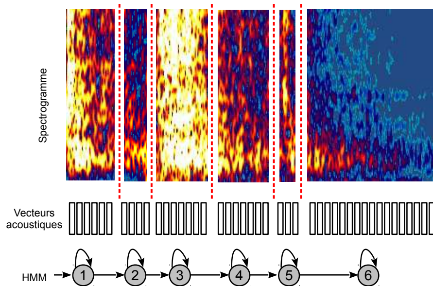
Figure 3.4: Spectrogram d'un claquement de porte et HMM correspondant à l'évolution temporelle
