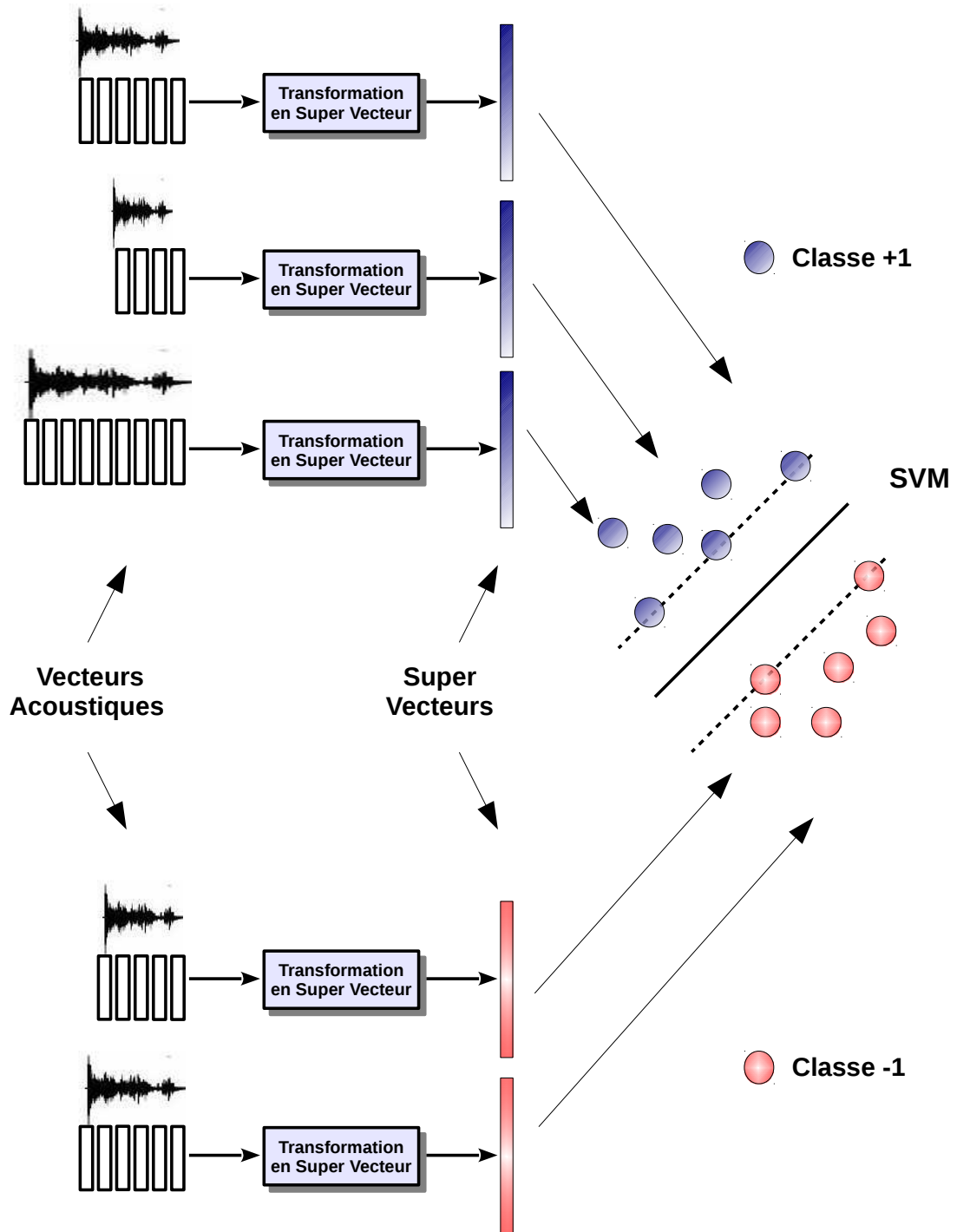
Figure 4.3: Des vecteurs acoustiques au super vecteurs SVM
