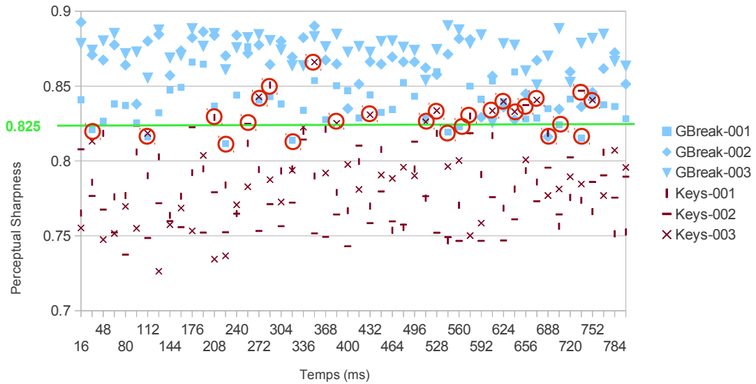
Figure 5.13: Une possible séparation linéaire entre les fenêtres des deux classes GlassBreaking et Keys en se basant sur le coefficient Perceptual Sharpness
