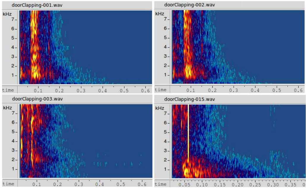
Figure 5.2: Spectrogrammes de claquements de porte
