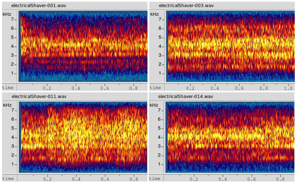
Figure 5.3: Spectrogrammes de bruits de moteur électrique (rasoir)
