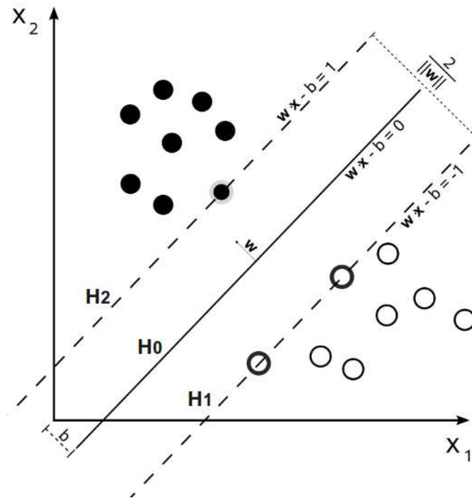
Figure 2.9: Exemple d'un classifieur linéaire.
