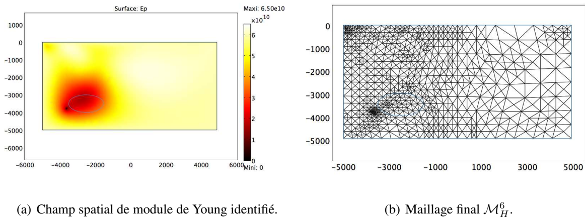
Figure 2.2 – Résultat de la stratégie de détection de cavité après 6 étapes de raffinement (cas 2D) [Puel et Aubry 2011].
