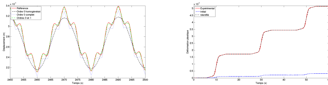
(a) Déplacement en x = L pour différentes estimations homogénéisées du problème direct.
