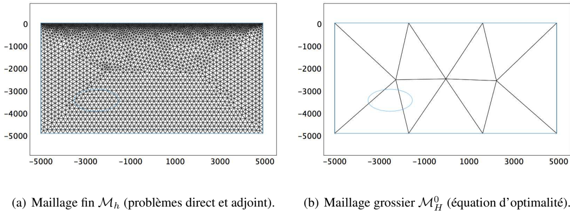
Figure 2.1 – Maillages utilisés pour la stratégie de détection de cavité (cas 2D) [Puel et Aubry 2011].
