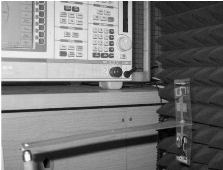
Figure 4.22 - Mesure de l'impédance des prototypes HO-01 avec l'Analyseur de Réseau Vectoriel ZVB8 de Rohde & Schwarz
