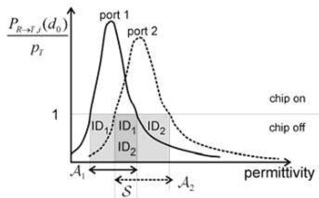
Figure 6.9 - Ensembles d'activation et gamme de détection d'un tag RFID à deux-ports en mode détection analogique
