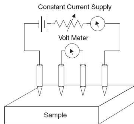
Figure 3.10 – Mesure de la résistivité de la couche métallique par sonde 4 pointes
