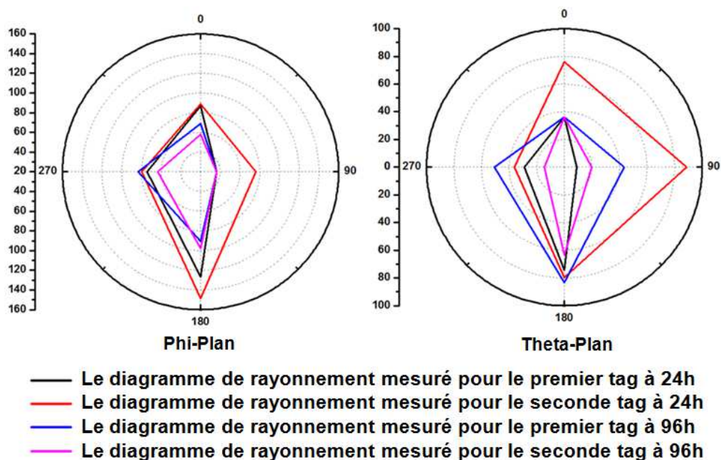
Figure 6.37 - Les diagrammes de rayonnement mesurés pour la conception To-2 sur Phi-Plan (à gauche) et Theta-Plan (à droite)
