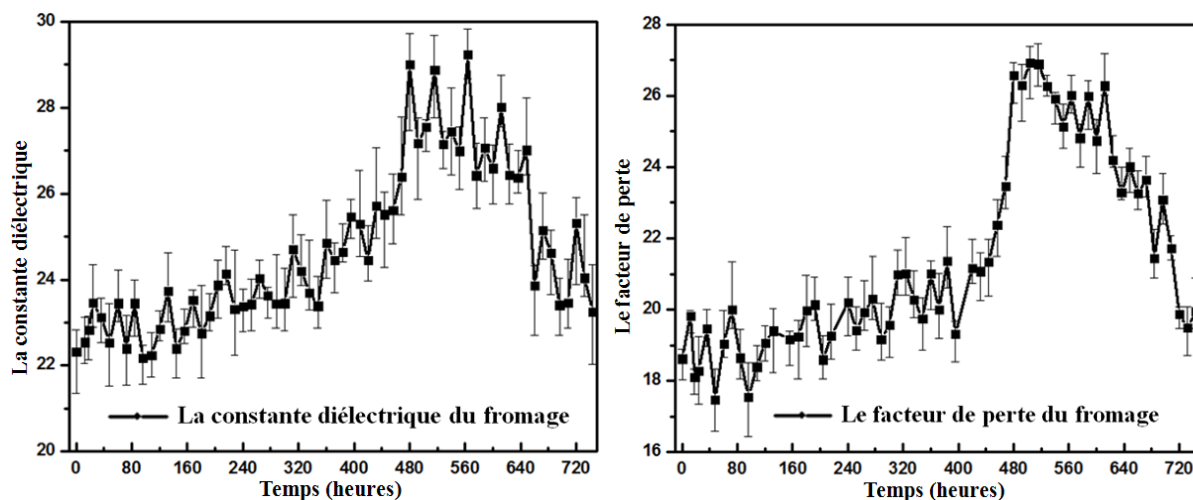
Figure 5.26 - La permittivité du fromage Cheddar en fonction du temps
