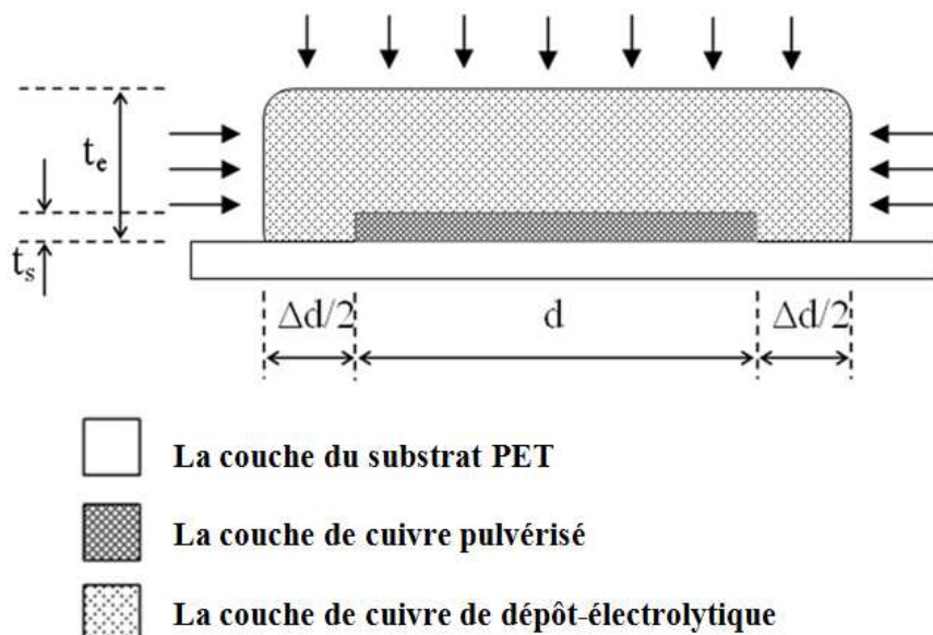
Figure 4.12 – Elargissement des motifs pendant le dépôt électrolytique
