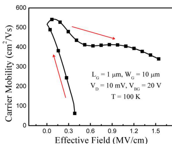
Fig. 11: Mobilité en fonction du champ électrique effectif. La grille arrière est polarisée en inversion ( V_{BG} = +20V ) et le canal avant s'ouvre graduellement.
