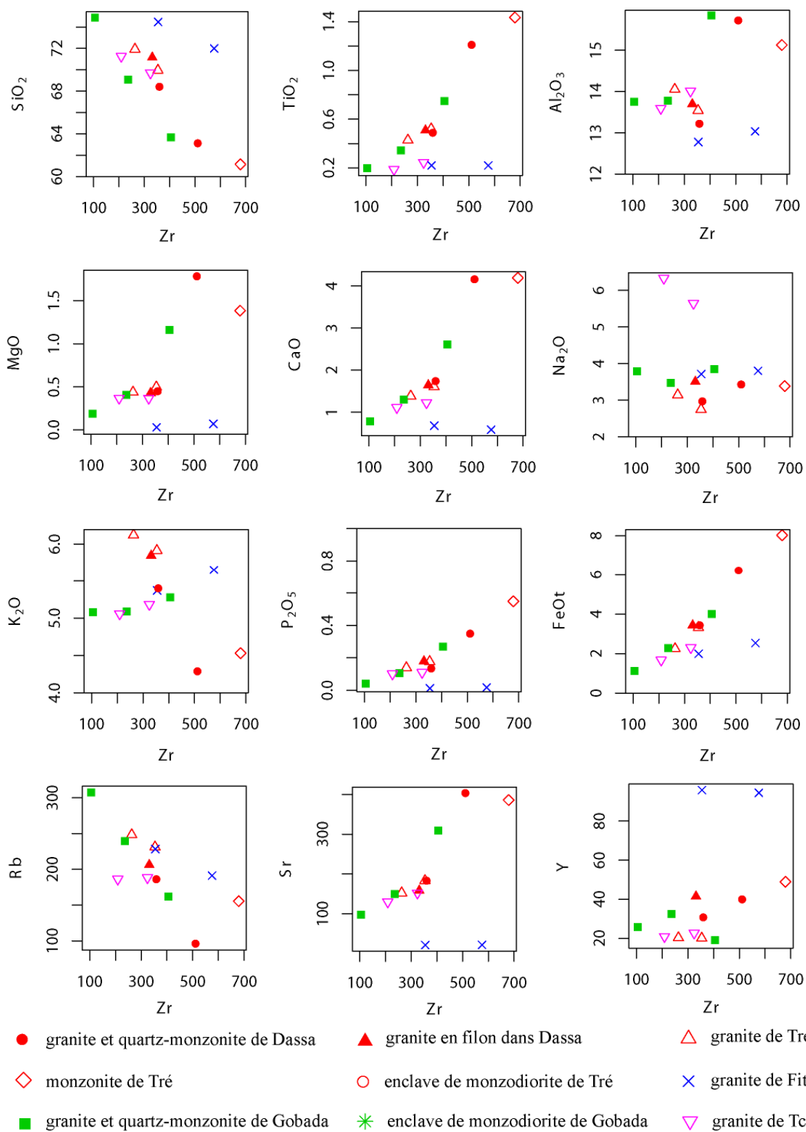
Figure V.4. Diagrammes Zr vs. éléments des granitoïdes de Dassa, Tré, Gobada, Tchetti et Fita.
