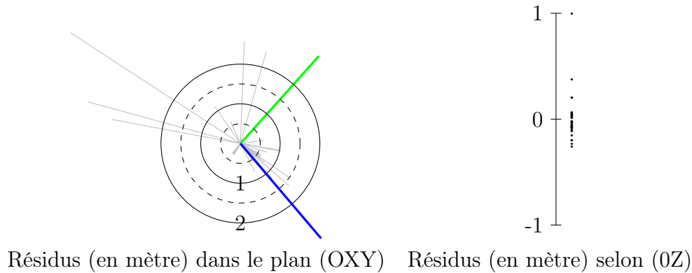
FIGURE 9.3 – Résidus 3D après recalage 3D/3D sur l'exemple (b).
