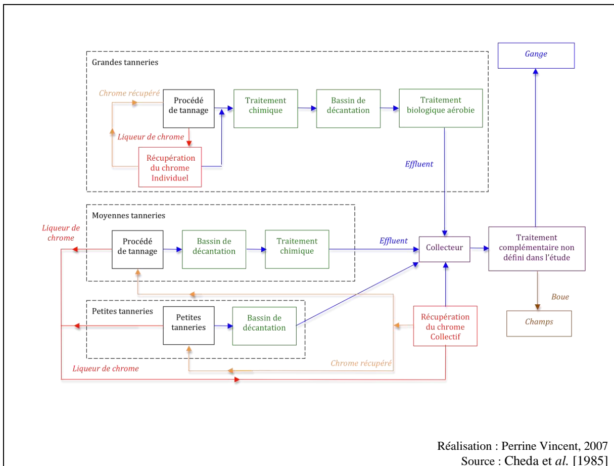
Schéma 3 – dispositif de traitement des eaux de tanneries de Jajmau proposé par Cheda et al. [1985]
