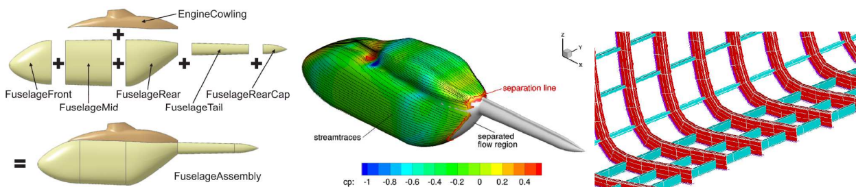
Figure 1.22: Ces captures d'écran proviennent de la référence [4]. La figure de gauche montre les différents éléments génériques du fuselage et assemblés de manière automatique. La figure au centre montre l'exploitation de la géométrie créée dans le logiciel VSAERO. Enfin, la figure de droite montre la génération d'une structure à l'aide d'éléments finis de type poutres...
