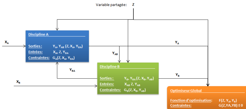
Figure 1.24: Cette figure présente un exemple de schéma d'optimisation multidisciplinaire avec des entrées propres à chaque discipline X_i , des variables partagées Z , des sorties multidisciplinaires Y_{i,j} , des sorties monodisciplinaires Y_i ainsi qu'une fonction d'optimisation du système F .
