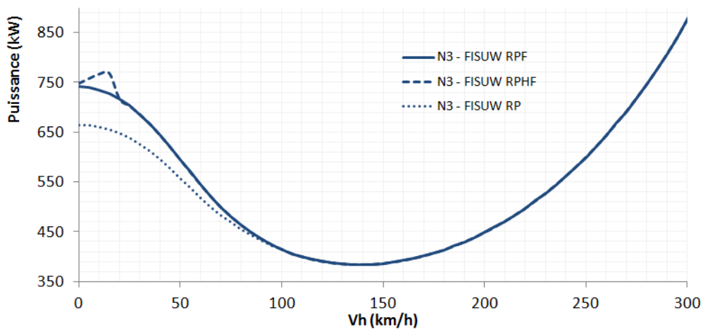
Figure 2.42: Comparaison entre deux modèles : FISUW avec et sans l'interaction sur l'empennage horizontal noté par la lettre H dans le terme RPHF.
