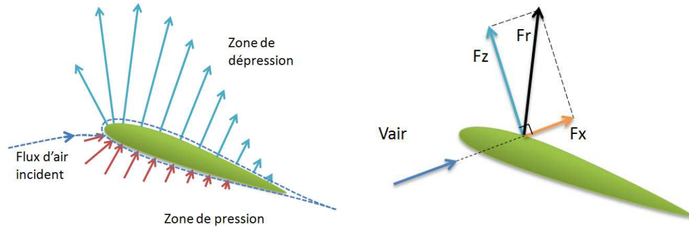
Figure 1.3: A gauche, schéma des zones de pression (en rouge) et de dépression (en bleu) créées par la circulation d'un fluide autour d'un profil de pale. A droite, schéma des forces générées par les zones de pression / dépression causé par le flux d'air incident V_{air} . Les forces représentées sont : F_z la force de portance, F_x la force de traînée et F_r , la force résultante.
