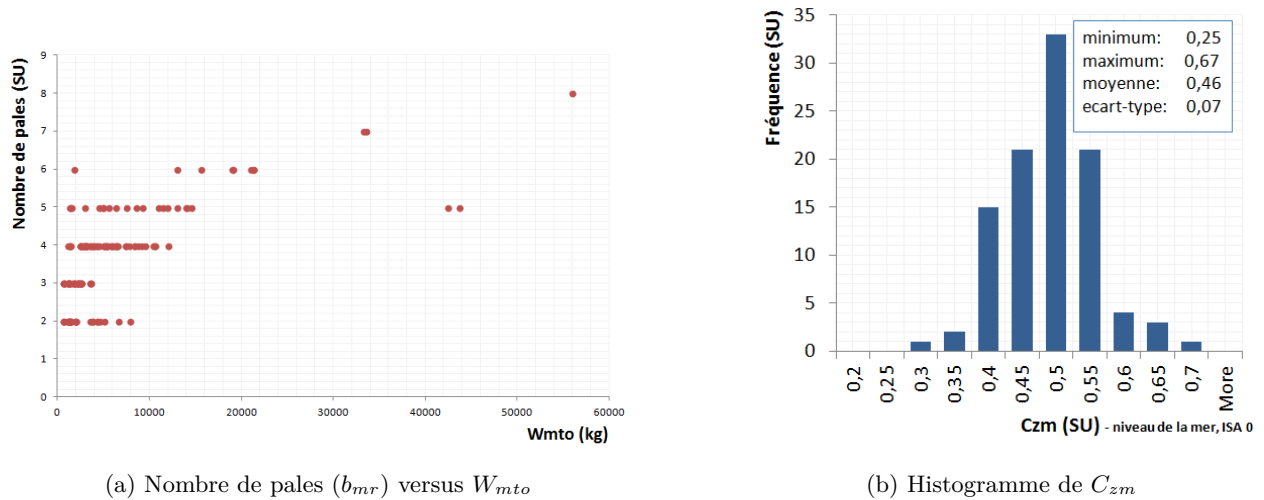
Figure 2.10: Exploitation de la base de données pour déterminer le nombre de pales.
