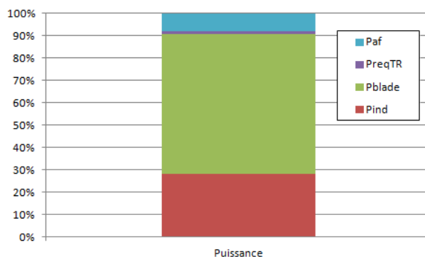
Figure 3.29: Comparaison des contributions de la puissance requise totale à 280 km/h pour un HO-90 du front de Pareto.
