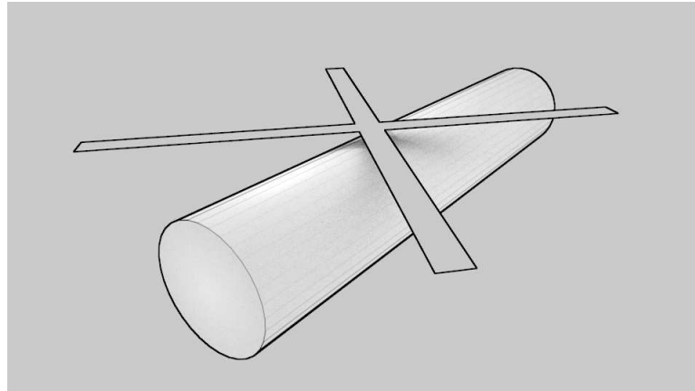
Figure 2.31: Géométrie considérée au niveau 1 et vue par le module aérodynamique.
