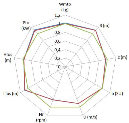
Figure 2.15: Résultats de la chaîne de calcul de niveau 0 pour le Dauphin SA 365N.
