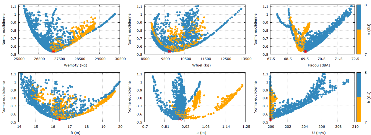
Figure 3.36: Diagrammes de niveaux en fonction des objectifs (ligne du haut) et des variables (lignes du bas). La norme euclidienne est utilisée.
