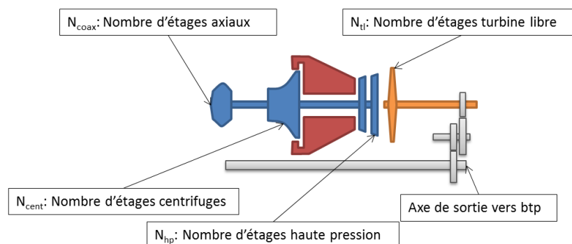
Figure 2.30: Exemple d'architecture d'une turbine considérée dans le module génération de puissance.
