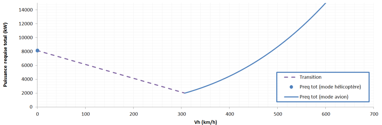
Figure 4.2: Bilan de puissance typique d'un convertible.
