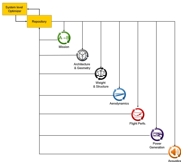
Figure 1.25: Méthode All At Once adaptée à un problème traité dans cette thèse et présentée dans [8]. Les disciplines sont découplées et ne communiquent qu'à travers une banque de données de variables : le « repository ». Seul ce dernier est lié à l'algorithme d'optimisation.
