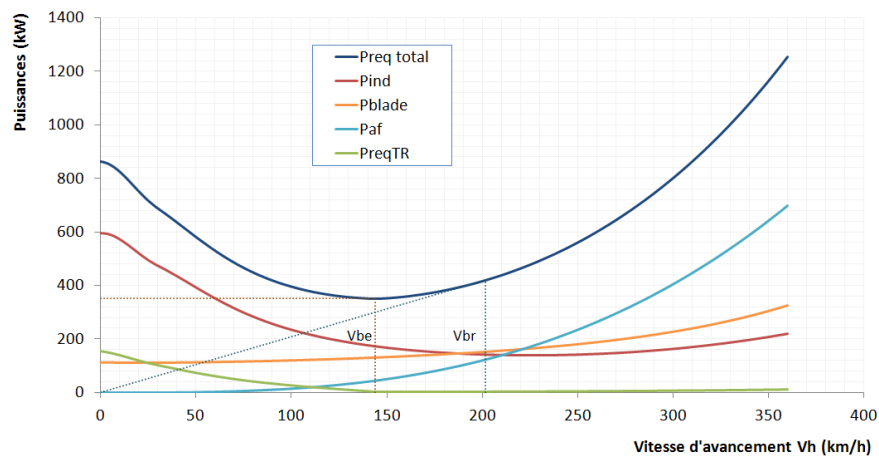
Figure 2.25: Variations des différentes puissances en fonction de V_h .
