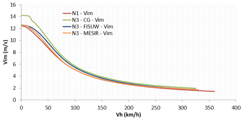
Figure 2.40: Comparaison des vitesses induites en fonction de la vitesse horizontale, V_h , pour différents modèles de niveau 3 et un modèle de niveau 1.
