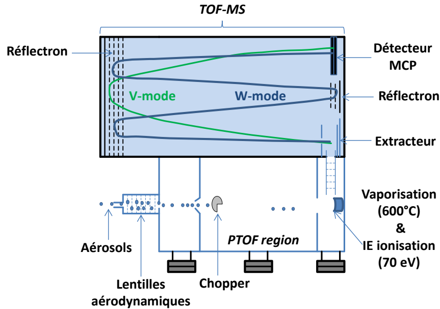
Figure II-15 : Schéma de l'HR-TOF-AMS (d'après DeCarlo et al., 2006).
