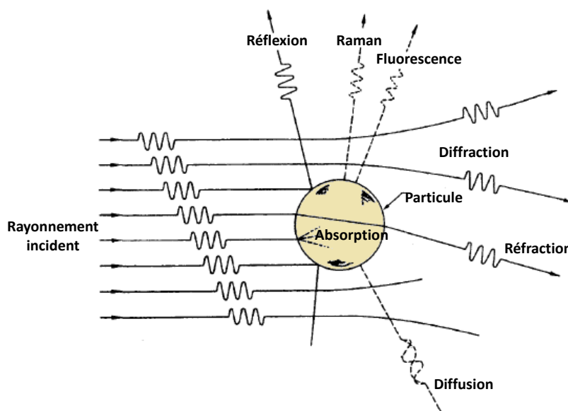
Figure I-2 : Mécanismes d'interaction entre une particule et une radiation incidente (d'après Seinfeld et Pandis, 2006).
