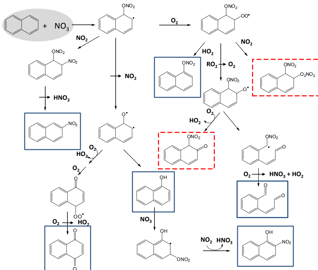
Figure IV-11: Mécanisme proposé pour l'oxydation du naphthalène en présence de radicaux nitrates (les carrés bleus représentent les produits identifiés par PTR-TOF-MS et les carrés rouges en pointillés ceux mis en évidence uniquement par FTIR).
