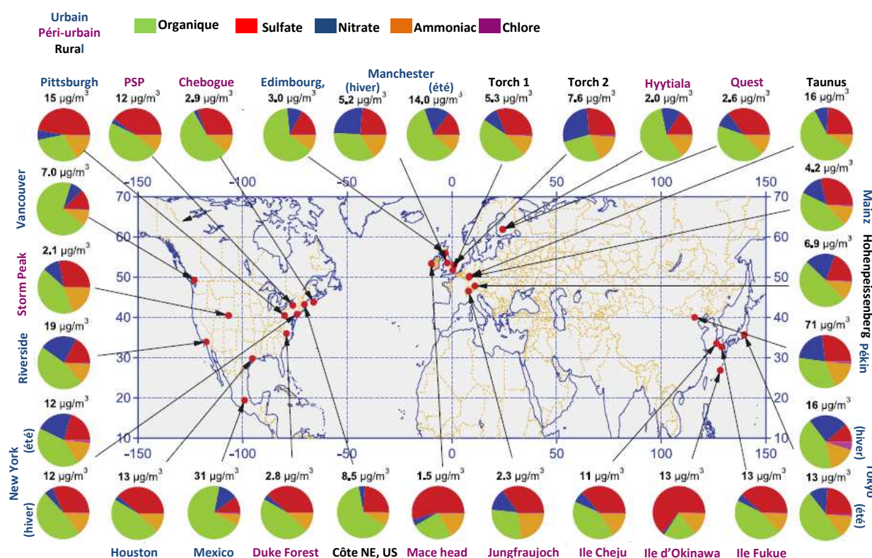
Figure I-3 : Caractérisation en masse de PM_1 (particules de diamètre aérodynamique inférieur à 1\mu m ) dans de nombreuses atmosphères à l'aide d'un AMS (spectromètre de masse à aérosols) (Zhang et al., 2007).
