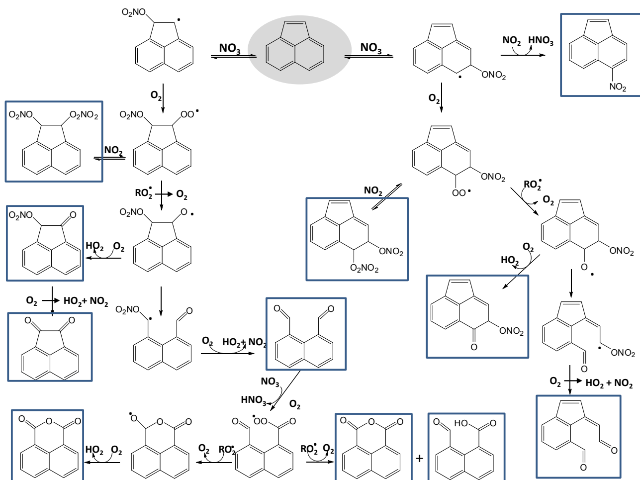
Figure IV-12 : Mécanisme proposé pour décrire l'oxydation de l'acénaphthylène initiée par le radical nitrate (les produits encadrés en bleu sont les composés identifiés dans ce travail).
