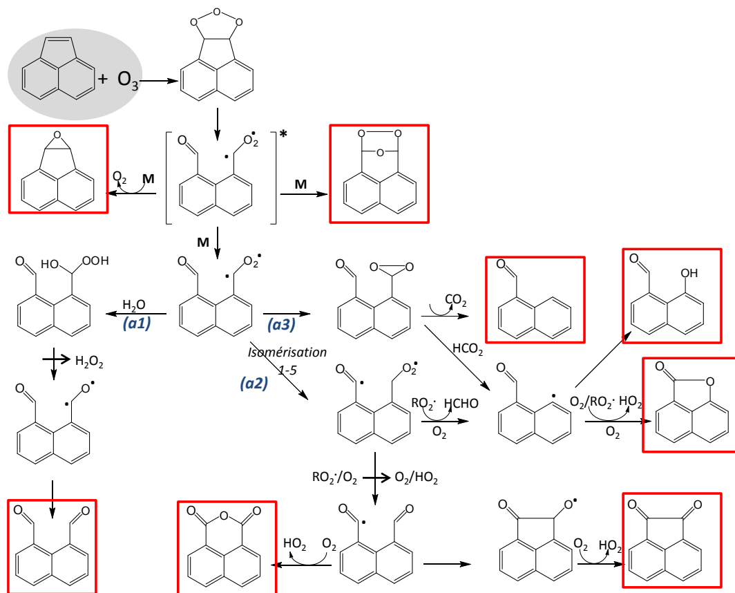
Figure IV-8 : Mécanisme proposé pour la réaction de l'acénaphthylène avec l'ozone.
