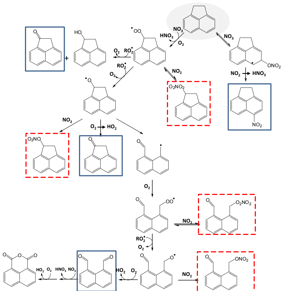
Figure IV-13 : Mécanisme proposé pour la réaction de l'acénaphthène avec le radical nitrate (les produits encadrés en bleu et en pointillés en rouge correspondent aux produits identifiés par PTR-TOF-MS et FTIR respectivement).
