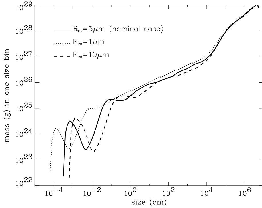
FIGURE 2.3: Exemples de distributions de la masse totale des grains résultant de l'évolution dynamique et collisionnelle d'un disque de débris massif ( M = 0.1M_{\oplus} pour a < 1 cm) après 10^7 années (Thébault & Augereau 2007). Plusieurs masses stellaires sont testées correspondant à autant de tailles d'éjection, notées ici R_{\text{PR}} ( M_{\star} = 1.7, 2.1, 2.5 M_{\odot} )
