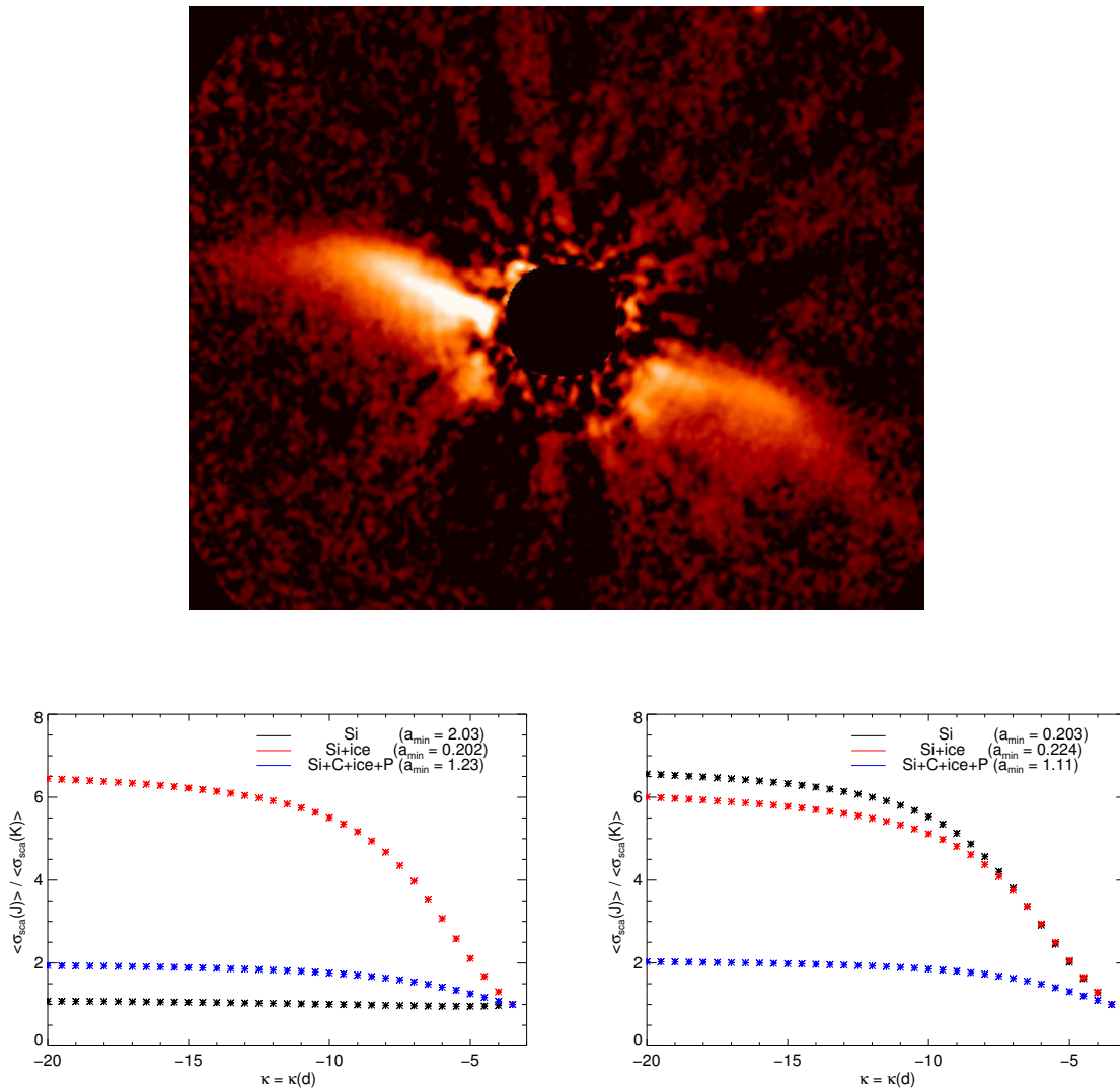
FIGURE 6.2: En haut : Le disque de HD 61005 imagé en bande K par le VLT/NaCo et traité avec l'algorithme LOCI corrigé des effets de l'auto-soustraction (E. Buenzli).
