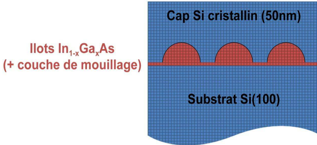
Figure IV.3.11: Représentation en coupe transverse de la structure des échantillons comportant un plan d'îlots d' \text{In}_{1-x}\text{Ga}_x\text{As} encapsulés par du Si cristallin d'abord à Tc (20 nm) puis avec une rampe de température 400-600°C (30nm).
