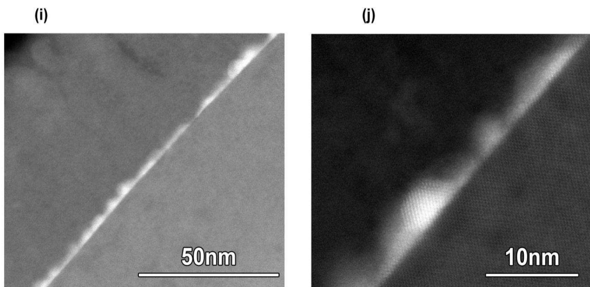
Figure III.3.22: Images TEM montrant des îlots d' \text{In}_{1-x}\text{Ga}_x\text{As} avec des teneurs x en Ga de : x=10\% (a et b), x=20\% (c et d), x=30\% (e et f), x=40\% (g et h), x=50\% (i et j), épitaxiés dans des conditions standard ( T_c=350^\circ\text{C} , rapport V/III=20) et encapsulés par du Si:a à 250^\circ\text{C} .
