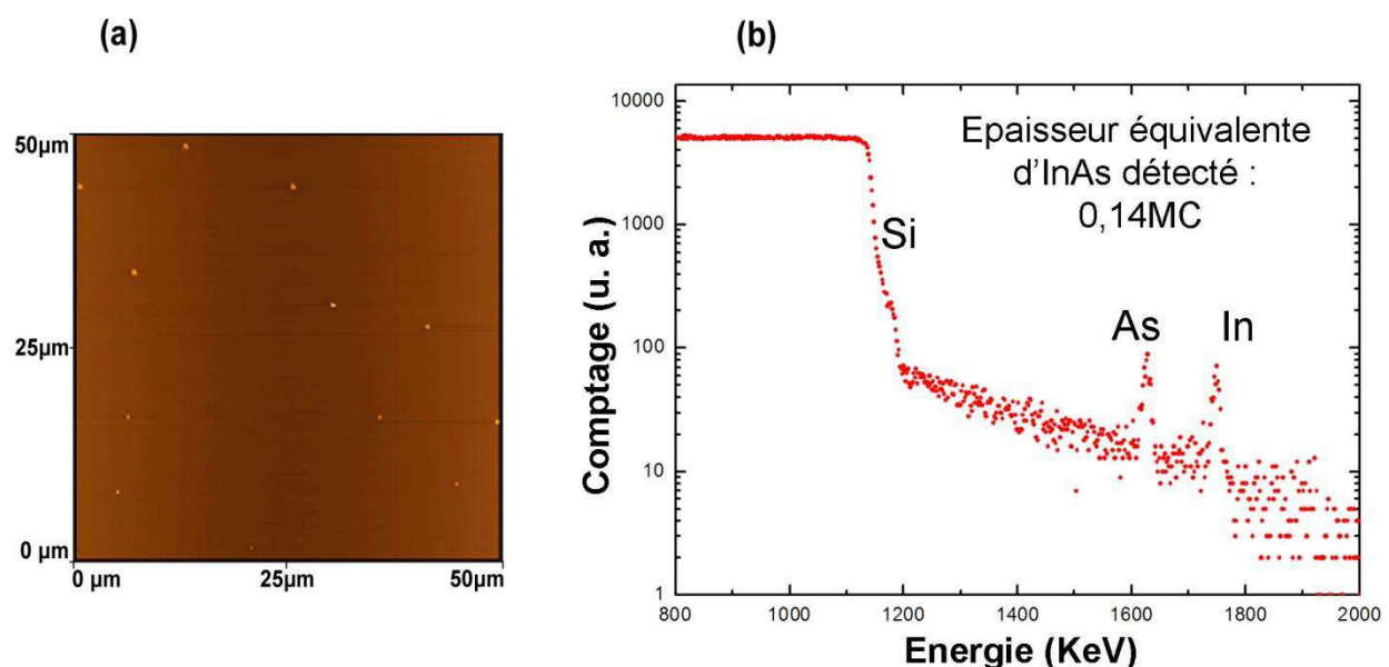
Figure III.3.6: Image AFM (a) et spectre RBS (b) d'un échantillon d'InAs épitaxié à T_C=530^\circ C (dépôt de 10 MC).
