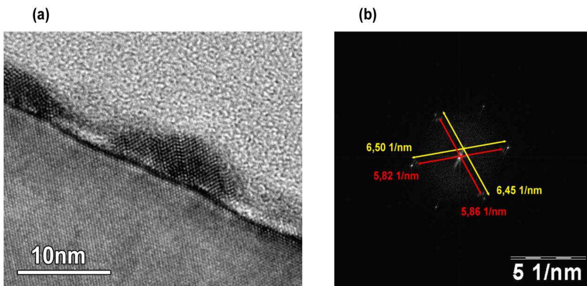
Figure III.3.20: Image TEM en coupe transversale (a) et transformée de Fourier (b) d'un îlot d'InAs épitaxié dans les conditions standard ( T_C=420^\circ\text{C} , V/III=20 ).
