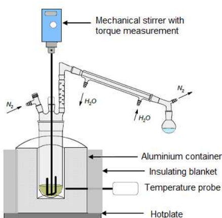
FIGURE 3 – Montage pour la synthèse des polyphthalamides
