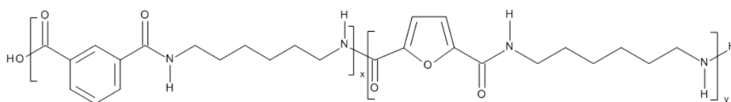
FIGURE 7 – Formule générale des copolyphthalamides PA 6-I (x) /6-F (y)
