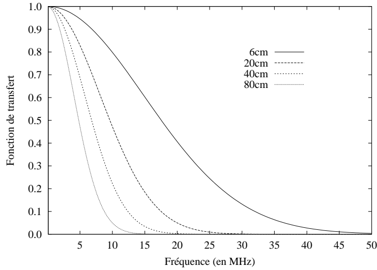
FIG. 2.13 – Module de la fonction de transfert normalisée de l'atténuation dans l'eau donnée pour plusieurs distance d'observation du transducteur, pour K = 3.75 \cdot 10^{-14} \text{dB.m}^{-1}.\text{Hz}^{-2} .
