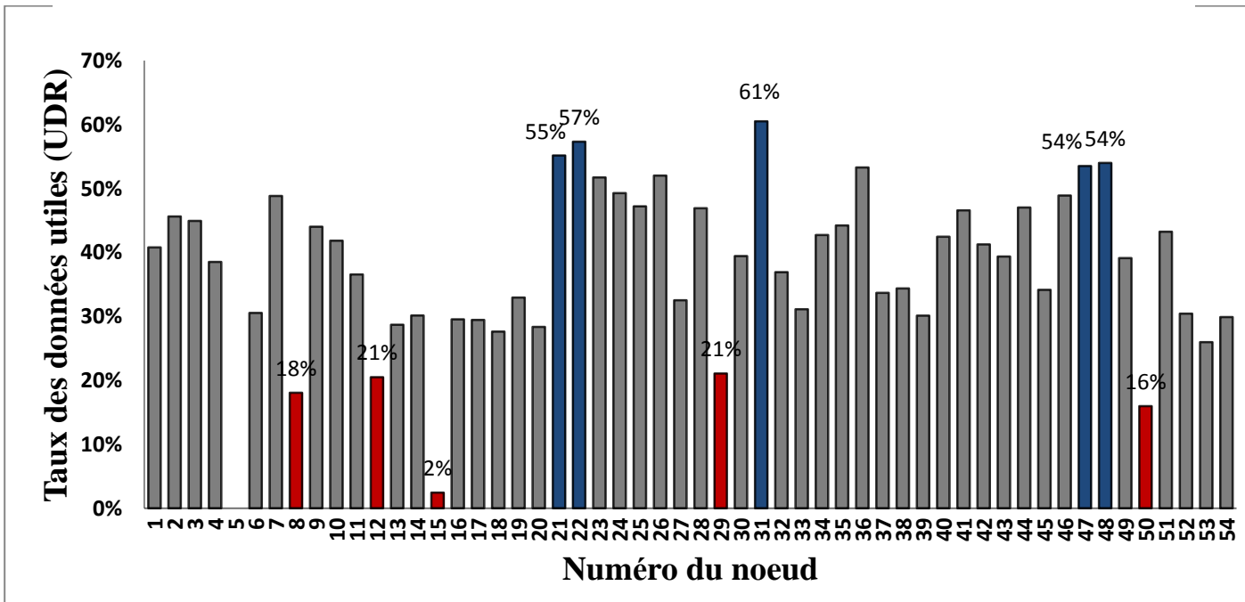
Figure 3-8 : Les deux capteurs 26 et 31 rapportent des valeurs erronées (voltage < 2.3)
