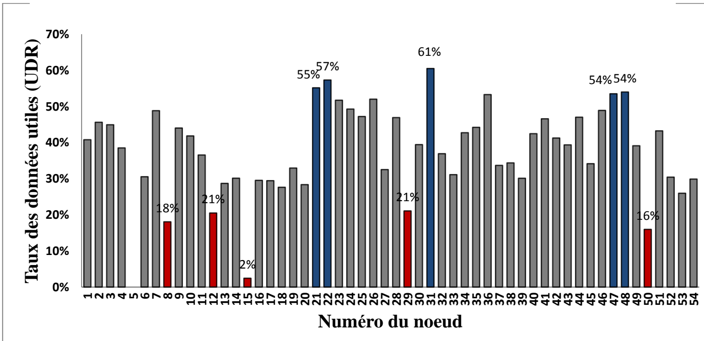
Figure 3-8 : Les deux capteurs 26 et 31 rapportent des valeurs erronées (voltage < 2.3)
