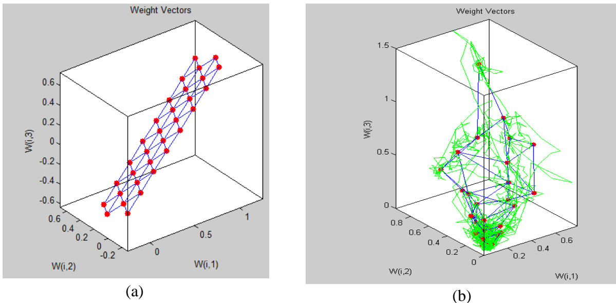
Figure 3-12 - Topologie hexagonale de 32 neurones en dimension 3 : (a) la carte avant l'apprentissage - (b) la carte après la convergence avec la distribution des données.
