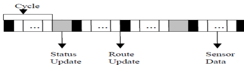
Figure 2-15: Allocation d'un créneau dans les réseaux de capteurs sans fils [85]
