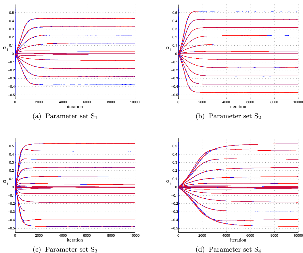
FIGURE A.7 – Convergence des coefficients pour NNLSM traitant le problème régularisé avec la norm- \ell_1
