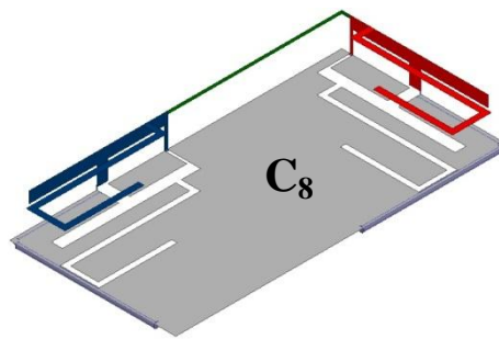
Géométrie du système multi-antennaire C_8
