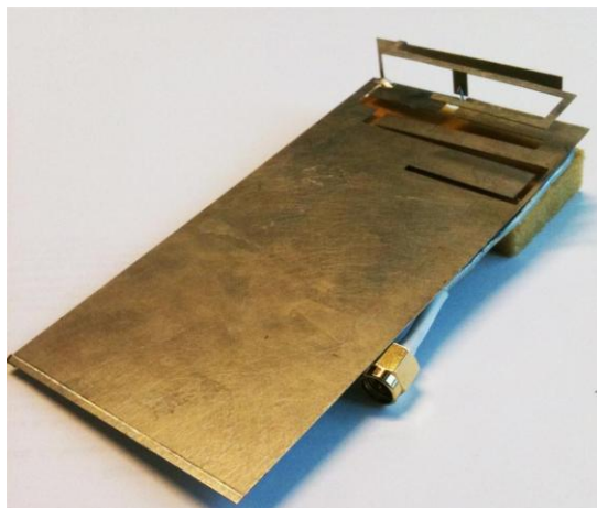
Prototype IFLA-AC réalisé sur du métal
