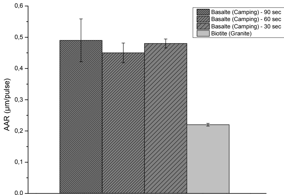
Figure IV-21. AAR des différentes minéralogies/mesures. A comparer avec la Figure VI-18.
