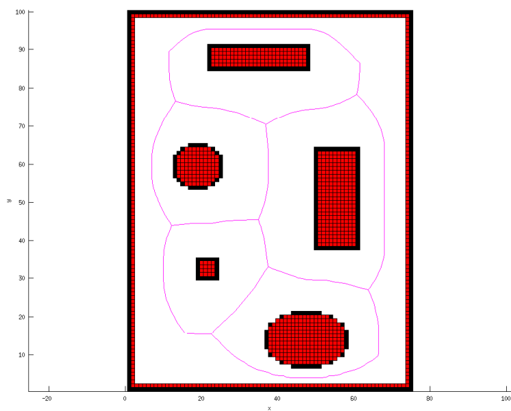
FIGURE 2.8 – Exemple d'un graphe de Voronoï.
