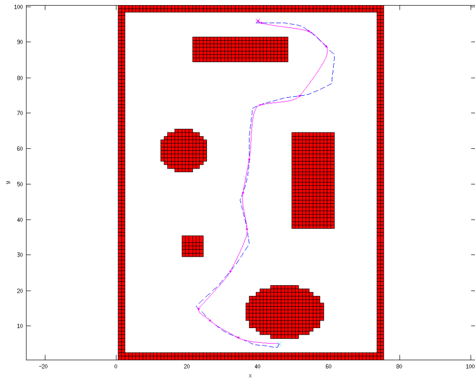
FIGURE 2.11 – Recherche d'une trajectoire optimale, en terme de longueur et de courbure, avec un temps final libre dans un espace contraint.
