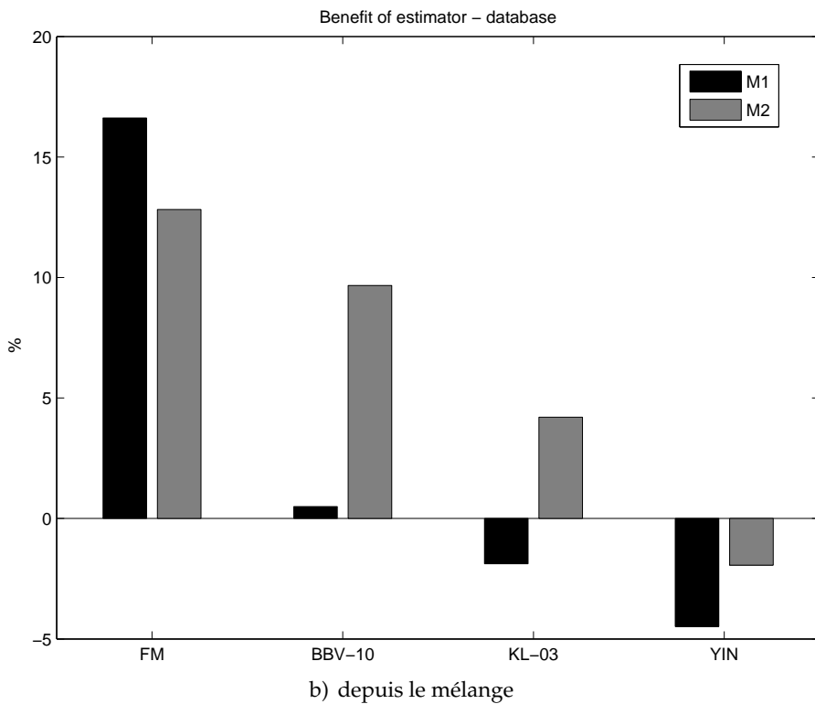
FIGURE 5.18 – Comparaison du gain en pourcentage de nombre de bits apporté par l'utilisation d'un estimateur. Les résultats sont triés par ordre décroissant du pourcentage de gain sur M2.
