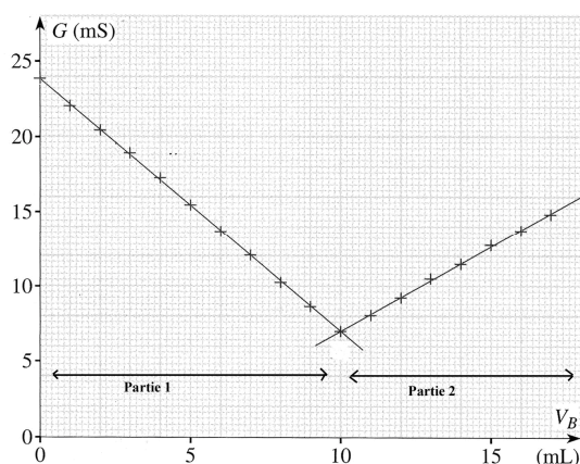
Figure 3 – Représentation graphique de la conductance en fonction du volume de solution d'hydroxyde de sodium versé
