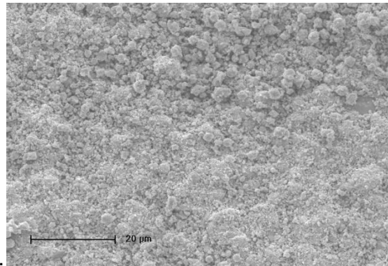
Figure 3-34 : Image MEB de la surface d'une bille de FAU [NaX] sans liant (Jean Daou, UHA)
