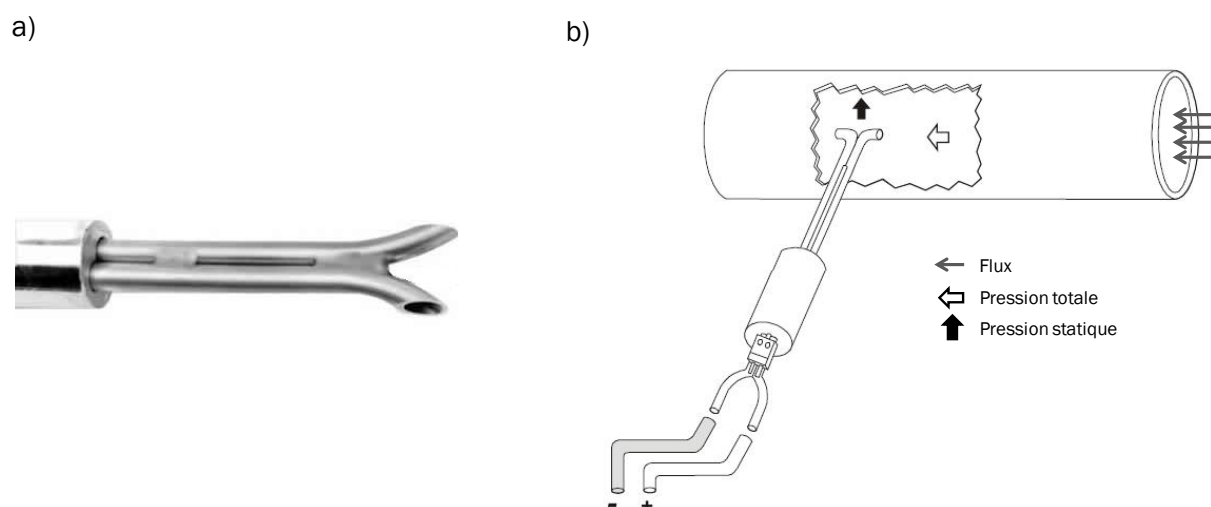
Figure 5-21 : Tube de Pitot S a) embout du tube de Pitot, b) schéma de principe
