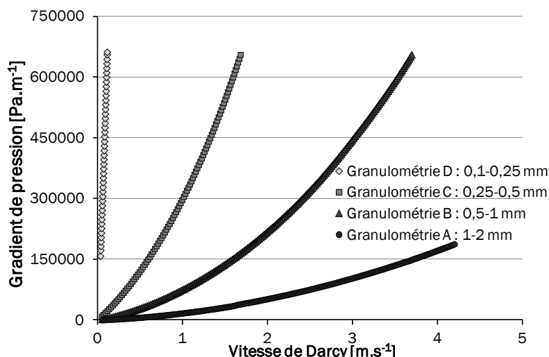
Figure 3-26 : Gradients de pression pour différentes granulométrie de zéolithe MFI [silicalite-1]
