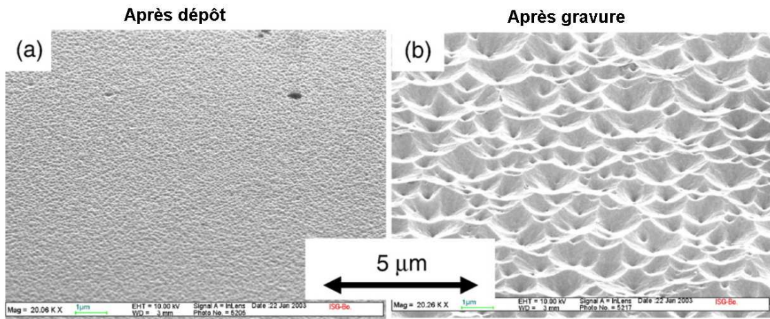
FIGURE 1.21 – Photos MEB d'une couche de ZnO:Al (a) avant gravure ; (b) après gravure par une solution d'acide chlorhydrique à 0,5 % (d'après [67])
