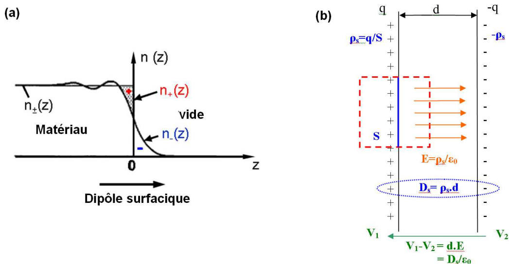
FIGURE 1.22 – (a) Formation d’un dipôle de surface par les électrons périphériques ; n(z) désigne la densité électronique (d’après [78]) (b) Lien quantitatif entre la densité surfacique de dipôle D_s et la différence de potentiel induite.
