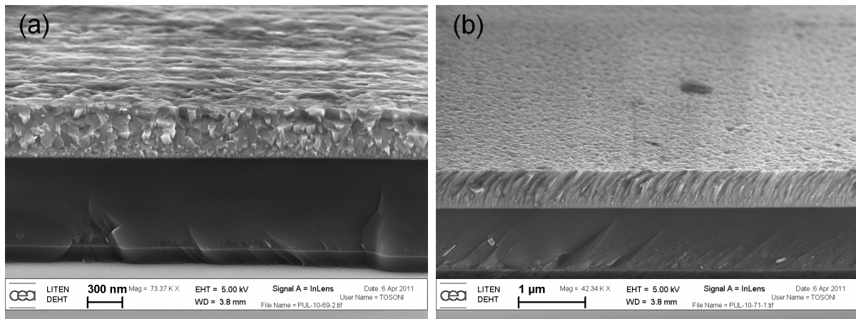
FIGURE 2.7 – Photos MEB de couches d'AZO déposées à (a) 150°C et (b) à 400°C
