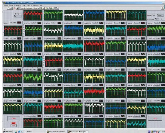
FIGURE 2.27. – Interface du programme d’acquisition montrant les 60 voies. Les signaux ont été acquis avec une fréquence d’échantillonnage de 1 kHz.
