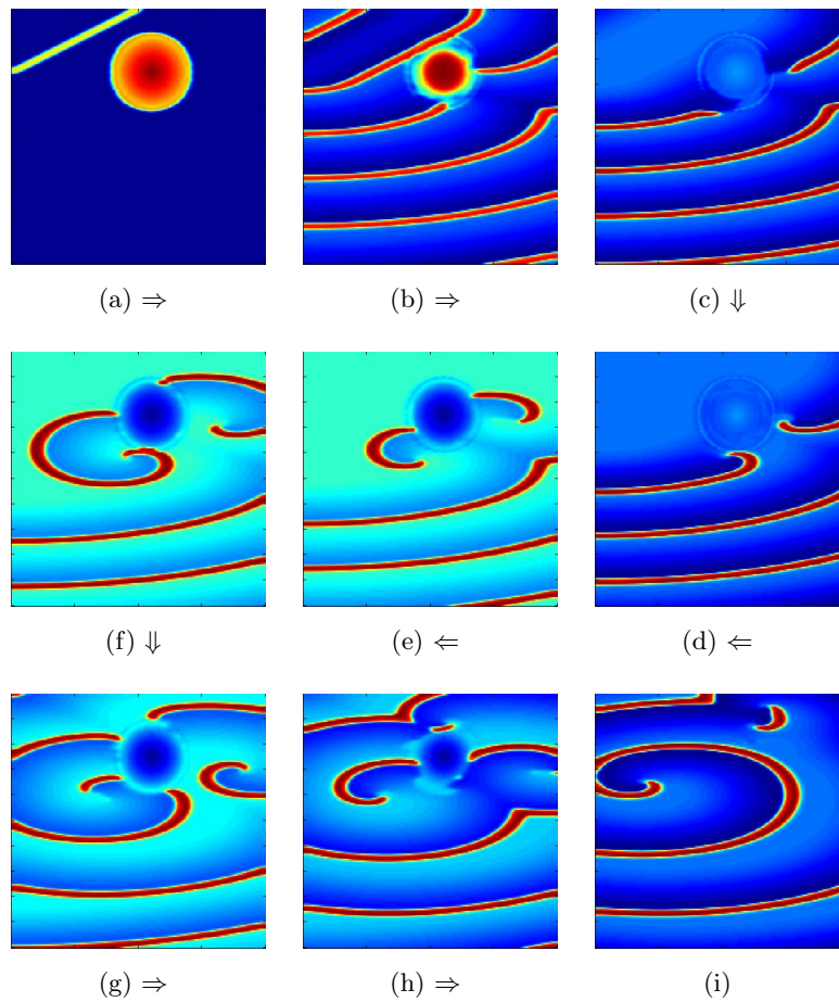
FIGURE 3.1. – Génération d'ondes spirales par la stimulation électrique dans un tissu légèrement arythmique. (a) : la source d'ondes planaires et la zone de stimulation ; (b) ⇒ (c) : la propagation d'ondes planaires ; (d) ⇒ (i) : la génération et l'évolution des ondes spirales. La couleur rouge indique la dépolarisation des cellules et la couleur bleue indique leur période réfractaire.
