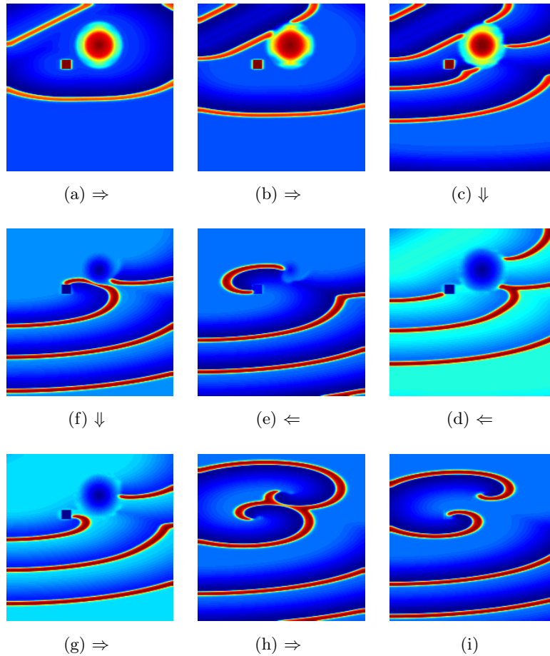
FIGURE 3.3. – Génération d'ondes spirales par la stimulation électrique dans un tissu ayant des obstacles : (a) : la source d'ondes planaires, zone de stimulation et un obstacle rectangulaire ; (b) \Rightarrow (c) : la propagation d'ondes planaires ; (d) \Rightarrow (i) : la génération et l'évolution d'ondes spirales. La couleur rouge indique la dépolarisation des cellules et la couleur bleue indique leur période réfractaire.
