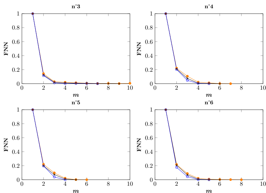
FIGURE 4.29. – Estimation de dimension d’immersion m par FNN, signaux arithmétiques.
