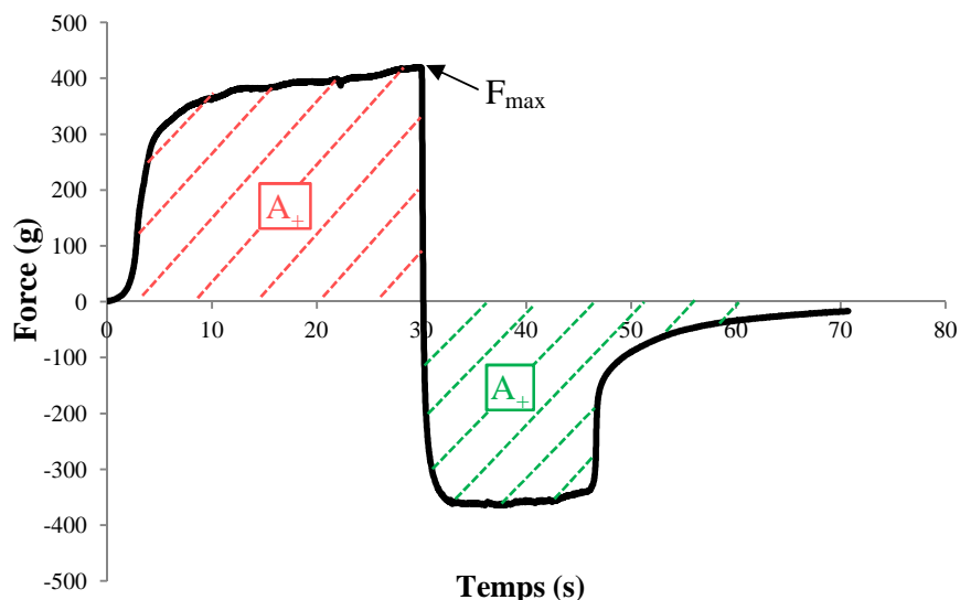
Figure 39. Représentation d'une courbe type d'extrusion obtenue avec les différents paramètres relevés
