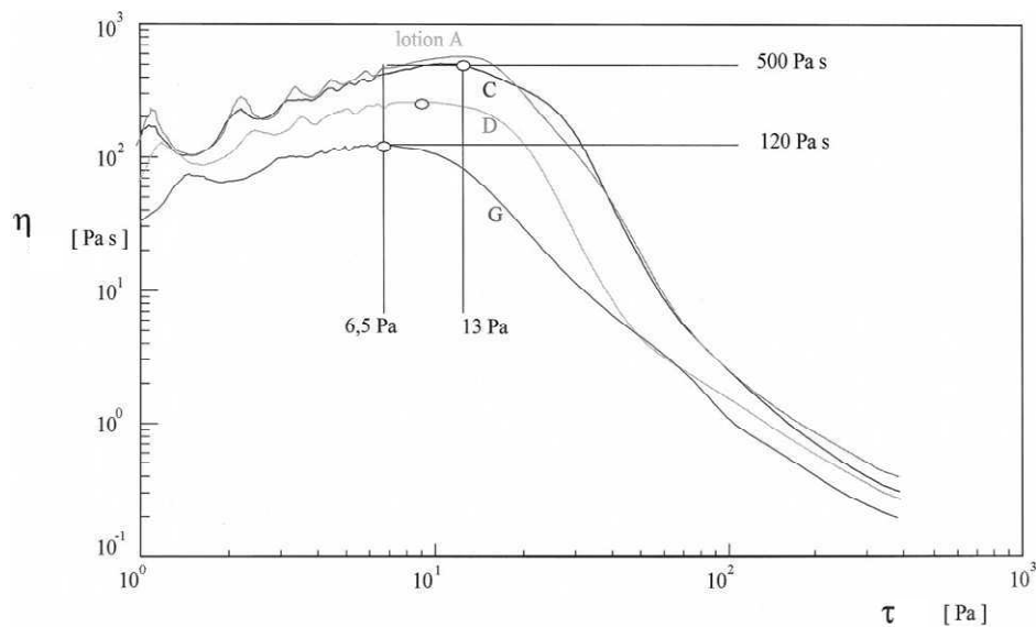
Figure 21. Courbes de viscosité en fonction de la contrainte pour des lotions H/E évaluées sensoriellement comme agréables (C et D) et comme désagréables (A et G) (Brummer & Godersky, 1999)
