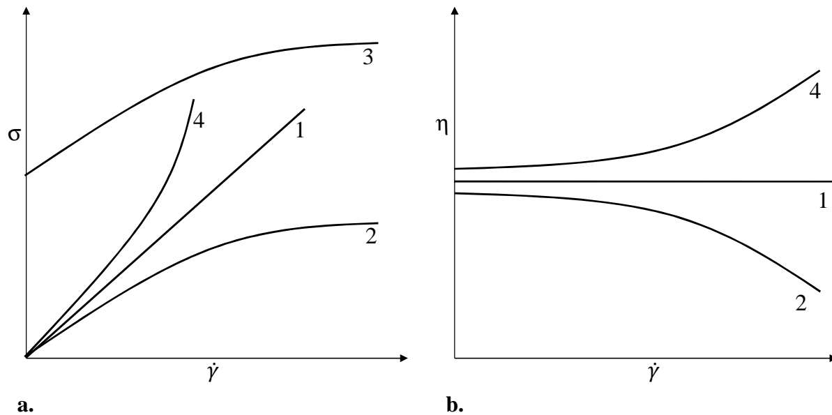
Figure 11. Allures des courbes d'écoulements pour des fluides newtonien (1), rhéofluidifiant (2), viscoplastique (3) et rhéoépaississant (4)
