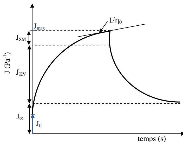
Figure 33. Représentation d'une courbe de fluage-relaxation type présentant les différents paramètres relevés
