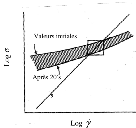
Figure 19. Courbes d'écoulement obtenues pour un fluide newtonien S, et une crème rhéofluidifiante, en mesurant la contrainte \sigma correspondante à chaque gradient de cisaillement \dot{\gamma} , immédiatement et 20 secondes après l'application du gradient (la durée de 20 secondes correspondant au temps moyen d'application sur la peau)
