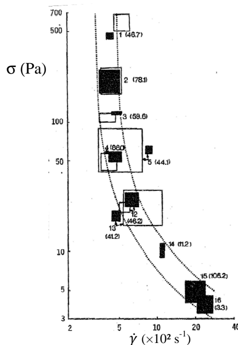
Figure 20. Courbe maîtresse des conditions rhéologiques ayant lieu lors de l'application de crèmes (1-5) ou laits (12-16) sur la peau
