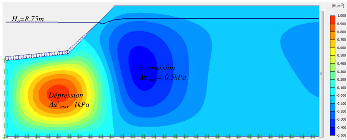
Figure 3.7 : Surpression interstitielle après 1h de consolidation au niveau H_o=8.75m (marée montante)
