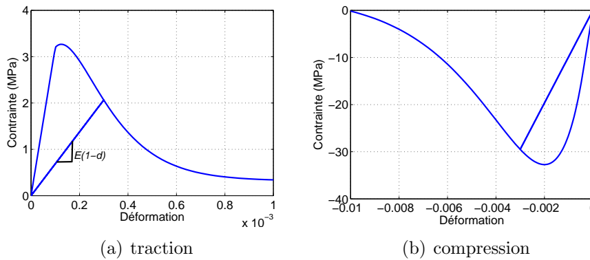
Figure 2.32: Courbes contraintes/déformations pour le modèle Mazars.
