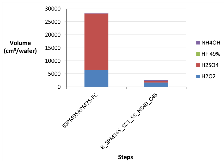
Figure A. 3 Classement des étapes de procédé en fonction de leur consommation de produits chimiques liquides dans l'atelier Wet, pour les deux étapes les plus consommatrices, pour la technologie 45 nm.
