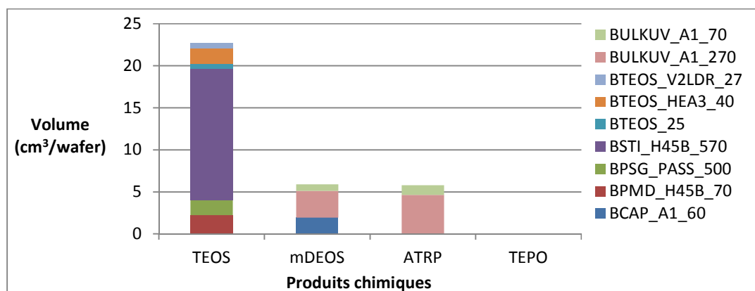
Figure 4. 24 Classement des produits chimiques liquides utilisés dans l'atelier Die1, par étape de la technologie 45 nm.
