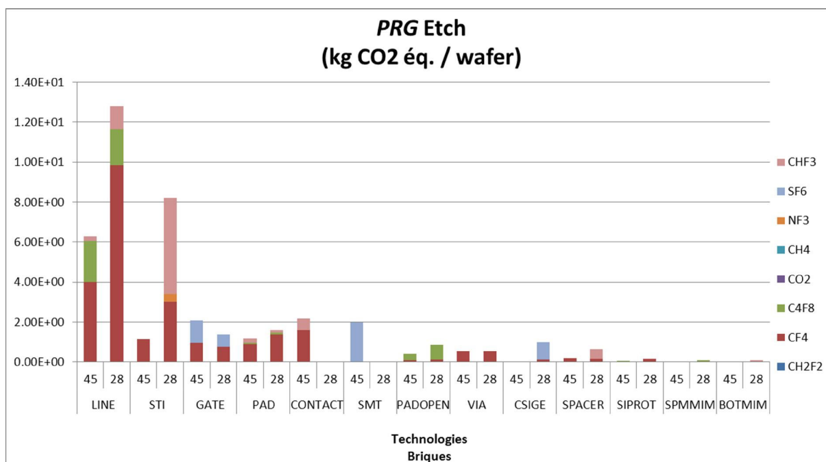
Figure 5. 10 Indicateur PRG détaillé pour un atelier de production (Etch), pour les technologies microélectroniques 45 et 28 nm.
